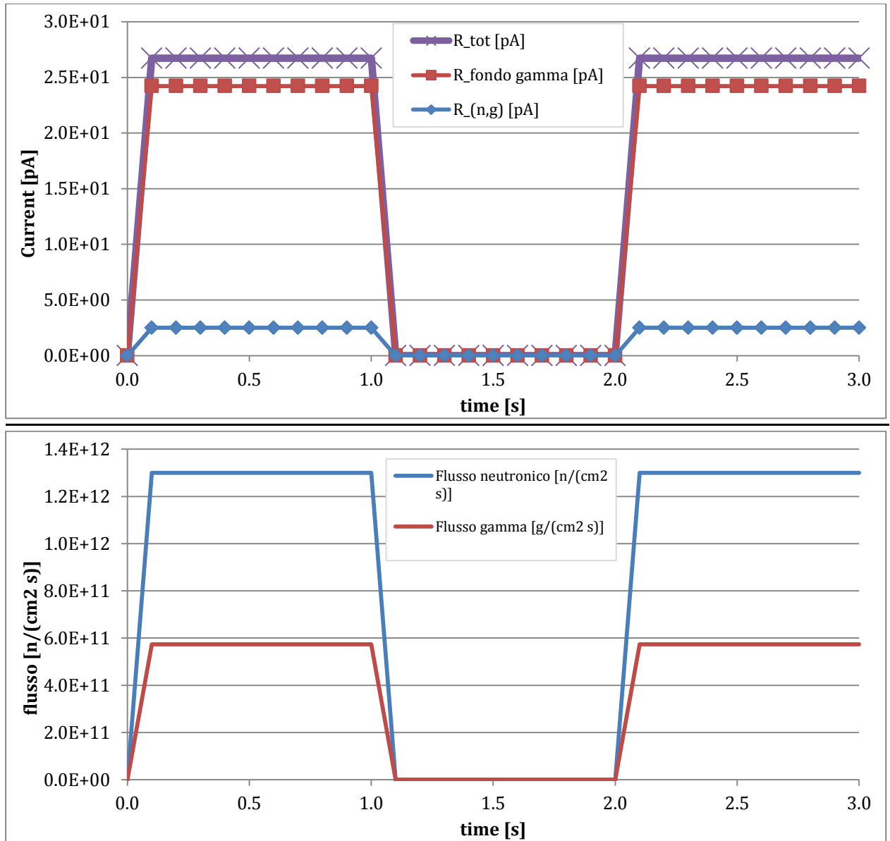
Figura 12 - Risposta dinamica del SPND alimentato con 0 Pt (platino in composizione isotopica naturale) all'interno del canale diametrale di TAPIRO al variare del flusso neutronico (e variazione del conseguente flusso gamma), nel caso di sonda "vergine".
