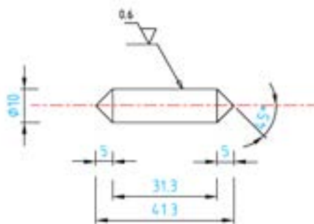
Fig. 7. Geometria provino per test di corrosione
