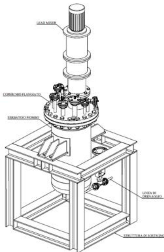
Figura 5: Disegno concettuale (vista isometrica) del vessel dell'impianto a metallo liquido pesante BID1.
