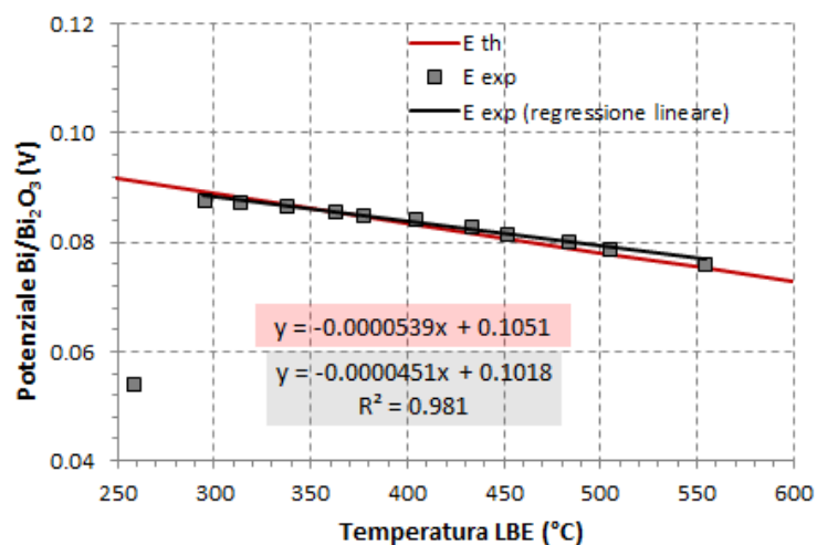
Figura 3: Calibrazione del sensore \text{Bi}/\text{Bi}_2\text{O}_3 in LBE saturo di ossigeno nell'intervallo di temperatura 260-550°C.
