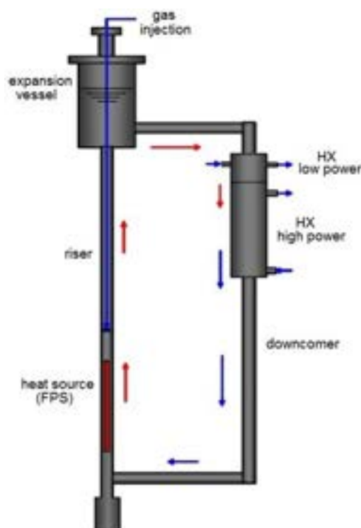
Figura 5: Illustrazione schematica del circuito primario dell'impianto NACIE-UP.
