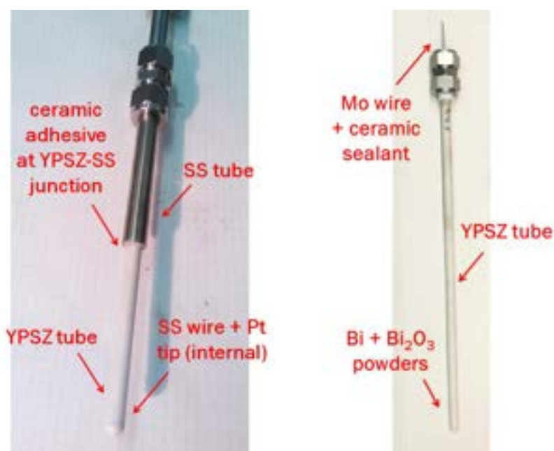
Figura 1: Immagine del sensore di ossigeno Pt-aria (sinistra) e del sensore metallo/metallo-ossido Bi/Bi 2 O 3 (destra) entrambi con elettrolita solido YPSZ.
