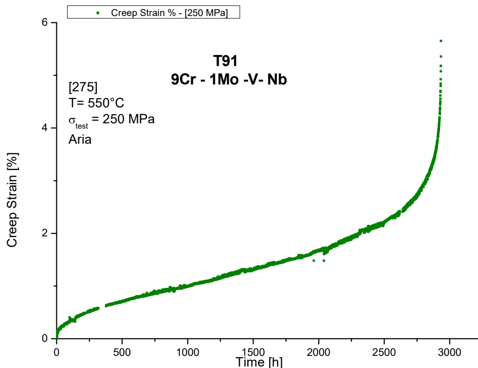
Figura 8: curva di creep relativa al campione [275] PM58412
