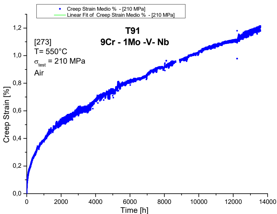
Figura 9: curva di creep relativa al campione [273] PM58212
