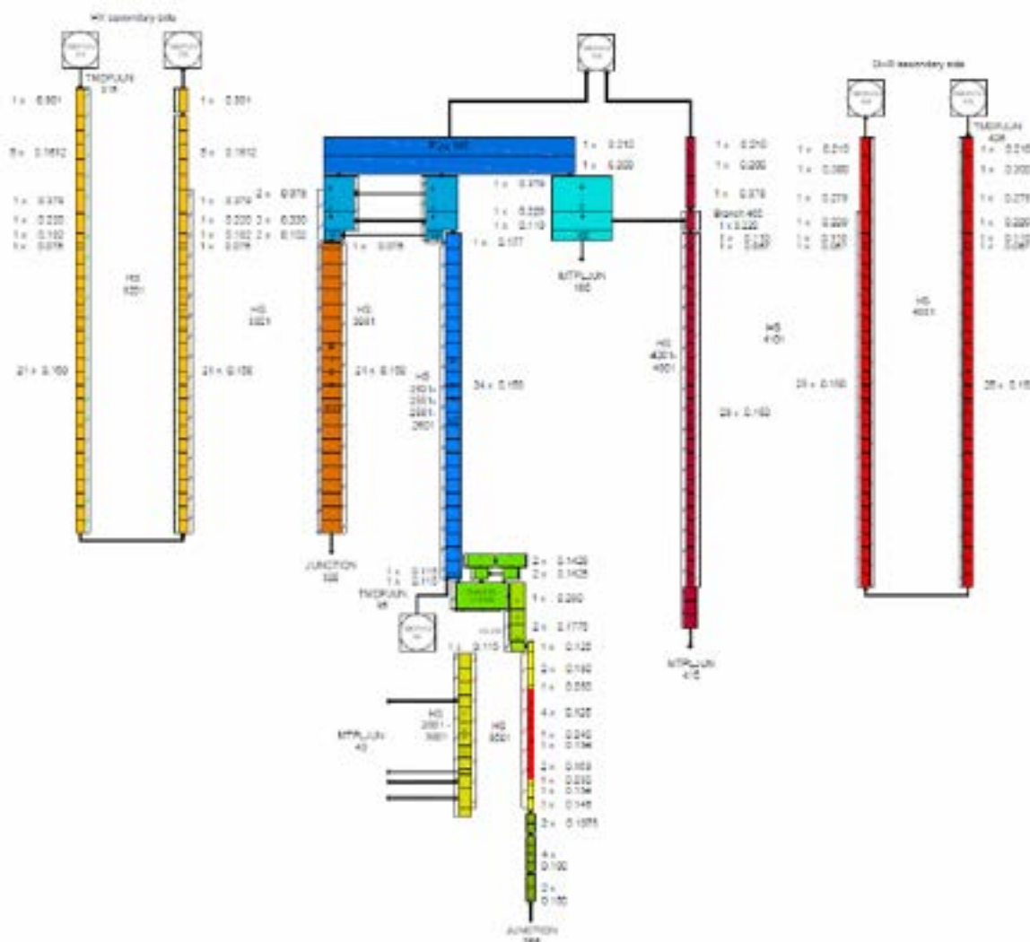
Fig. 2.9 – Nodalizzazione scheme: mono-dimensional model
