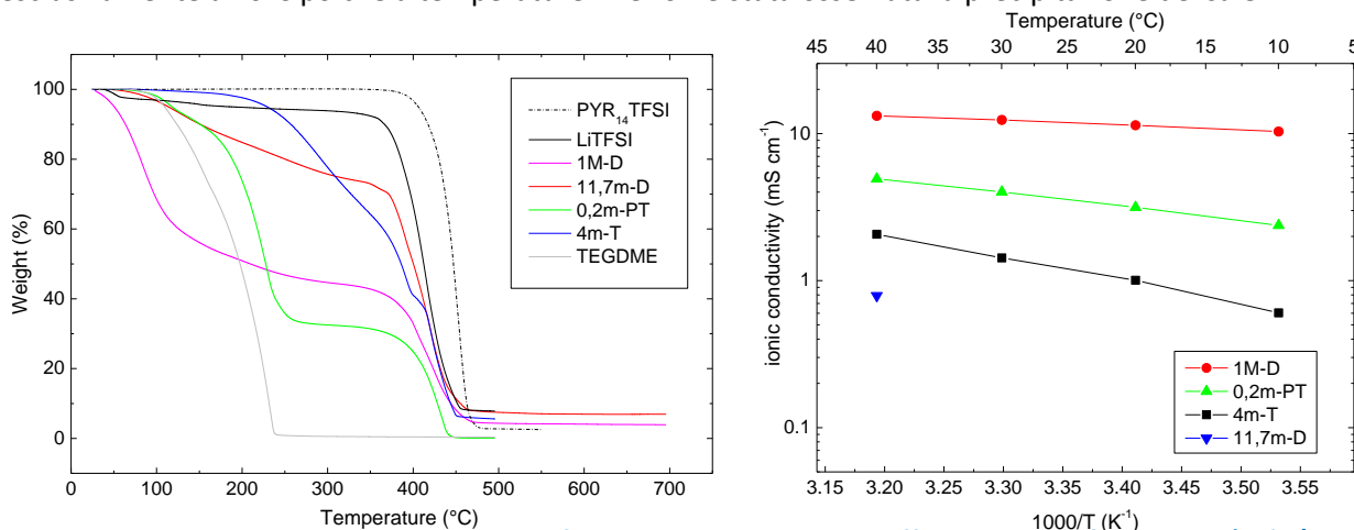
Figura 1. Analisi termogravimetrica di varie formulazioni elettrolitiche effettuate sotto flusso di Ar (10°C/min) e conducibilità ionica di varie formulazioni elettrolitiche a diverse temperature.
