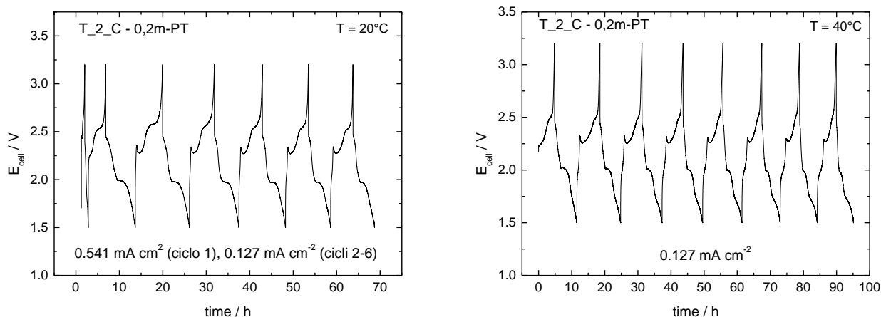
Figura 5. Profili di potenziale dei cicli di carica/scarica dell'elettrodo T_2_C testato in 0,2m-PT a 20°C e a 40°C.
