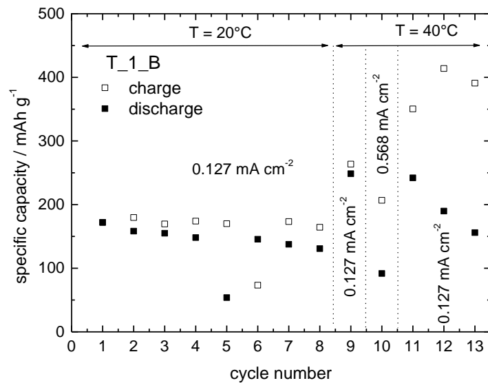
Figura 3. Capacità specifica di carica e scarica vs. numero di cicli a diverse correnti dell'elettrodo T_1_B testato a 20°C e a 40°C in 0,2m-PT.
