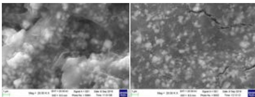
Figura 10. SEM e EDS di T_1_A [TiO 2 (rutilo) + S 75% - carbone 17%] ciclato in 1M-D e di T_1_B ciclato in 0,2m-PT.
