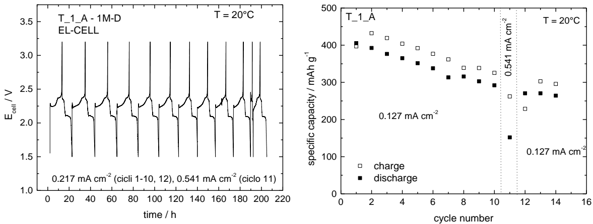
Figura 8. Profili di potenziale dei cicli di carica/scarica e capacità specifica di carica e scarica vs. numero di cicli a diverse correnti a 20°C dell'elettrodo T_1_A testato in 1M-D.
