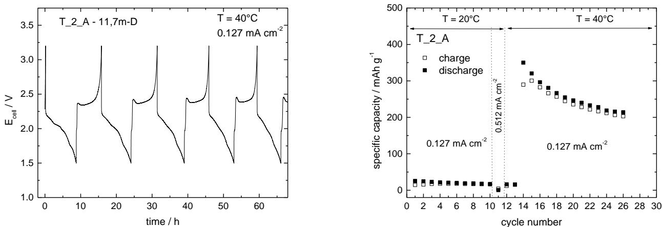
Figura 7. Profili di potenziale dei cicli di carica/scarica dell'elettrodo e capacità specifica di carica e scarica vs. numero di cicli a diverse correnti T_2_A testato in 11,7m-D a 20°C e a 40°C.
