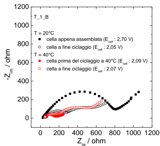
Figura 4. EIS nel range 100 kHz-100 mHz a 20°C e a 40°C dell'elettrodo T_1_B testato in 0,2m-PT.
