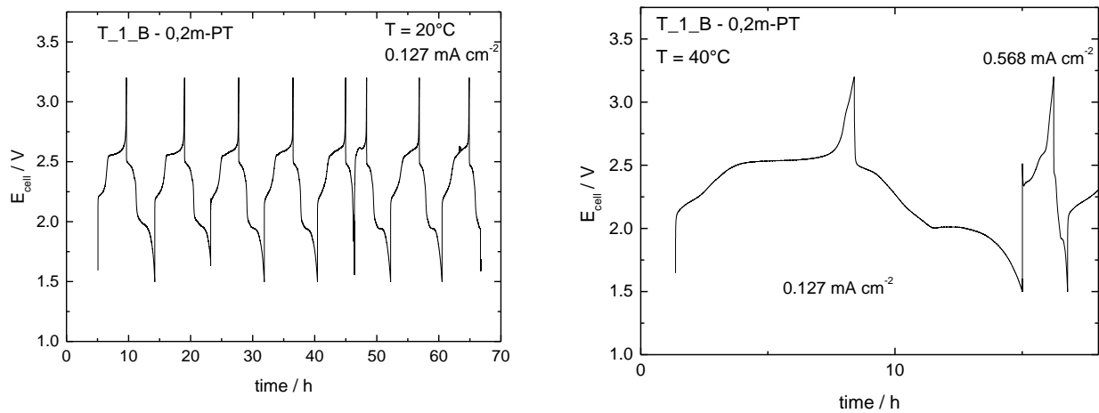
Figura 2. Profili di potenziale dei cicli di carica/scarica a 20°C e a 40°C dell'elettrodo T_1_B testato in 0,2m-PT.
