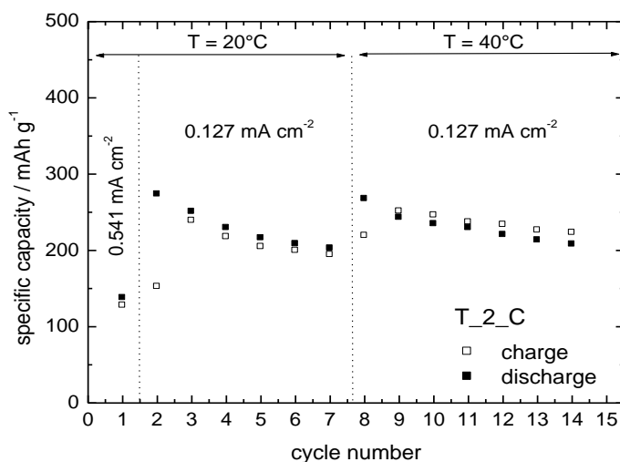
Figura 6. Capacità specifica di carica e scarica vs. numero di cicli a diverse correnti dell'elettrodo T_2_C testato a 20°C e a 40°C in 0,2m-PT.
