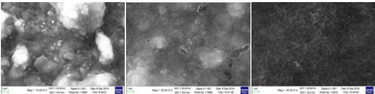
Figura 9. SEM e EDS di G_6_B [ \text{Li}_2\text{S} (Fluka) 68,3% - carbone + pirrolo 23,7%] pristino, ciclato in 1M-D e in 0,2m-PT
