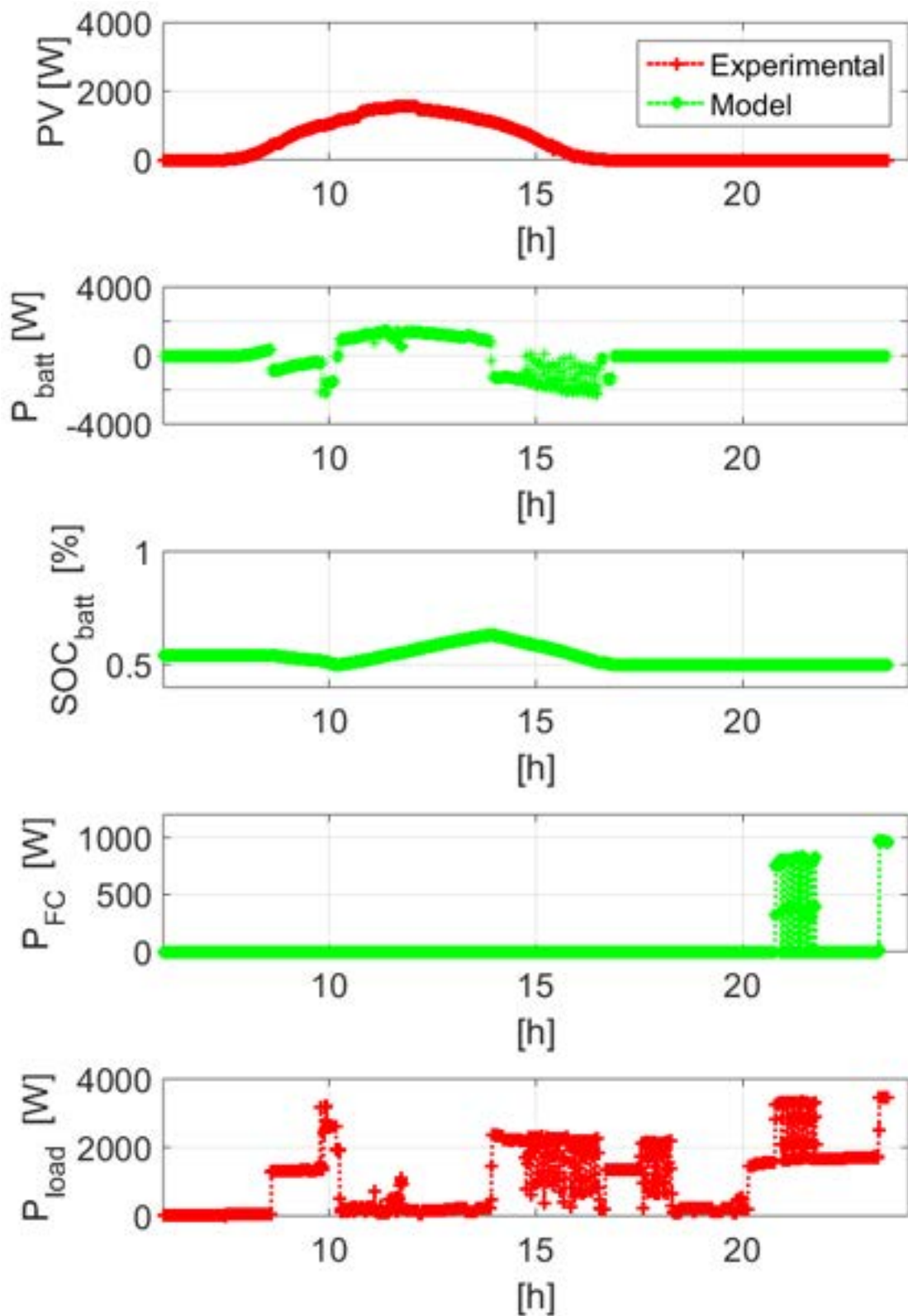
Figura 13. Andamento sperimentale-numerico di (dall'alto) potenza erogata dall'impianto fotovoltaico, potenza scambiata con la batteria, SOC della batteria, potenza erogata dalla Fuel Cell, potenza richiesta al carico. Giornata rappresentativa della stagione invernale dalle 6 alle 24.
