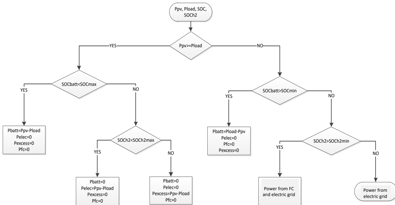
Figura 5. Strategia di controllo per sistemi HRES applicati a Micro-Grid connesse [14].
