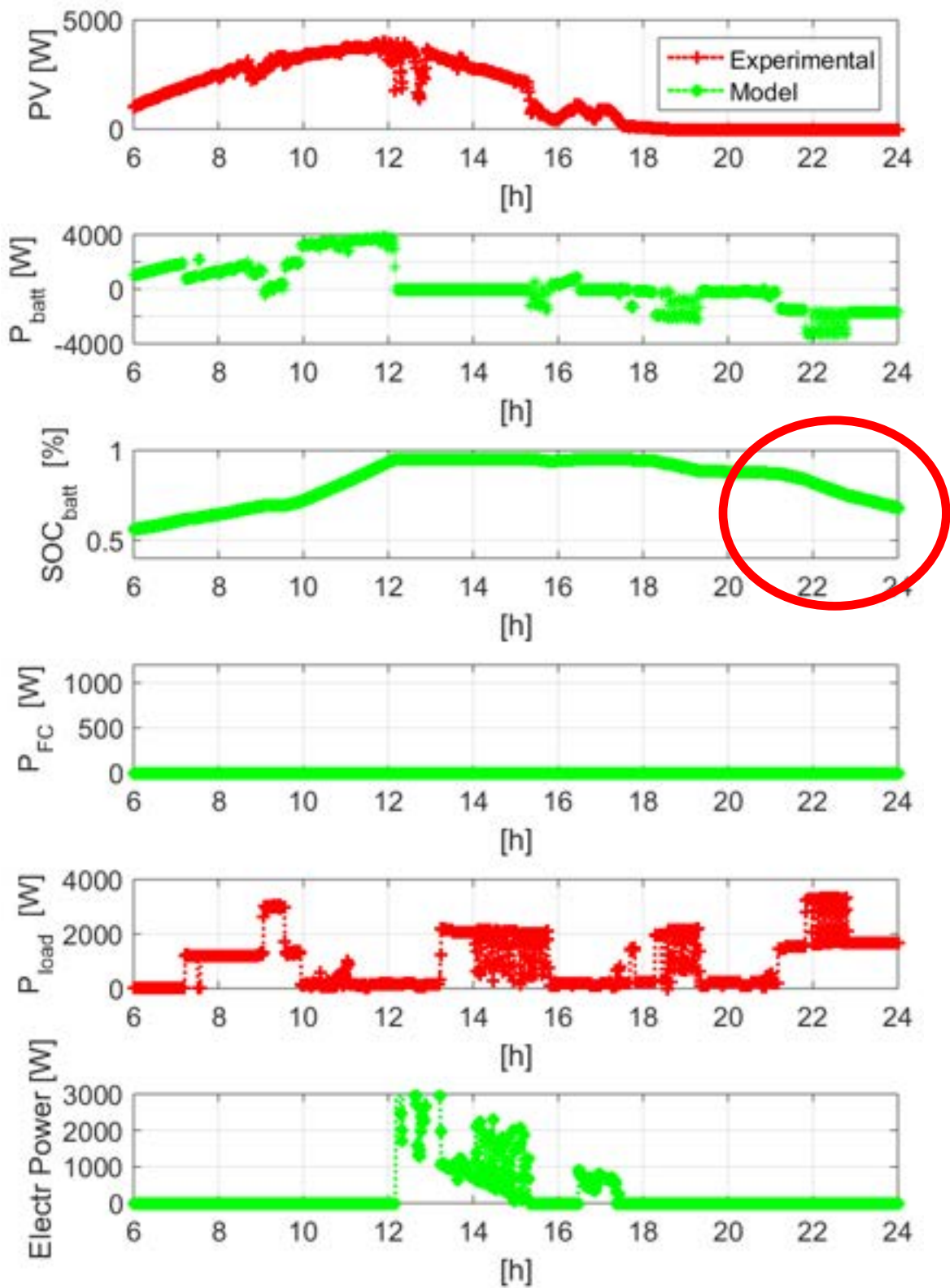
Figura 16. Andamento sperimentale-numeric di (dall'alto) potenza erogata dall'impianto fotovoltaico, potenza scambiata con la batteria, SOC della batteria, potenza erogata dalla Fuel Cell, potenza richiesta al carico, potenza richiesta dall'elettrolizzatore. Giornata rappresentativa della stagione estiva dalle 6 alle 24, capacità della batteria di 640 Ah@48V e impianto fotovoltaico da 5 kWp.
