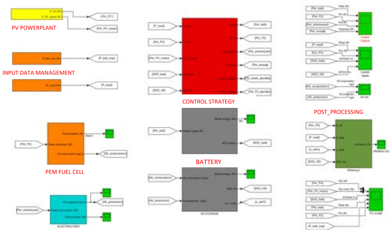
Figura 4. Modello Matlab-Simulink di sistemi HRES.
