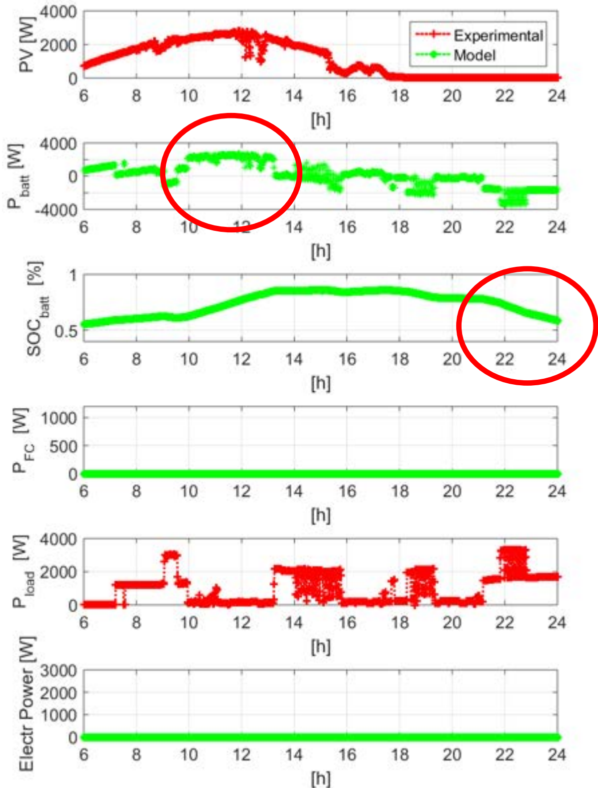
Figura 15. Andamento sperimentale-numeric di (dall'alto) potenza erogata dall'impianto fotovoltaico, potenza scambiata con la batteria, SOC della batteria, potenza erogata dalla Fuel Cell, potenza richiesta al carico, potenza richiesta dall'elettrolizzatore. Giornata rappresentativa della stagione estiva dalle 6 alle 24, capacità della batteria di 640 Ah@48V (capacità nominale dell'esperimento).
