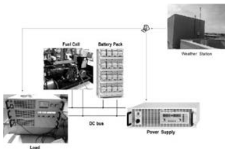
Figura 2. Setup sperimentale implementato nel laboratorio del Dipartimento di Ingegneria Industriale dell'Università di Roma "Tor Vergata [15].
