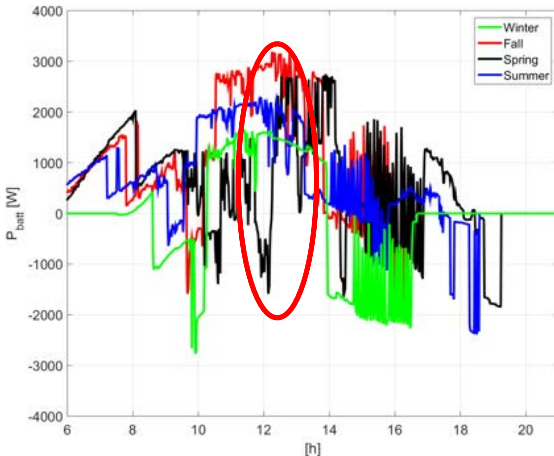
Figura 12. Confronto tra gli andamenti di potenza scambiata con la batteria nelle quattro giornate rappresentative.
