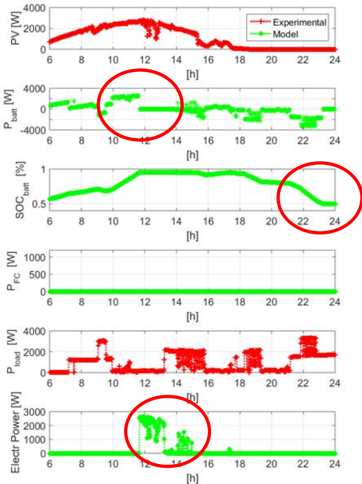
Figura 14. Andamento sperimentale-numerico di (dall'alto) potenza erogata dall'impianto fotovoltaico, potenza scambiata con la batteria, SOC della batteria, potenza erogata dalla Fuel Cell, potenza richiesta al carico, potenza richiesta dall'elettrolizzatore. Giornata rappresentativa della stagione estiva dalle 6 alle 24, capacità della batteria di 320 Ah@48V (1/2 dell'esperimento).
