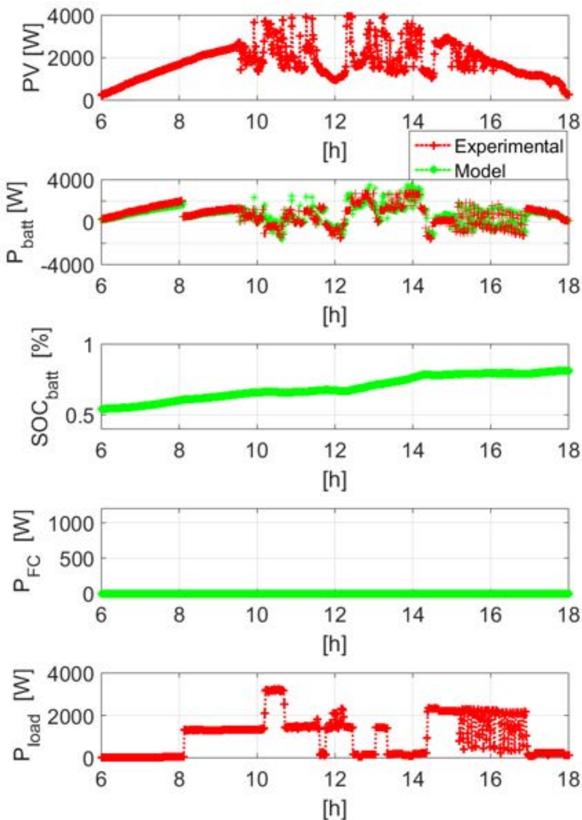
Figura 10. Andamento sperimentale-numerico di (dall'alto) potenza erogata dall'impianto fotovoltaico, potenza scambiata con la batteria, SOC della batteria, potenza erogata dalla Fuel Cell, potenza richiesta al carico. Giornata rappresentativa della stagione primaverile.
