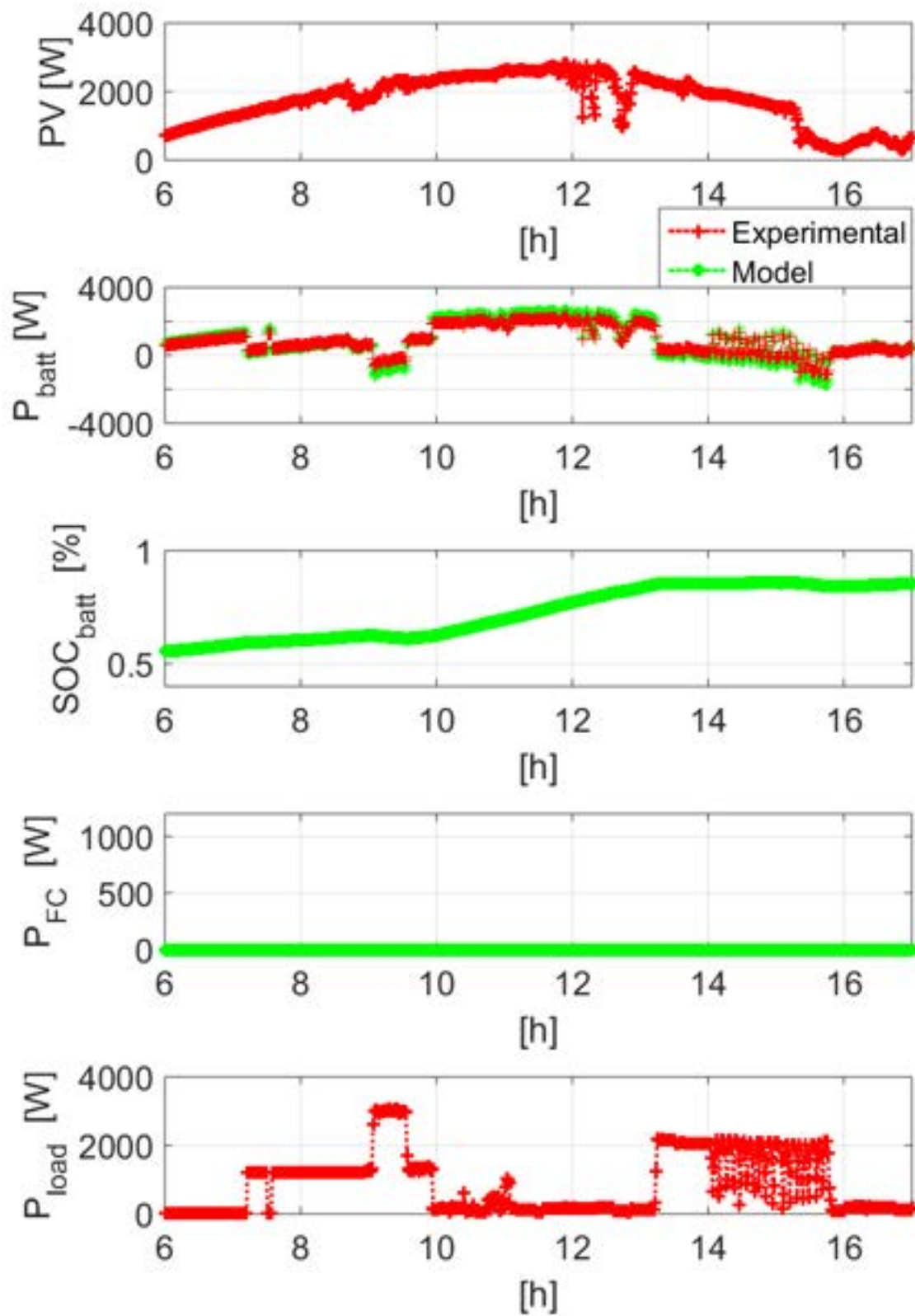
Figura 11. Andamento sperimentale-numeric di (dall'alto) potenza erogata dall'impianto fotovoltaico, potenza scambiata con la batteria, SOC della batteria, potenza erogata dalla Fuel Cell, potenza richiesta al carico. Giornata rappresentativa della stagione estiva
