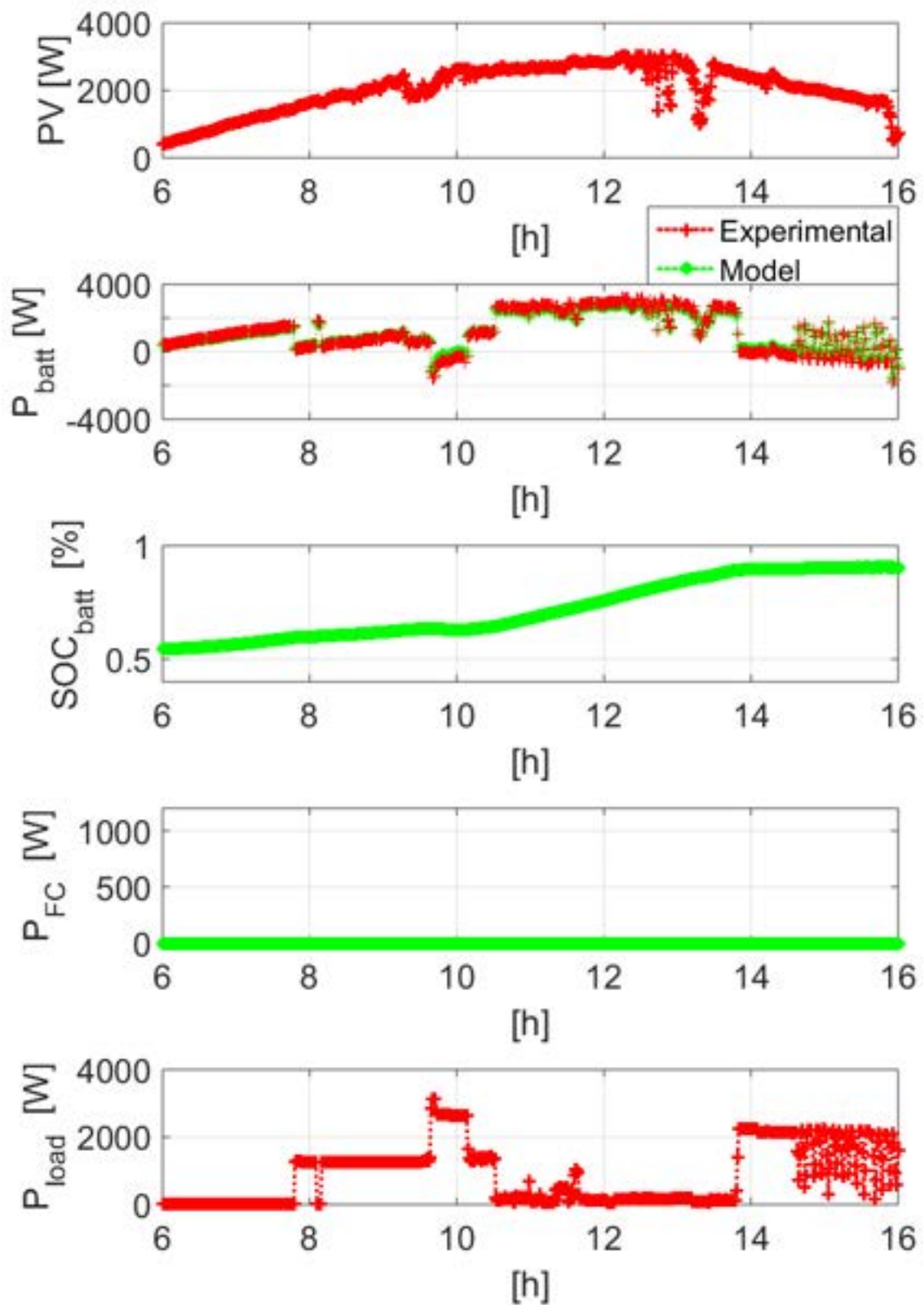
Figura 9. Andamento sperimentale-numerico di (dall'alto) potenza erogata dall'impianto fotovoltaico, potenza scambiata con la batteria, SOC della batteria, potenza erogata dalla Fuel Cell, potenza richiesta al carico. Giornata rappresentativa della stagione autunnale.
