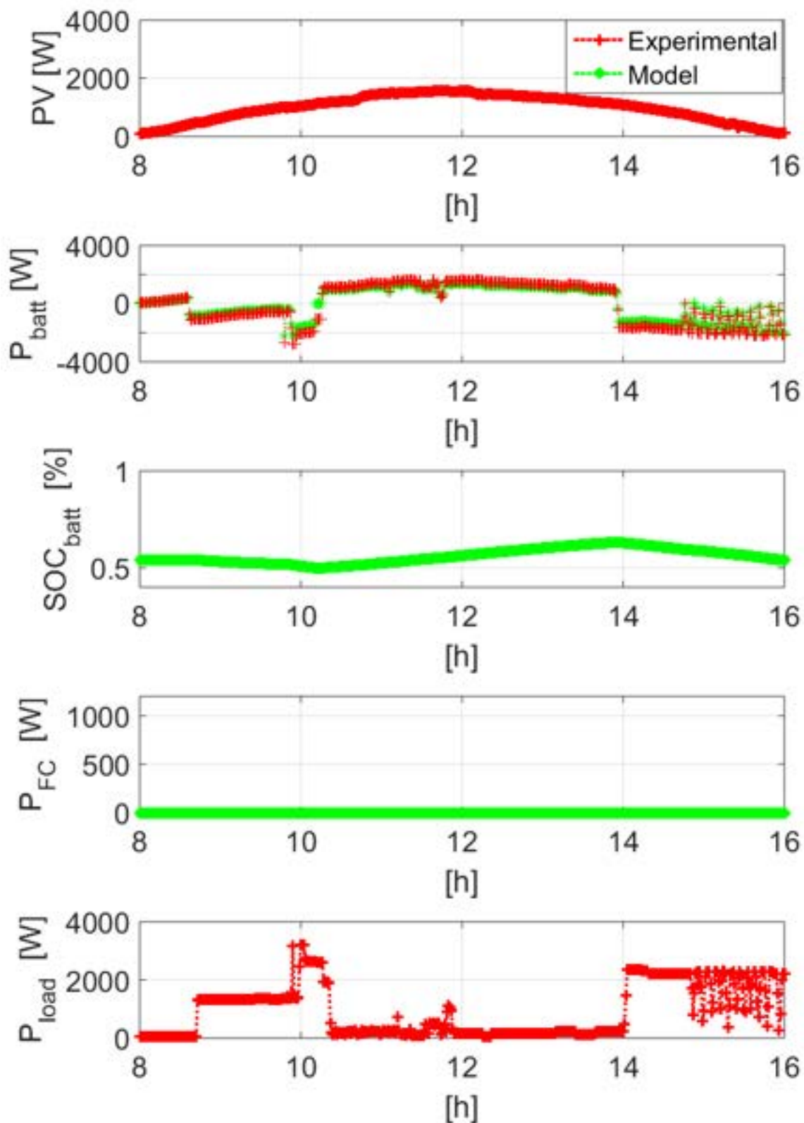
Figura 8. Andamento sperimentale-numerico di (dall'alto) potenza erogata dall'impianto fotovoltaico, potenza scambiata con la batteria, SOC della batteria, potenza erogata dalla Fuel Cell, potenza richiesta al carico. Giornata rappresentativa della stagione invernale.
