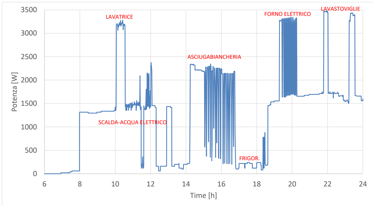
Figura 3. Carico elettrico richiesto in funzione del tempo con indicazioni del contributo dei diversi elettrodomestici [14]
