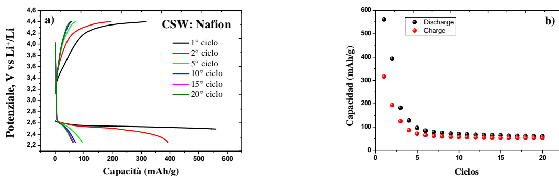
Fig. 14 a) Cella Li/aria scaricata e ricaricata a corrente di 0.1 \text{ mA/cm}^2 , limitando il tempo di scarica a un 20% della scarica totale; catodo Csw e legante Nafion.
