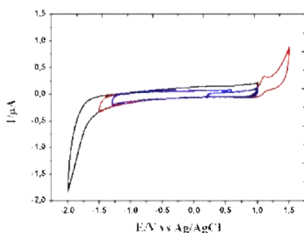
Fig. 1 Profilo voltammetrico dell'elettrodo vetroso di carbonio in 0.1M LiClO 4 TEGDME, soluzione satura di Ar, in differenti intervalli di potenziale, alla velocità di scansione di 10mV/s, 10 cicli.
