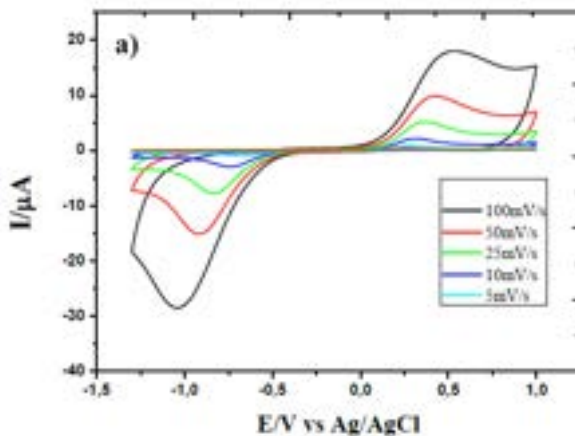
Fig. 7 Profili voltammetrici del glassy carbon in presenza di ossigeno in 0.1 M LiClO 4 in TEGDME a diverse velocità di scansione.
