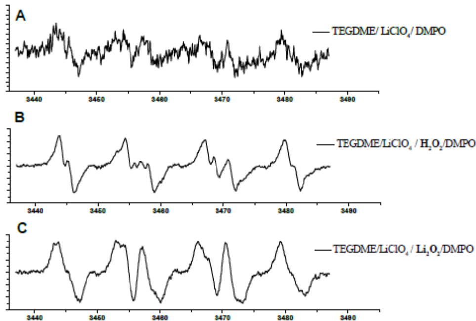
Fig. 5 A) spettro di 0.1M \text{LiClO}_4 in TEGDME. B) 0.1M \text{HClO}_4 in \text{LiClO}_4 in TEGDME/ \text{H}_2\text{O}_2 , C) 0.1 M \text{LiClO}_4 in TEGDME/ \text{Li}_2\text{O}_2 . In tutti gli spettri è stato utilizzato 5,5-dimethyl-1-pyrroline N-oxide (DMPO).
