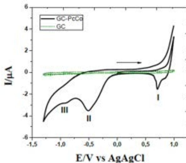
Fig. 9 Profilo voltammetrico di un elettrodo modificato con PcCo in 0.1M LiClO_4 in TEGDME ( N_2 ). Velocità di scansione: 10 mV / s.
