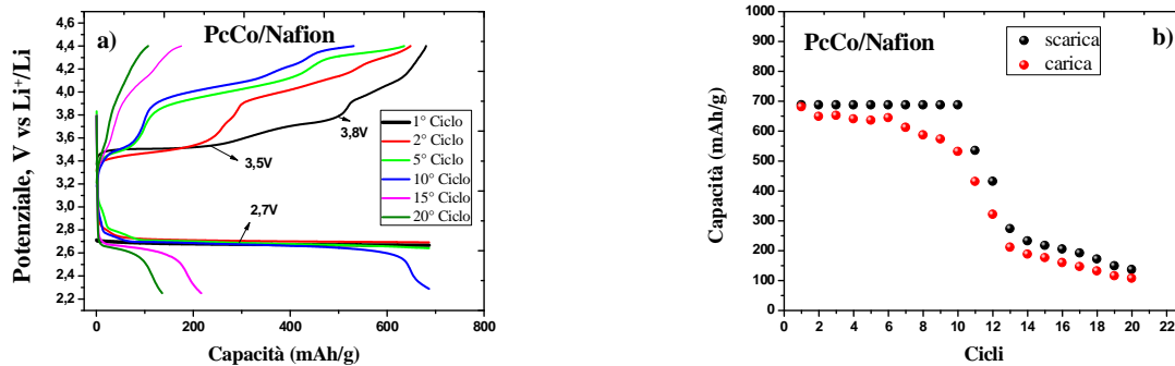
Fig. 15 a) Cella Li/aria scaricata e ricaricata a corrente di 0.1\text{mA}/\text{cm}^2 , limitando il tempo di scarica a un 20% della scarica totale; catodo PcCo e legante Nafion.
