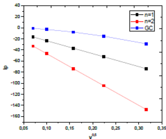
Fig. 8 Curve I_p vs. v^{0.5} , riferite al processo ORR sull elettrodo glassy carbon, curva rossa processo con n=2 , curva nera si riferisce a un processo in cui il trasferimento di elettroni è pari a n=1 , curva blu dati sperimentali ottenuti.
