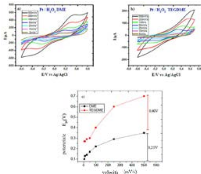
Fig. 3 Profilo ottenuto dalla voltammetria, elettrodo Pt in 9.8 mM H 2 O 2 in DME (a), in TEGDME (b), analisi dei potenziali di ossidazione per H 2 O 2 in funzione della velocità di scansione in DME (nero) e TEGDME (rosso)(c)
