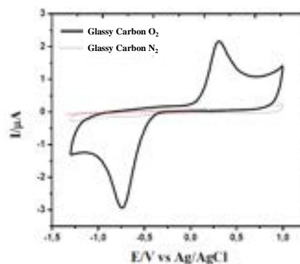
Fig. 6 Profilo voltammetrico del glassy carbon in assenza e in presenza di ossigeno in 0.1 M \text{LiClO}_4 in TEGDME. Velocità di scansione di 10\text{mV/s} .
