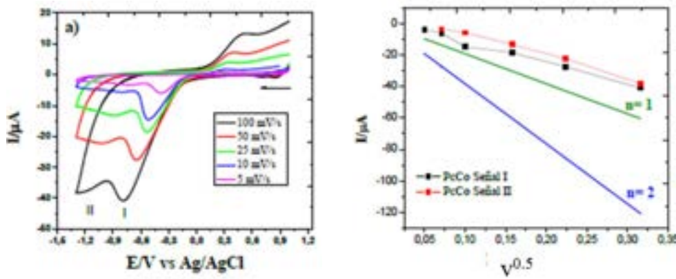
Fig. 11 a) Profilo voltammetrico di un elettrodo modificato con PcCo in presenza di ossigeno in 0.1M LiClO 4 in TEGDME a varie velocità di scansione, b) corrente di picco catodico ( I_p ) verso la radice quadrata della velocità di scansione, per ORR con un elettrodo modificato PcCo.
