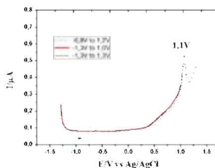
Fig. 2 Profilo ottenuto dalla voltammetria a impulso differenziale, dell'elettrodo vetroso di carbonio in 0.1M LiClO 4 TEGDME, soluzione satura di Ar, in differenti intervalli di potenziale.
