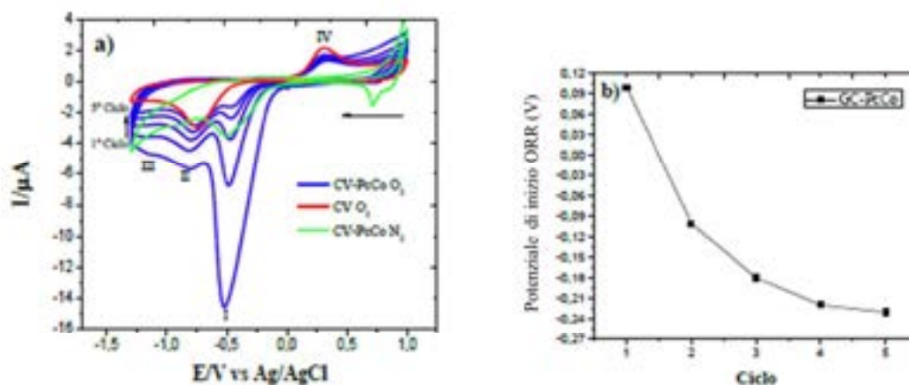
Fig. 10 a) Profilo voltammetrico di un elettrodo modificato con PcCo in assenza di ossigeno (curva verde) e in presenza di ossigeno (curva blu) in 0.1M LiClO 4 in TEGDME. Velocità di scansione: 10 mV / s. b) Spostamento del potenziale di inizio ORR in funzione del numero cicli.
