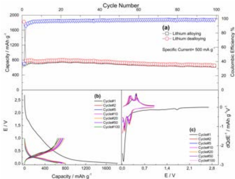
Figura 13. (a) Capacità in carica/scarica dell'elettrodo ( I = 500 \text{ mA g}^{-1} ) di Si@TiO 2 ; (b) profili galvanostatici E vs Q di Si@TiO 2 ; (c) profili differenziali dQ/dE vs E di Si@TiO 2 . Range di potenziale 0.01 < E \text{ (V)} < 1 .
