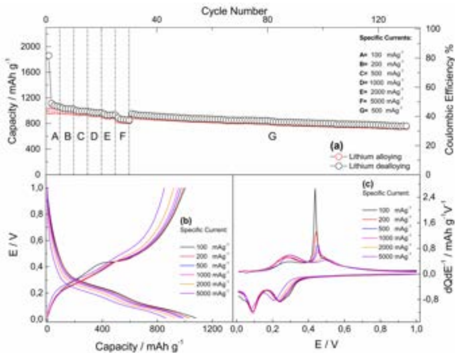
Figura 14. (a) Rate capability di Si@TiO 2 . (A) I = 100 \text{ mA g}^{-1} ; (B) I = 200 \text{ mA g}^{-1} ; (C) I = 500 \text{ mA g}^{-1} ; (D) I = 1000 \text{ mA g}^{-1} ; (E) I = 2000 \text{ mA g}^{-1} ; (F) I = 5000 \text{ mA g}^{-1} ; (G) I = 500 \text{ mA g}^{-1} ; (b) profili galvanostatici E vs Q di Si@TiO 2 ; (c) profili differenziali dQ/dE vs E di Si@TiO 2 . Range di potenziale 0.01 < E \text{ (V)} < 1 .
