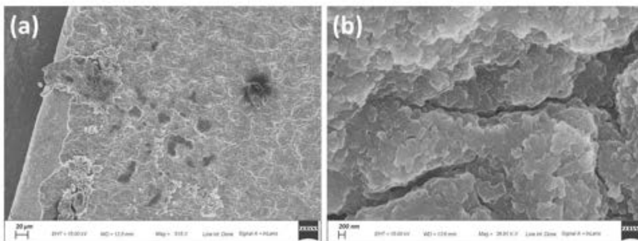
Figura 15. Micrografie SEM post-mortem di Si@TiO 2 a diversi ingrandimenti.
