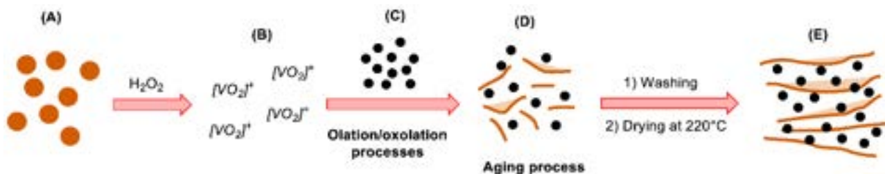
Figura 1. Sintesi del composito Si@V 2 O 5 . (A) o- V 2 O 5 cristallino; (B) ioni [VO 2 ] 2+ ; (C) Nanoparticelle di Silicio; (D) Precursore di Si@ V 2 O 5 ; (E) Composito Si@ V 2 O 5 .
