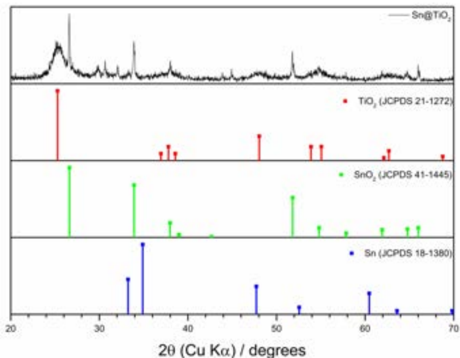
Figura 16. Caratterizzazione XRD di \text{Sn@TiO}_2 .
