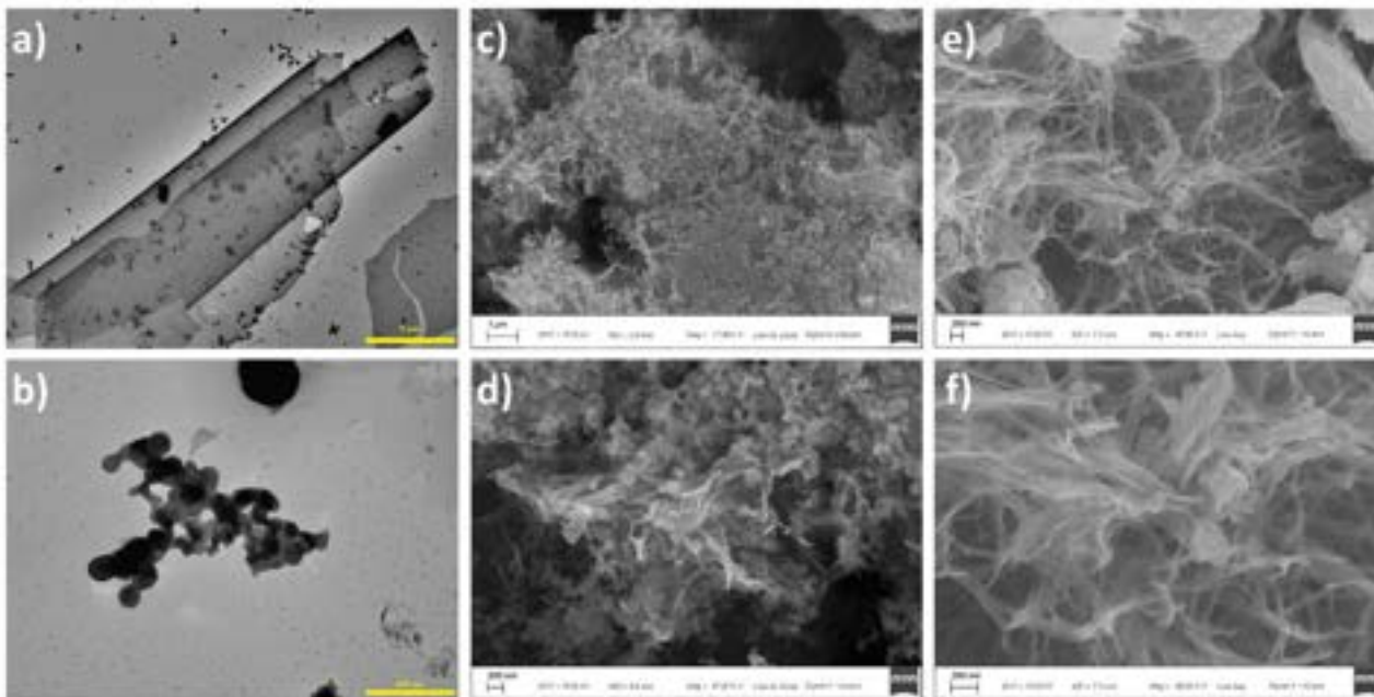
Figure 4. Micrografie TEM (a-b) e SEM (c-d) di Si@V 2 O 5 e SEM di V 2 O 5 (e-f).
