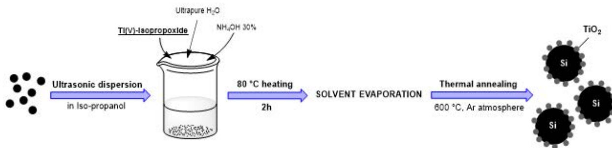
Figura 2. Sintesi dei compositi Si@TiO 2 e Sn@TiO 2 .
