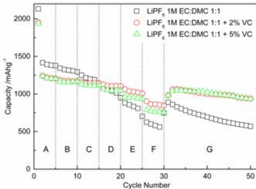
Figura 8. Rate capability di Si@V 2 O 5 utilizzando diverse formulazioni elettrolitiche. (A) I = 100 mA g -1 ; (B) I = 200 mA g -1 ; (C) I = 500 mA g -1 ; (D) I = 1000 mA g -1 ; (E) I = 2000 mA g -1 ; (F) I = 4000 mA g -1 ; (G) I = 500 mA g -1 .
