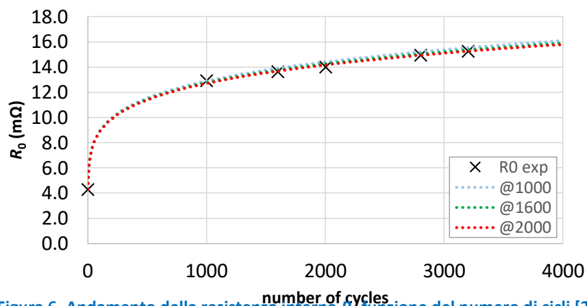
Figura 6. Andamento della resistenza interna R_0 funzione del numero di cicli [2]
