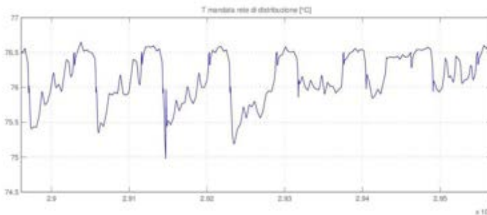
Figura 3-3 - Temperatura di mandata della rete di teleriscaldamento
