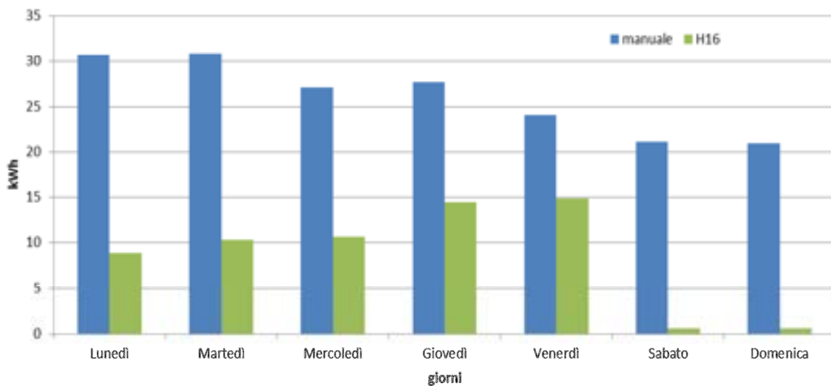
Figura 2.15 confronto settimanale strategie linea cdz (ed. F67)
