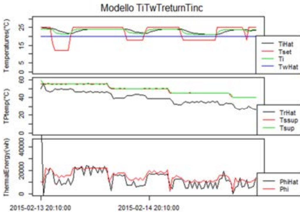
Figura 2.32 risultati modello attuale
