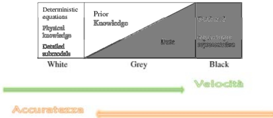
Figura 2.24 : combinazione white e black-box
