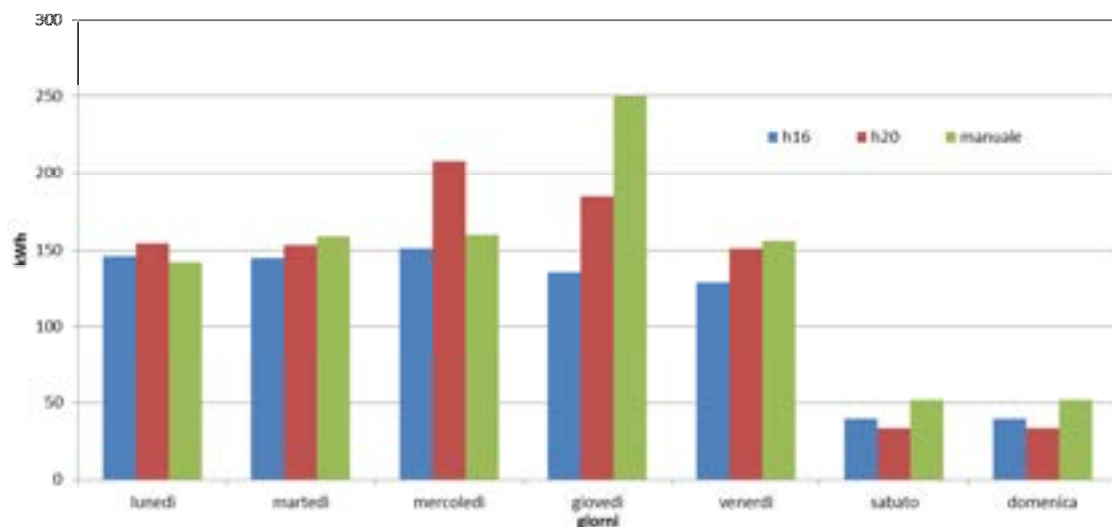
Figura 2.3 confronto settimanale totale strategie linea luci
