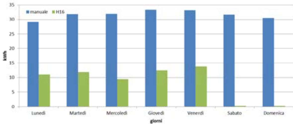
Figura 2.18 confronto settimanale strategie linea cdz (ed. F70)
