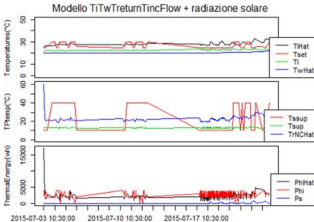
Figura 2.55 TiTwTreturnTincFlow con la radiazione solare
