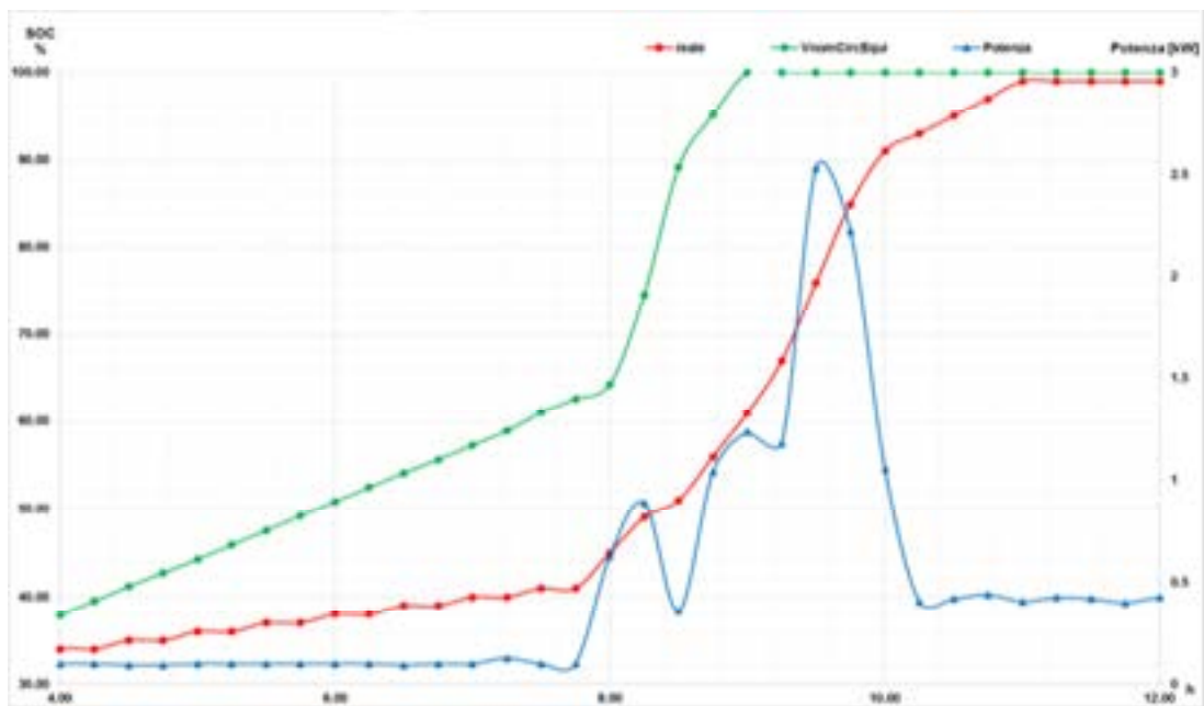
Figura 2.63 Particolare della fase di carica dello storage elettrico (simulato vs. reale)
