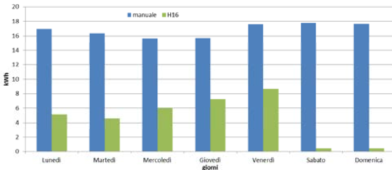
Figura 2.20 confronto settimanale strategie linea cdz (ed. F72)
