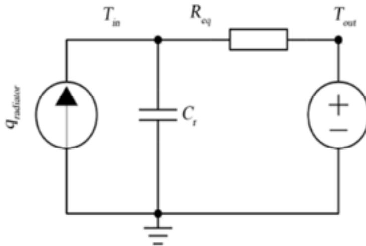
Figura 2.27 schema circuitale equivalente edificio 3.7
