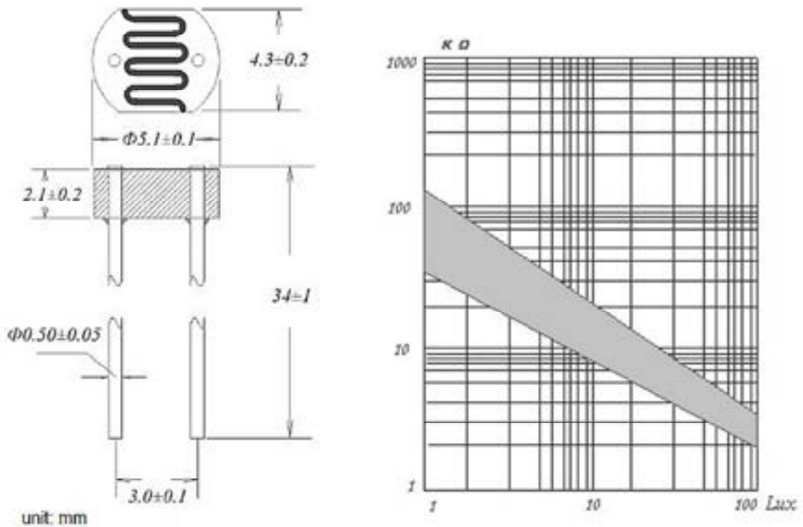
Figura 3.8 – Caratteristiche tecniche del sensore di luminosità
