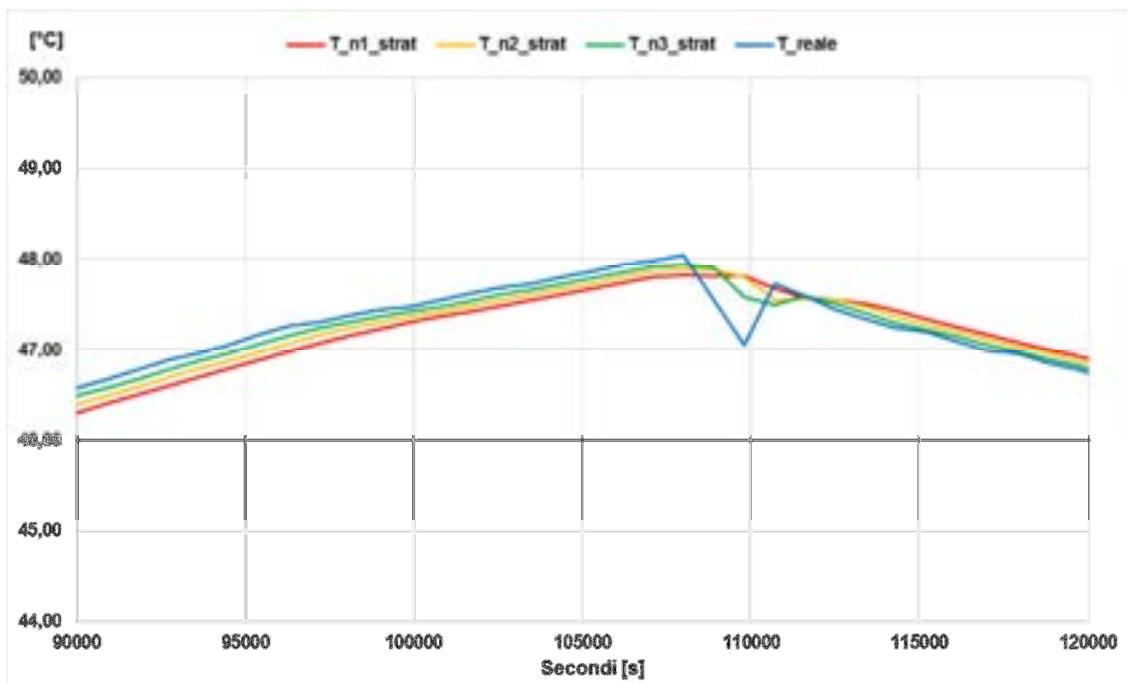
Figura 2.60. Particolare della variazione di temperatura T tra i nodi
