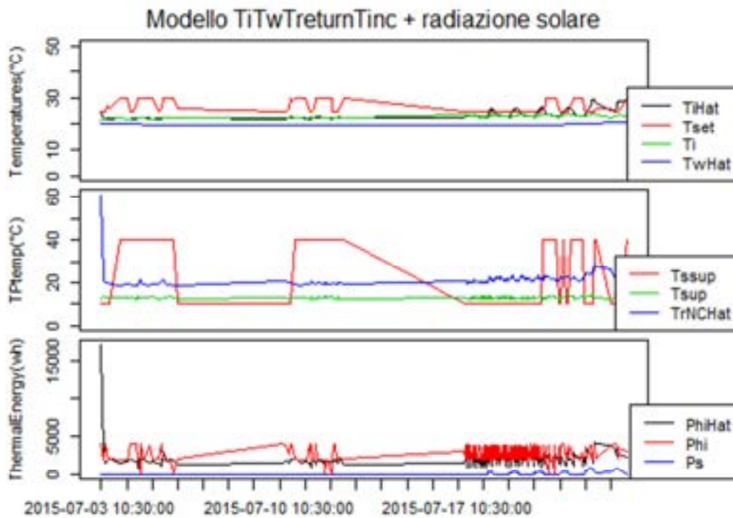
Figura 2.50 modello TiTwTreturnTinc più radiazione solare
