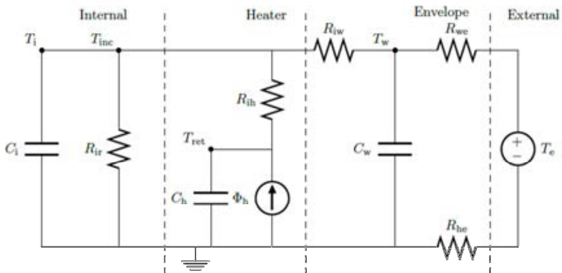
Figura 2.30 schema circuitale TiTwTreturnTinc
