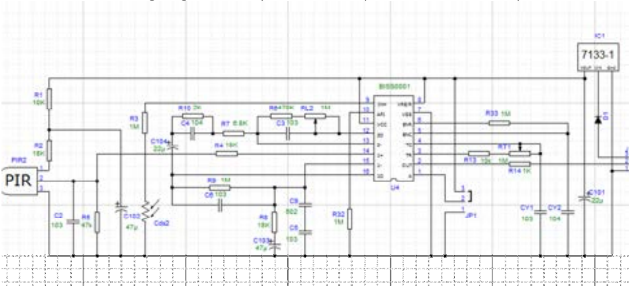
Figura 3.11 Schema elettrico e Caratteristiche del sensore P.I.R.
