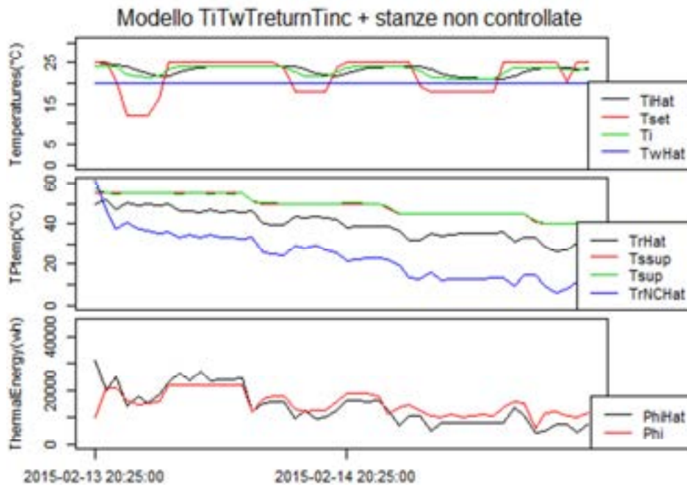
Figura 2.35 risultati con l'aggiunta delle stanze non controllate e modifica del periodo di campionamento
