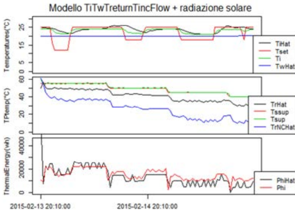
Figura 2.44 con radiazione solare
