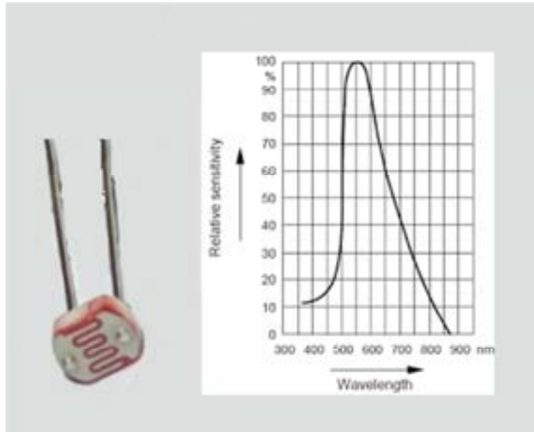
Figura 3.7 - Sensore di luminosità a fotoresistenza
