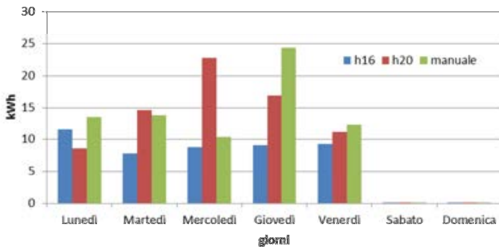
Figura 2.9 confronto settimanale strategie ed.F71 linea luci
