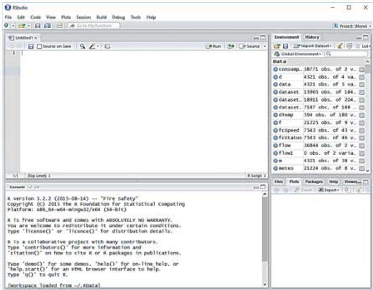
Figura 2.25 schermata Rstudio
