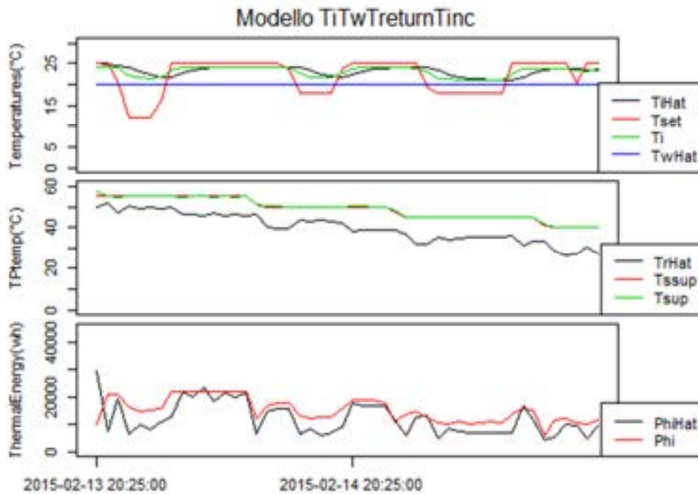
Figura 2.33 risultati modello attuale ( T_s = 3600 )
