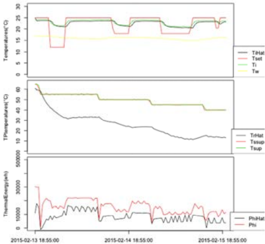
Figura 2.41 circuito TiTwTreturnTincFlow vecchio
