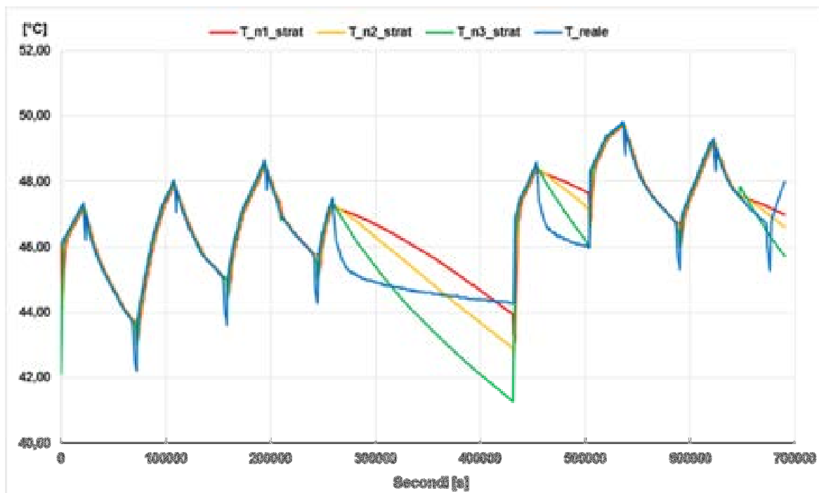
Figura 2.59. Confronto T reale – T modello stratificato a 3 nodi
