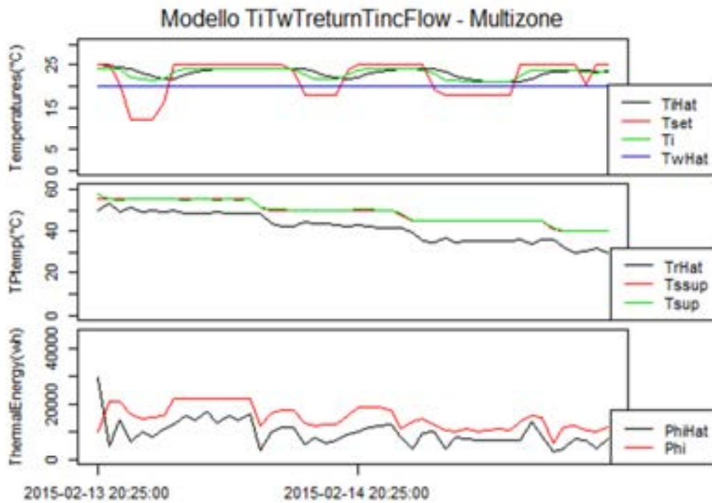
Figura 2.40 circuito TiTwTreturnTincFlow + cambiamento T_s
