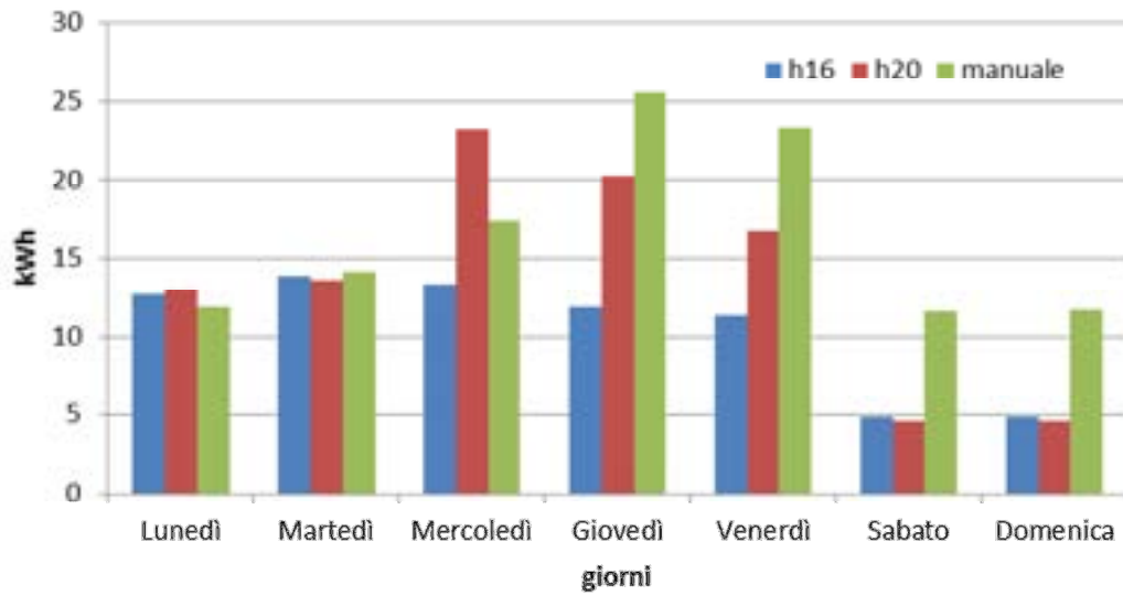
Figura 2.7 confronto settimanale strategie ed.F69 linea luci
