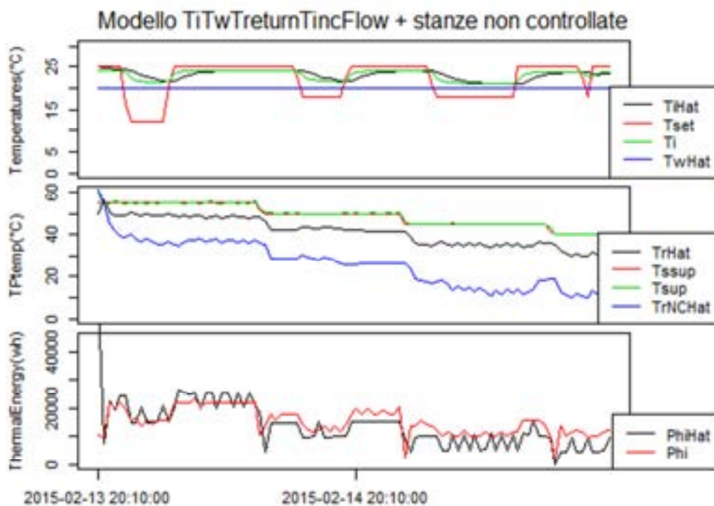
Figura 2.42 con stanze non controllate nuovo
