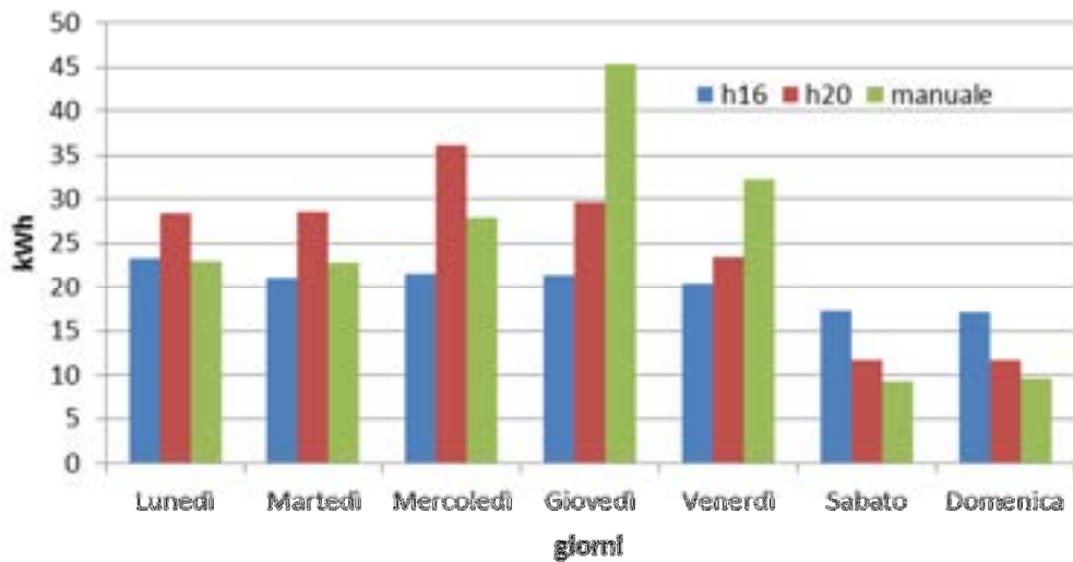
Figura 2.5 confronto settimanale strategie ed.F67 linea luci
