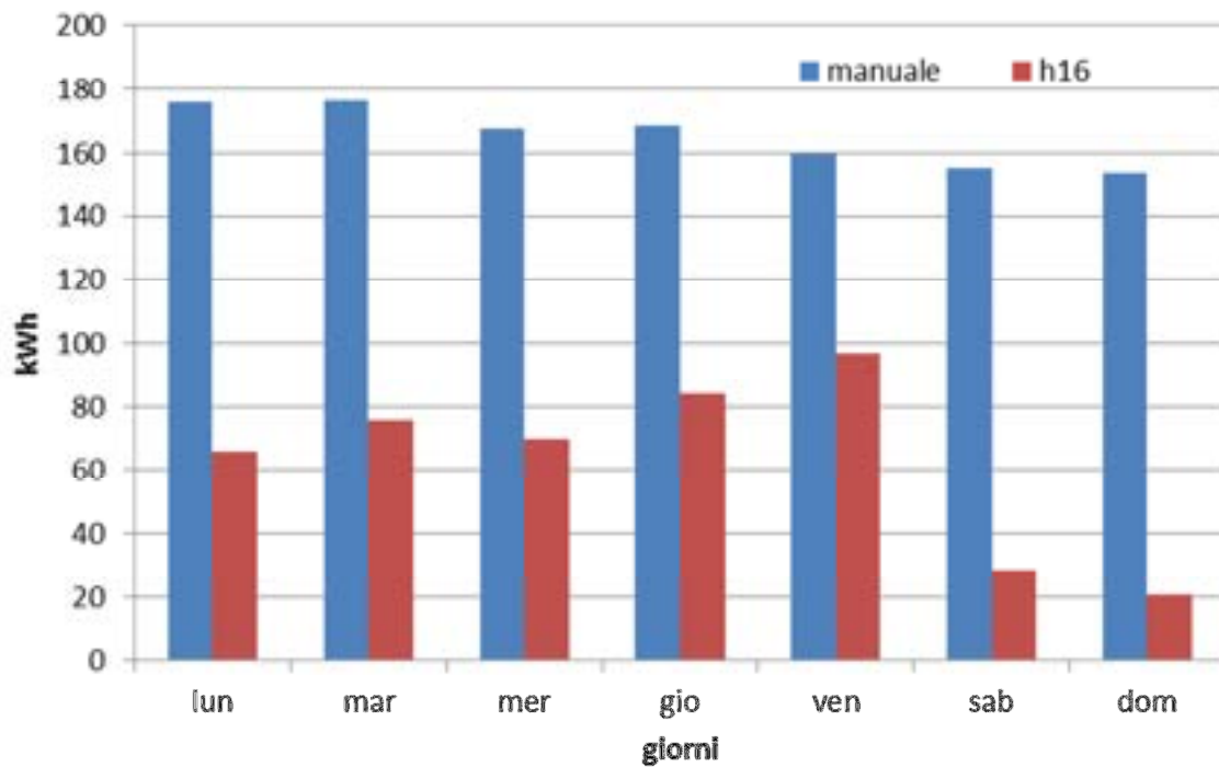
Figura 2.13 confronto settimanale totale strategie linea cdz
