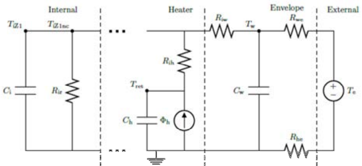
Figura 2.52 circuito TiTwTreturnTincFlow
