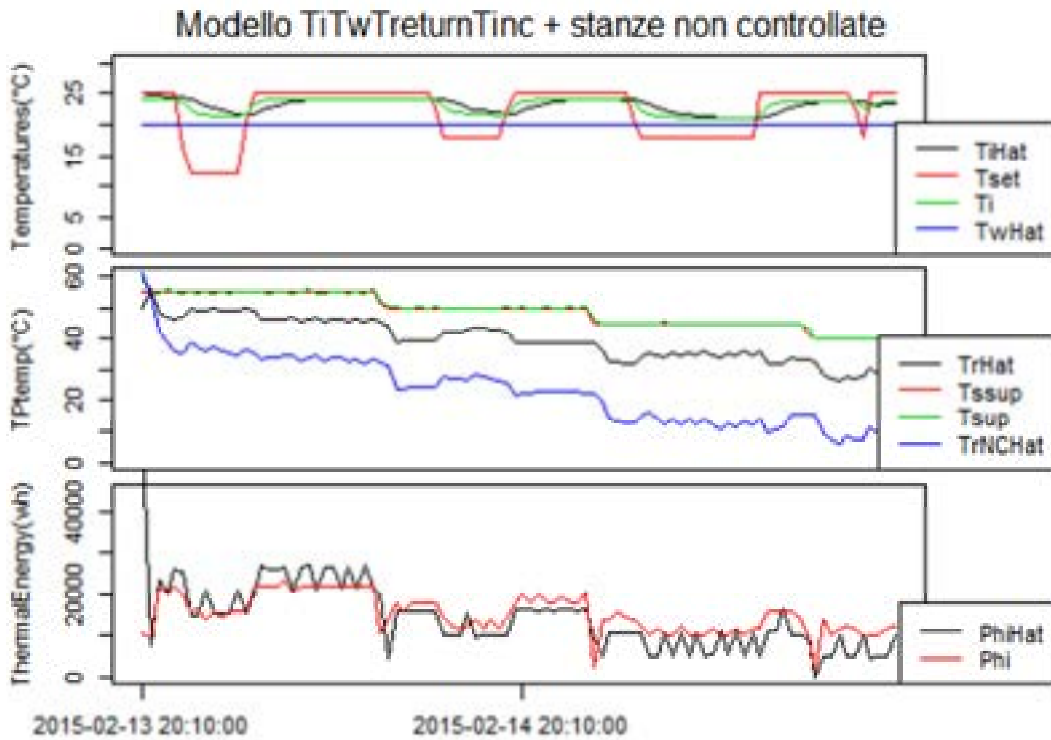
Figura 2.34 risultati con l'aggiunta delle stanze non controllate
