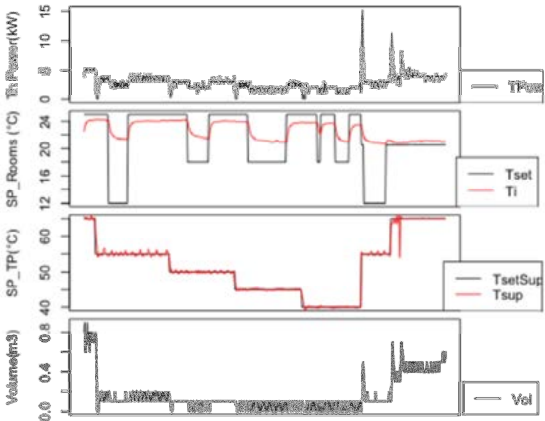
Figura 2.29 risultati ottenuti con radiatore chiuso
