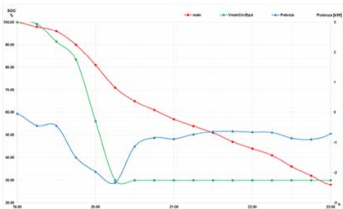
Figura 2.64. Particolare della fase di scarica dello storage elettrico (simulato vs. reale)
