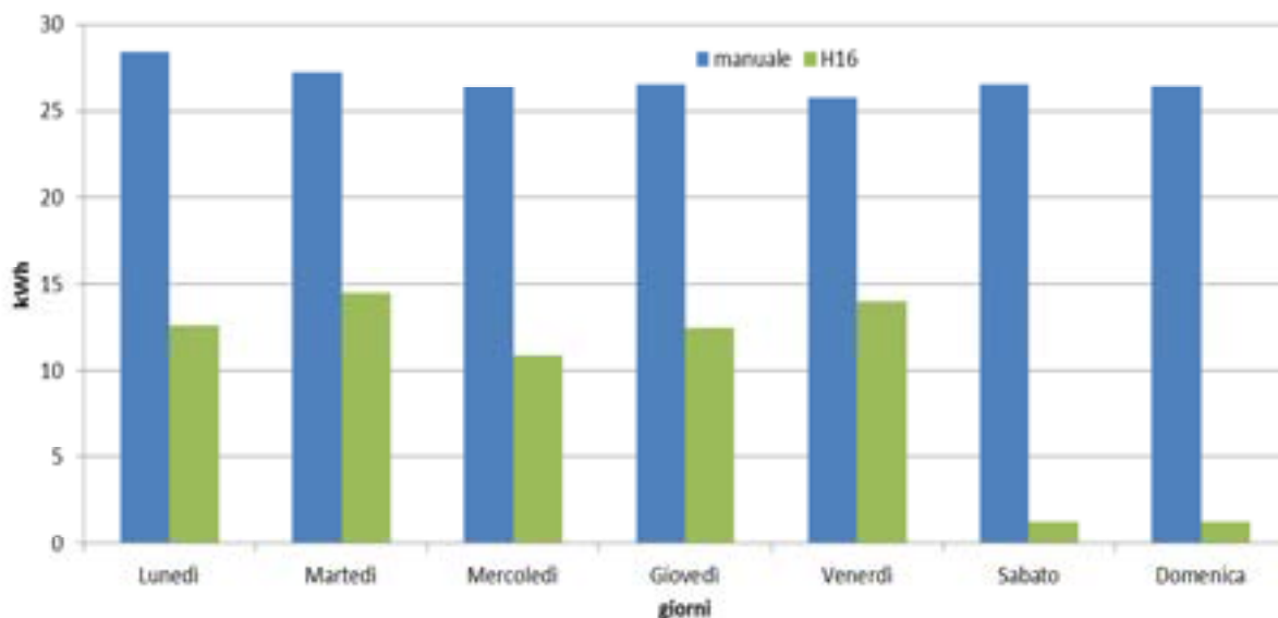
Figura 2.14 confronto settimanale strategie linea cdz (ed. F66)
