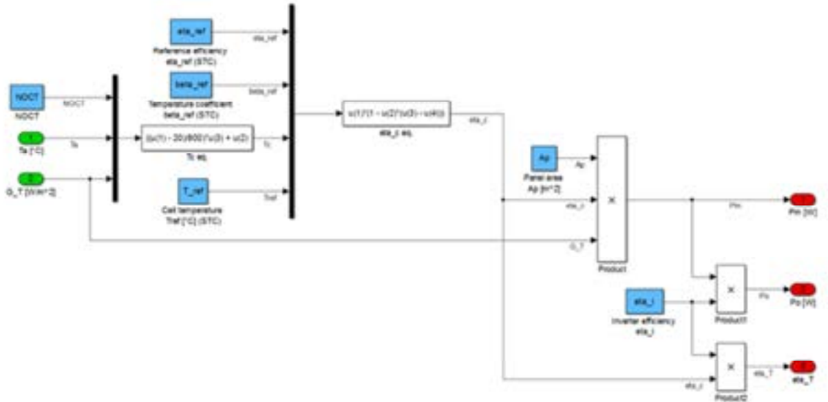
Figura 2.57. Modello Simulink dei pannelli fotovoltaici e dell'inverter.
