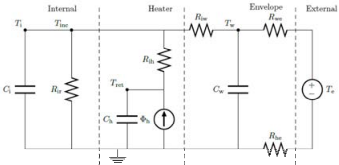
Figura 2.47 circuito T_i T_w T_{ret} T_{inc}
