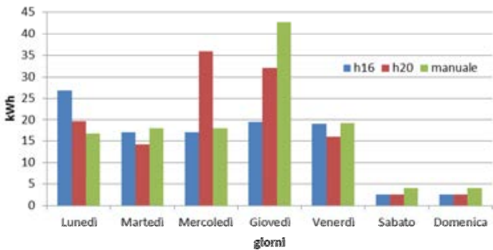
Figura 2.6 confronto settimanale strategie ed.F68 linea luci
