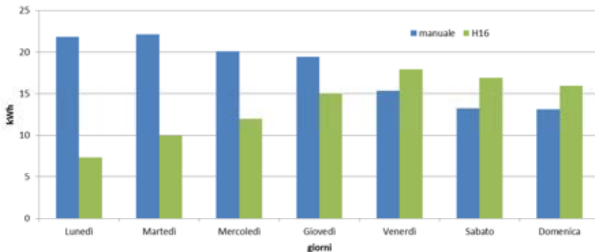
Figura 2.16 confronto settimanale strategie linea cdz (ed. F68)
