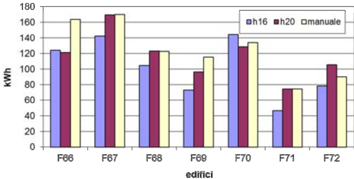
Figura 2.2 riepilogo strategie linea luci
