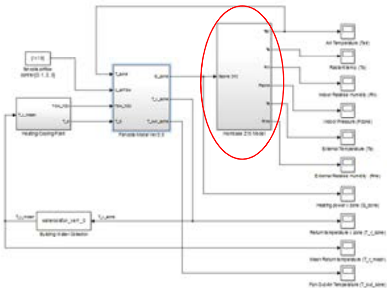
Figura 2.68. Simulatore F40 con Hambase
