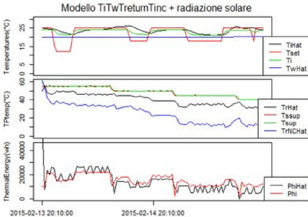
Figura 2.37 risultati con l'aggiunta della radiazione solare
