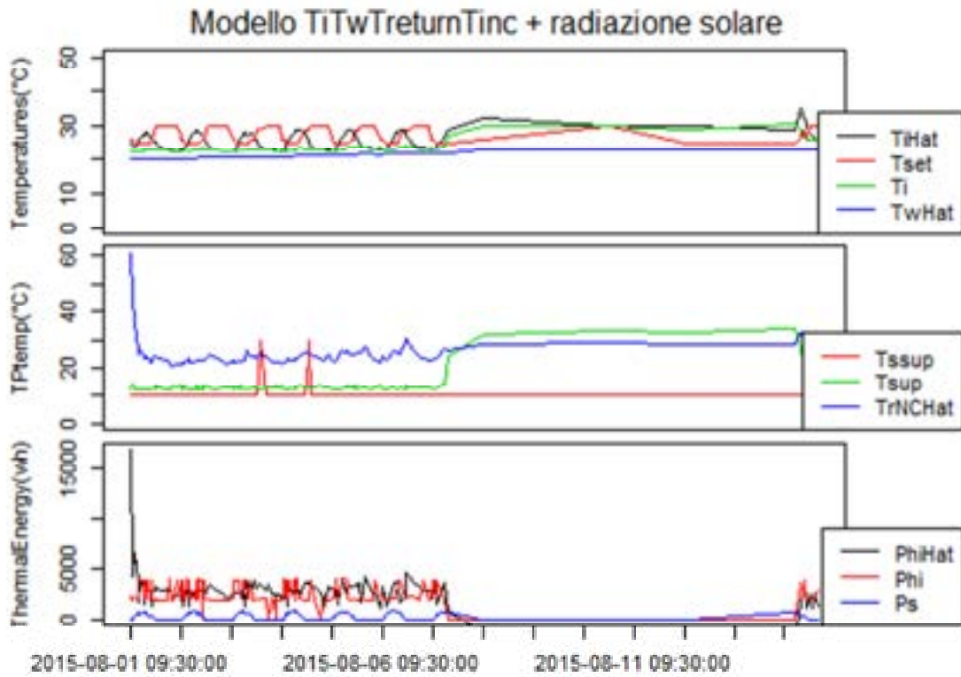
Figura 2.51 modello TiTwTreturnTinc più radiazione solare
