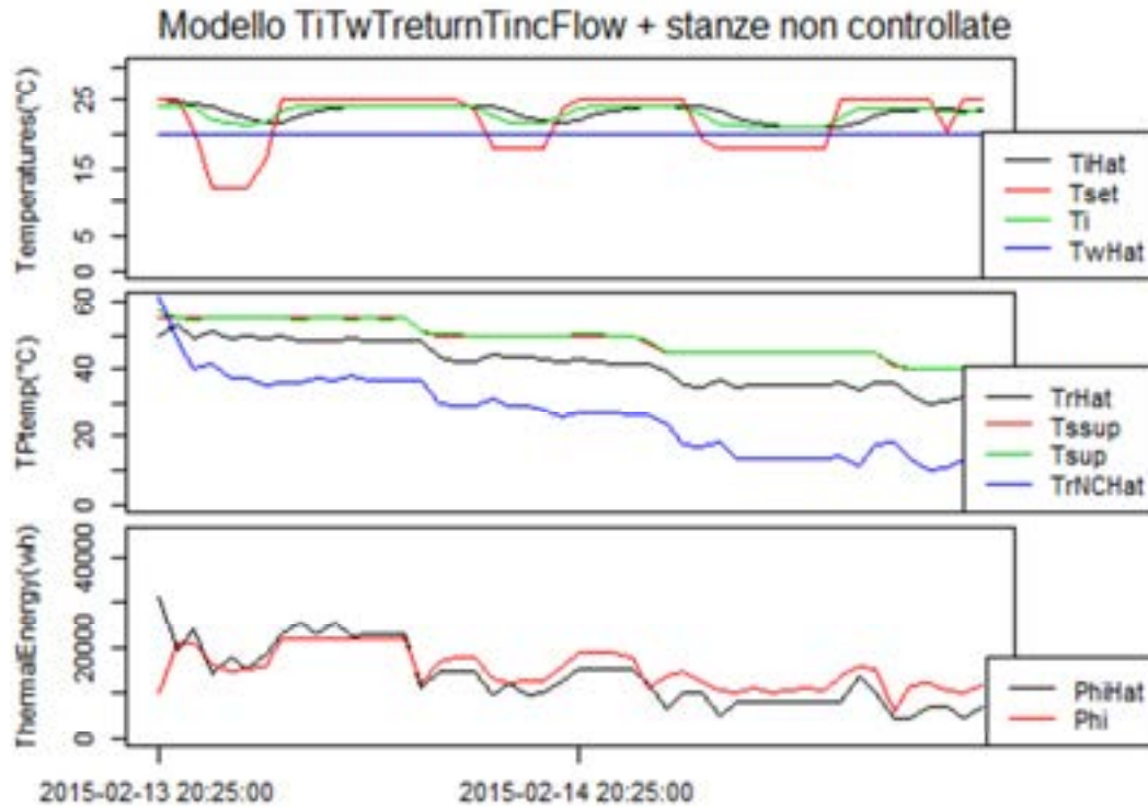
Figura 2.43 con stanze non controllate nuovo + cambio periodo
