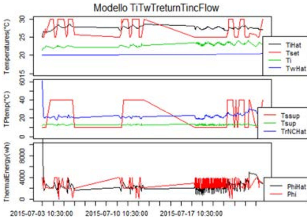
Figura 2.53 TiTwTreturnTincFlow con le sole stanze non controllate
