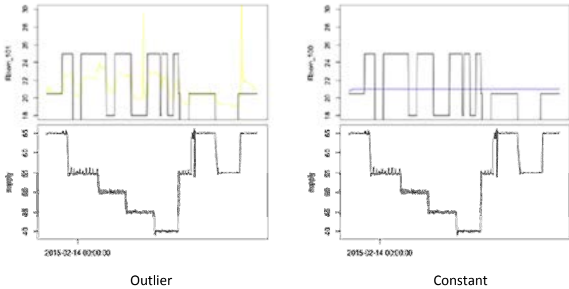
Figura 2.28 risultati comportamento stanze
