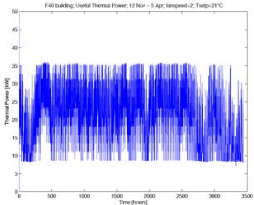
Figura 2.66. potenza termica invernale
