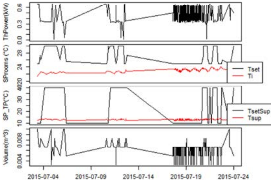
Figura 2.46 analisi comportamento F40
