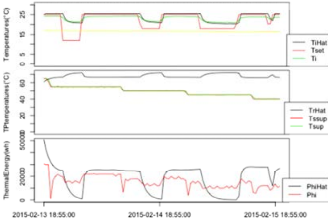
Figura 2.31 risultati modello vecchio
