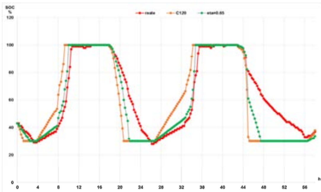
Figura 2.62 Confronto dell'andamento del SOC tra le ultime simulazioni ed i dati sperimentali
