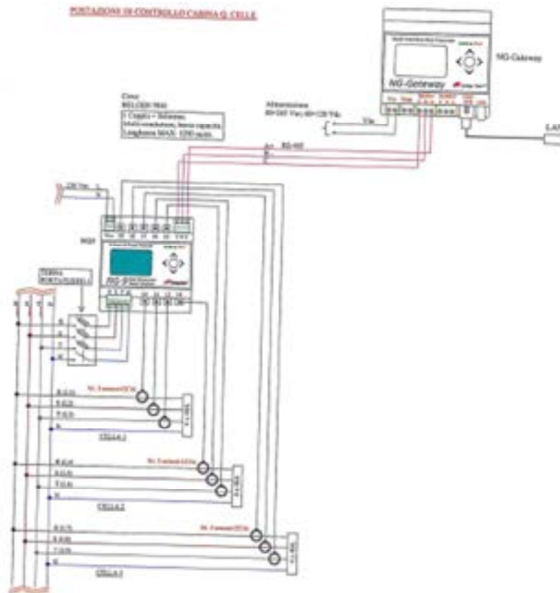
Figura 2.79 Schema tecnico
