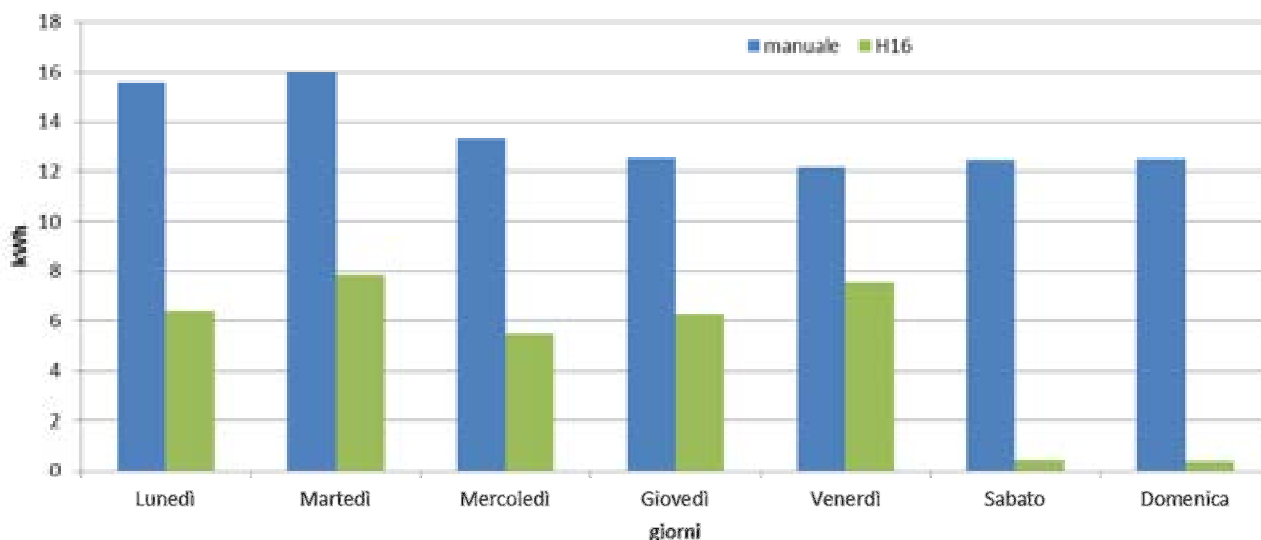
Figura 2.21 confronto settimanale strategie linea cdz (ed. F73)
