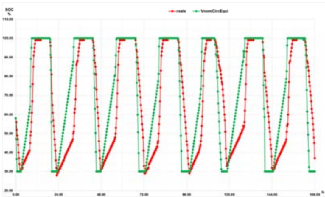
Figura 2.61 Confronto dell'andamento del SOC tra le prime simulazioni ed i dati sperimentali
