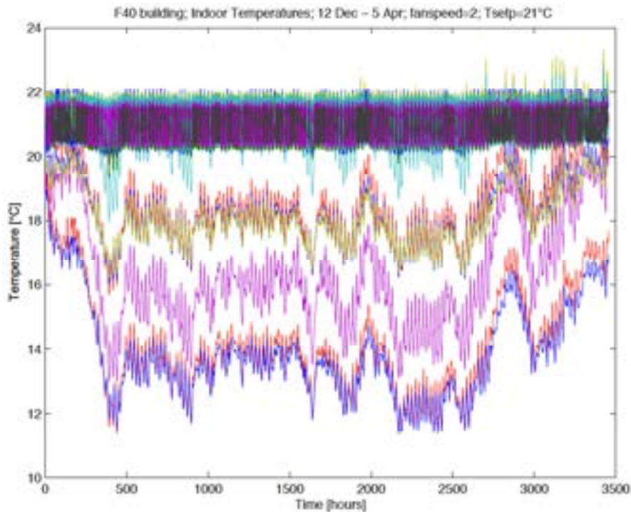
Figura 2.65. temperature interne invernali
