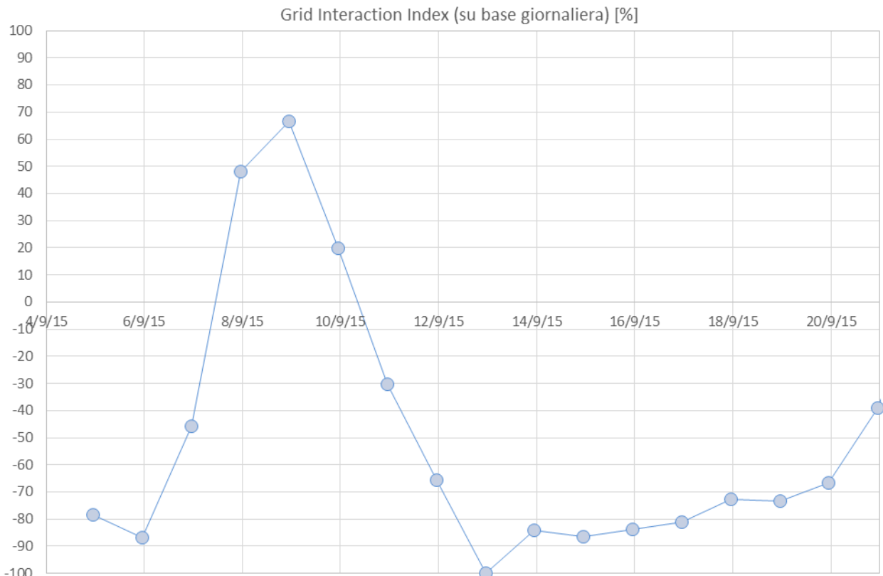
Figura 34. Indice di grid interaction calcolato su base giornaliera in periodo caldo (settembre)
