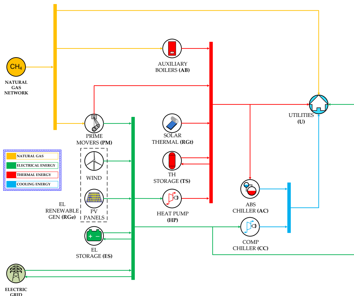
Figura 31 – Schema della smart grid ottimizzata dal software EGO 1.0
