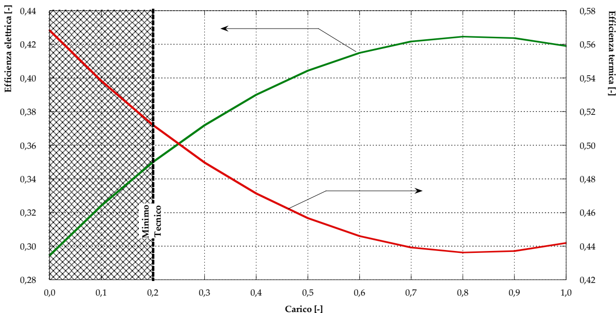
Figura 18 – Andamento delle efficienze elettrica e termica del motore a combustione interna al variare del carico
