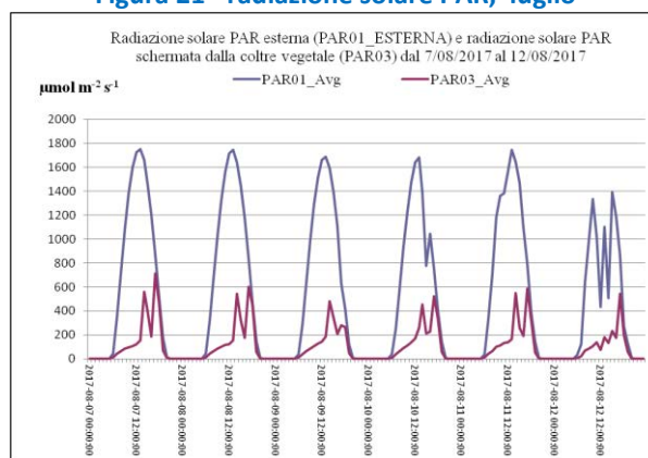
Figura 23 - radiazione solare PAR, agosto
