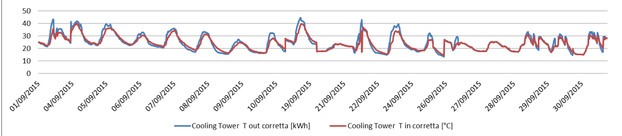
Figura 76 - Temperature torre evaporativa, settembre 2015
