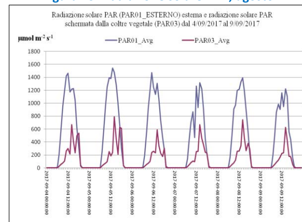
Figura 25 - radiazione solare PAR, settembre
