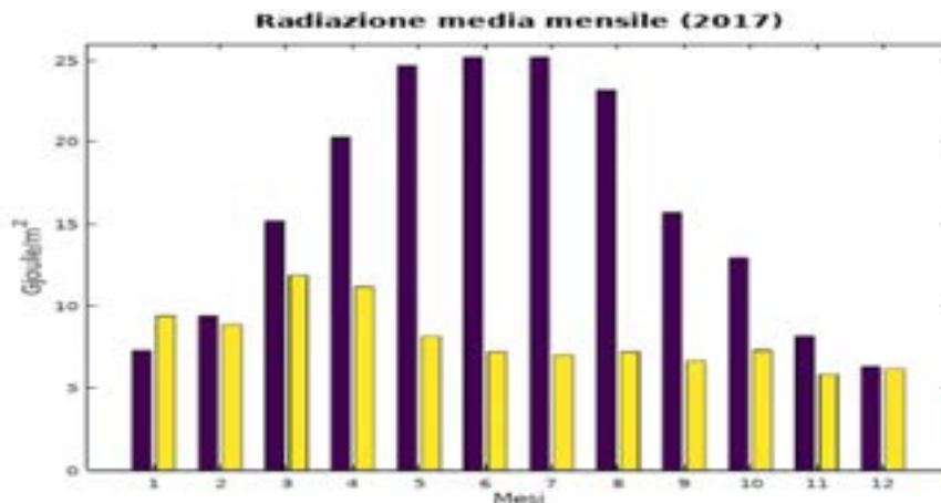
Figura 33 - Radiazioni giornaliere medie rilevate dal sensore posto sul tetto ( barre viola ) e dal sensore tra coltre e muro sulla parete Sud Ovest ( giallo )
