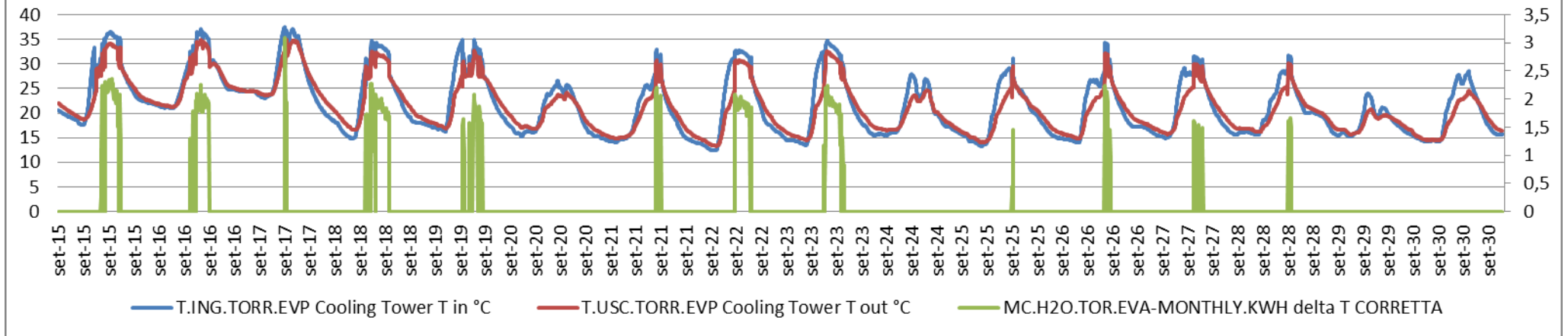
Figura 94 - Temperature torre evaporativa, settembre 2017
