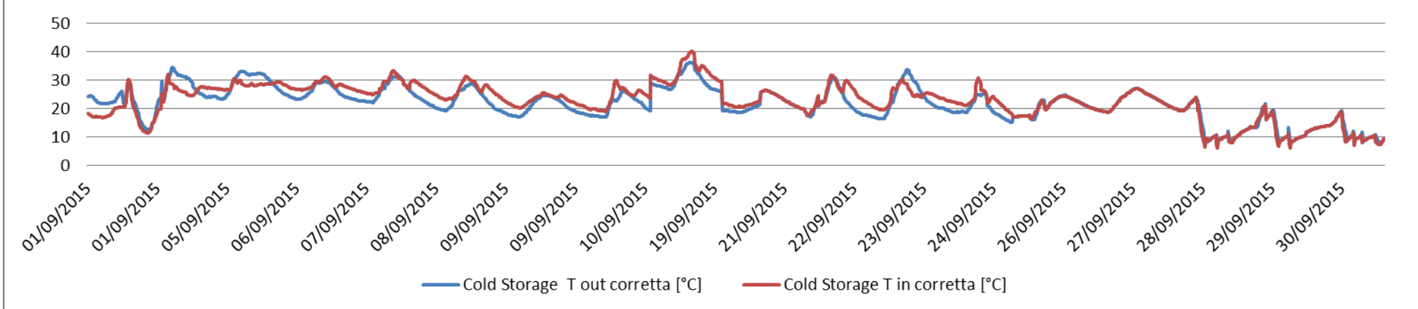
Figura 75 - Temperature acqua refrigerata all'uscita dalla macchina ad assorbimento, settembre 2015
