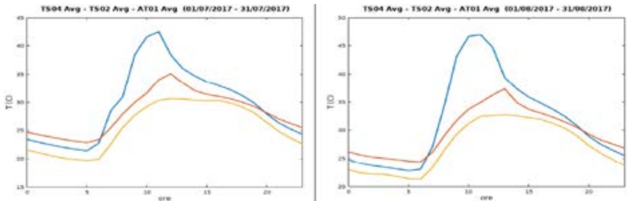
Temperatura media della parete Sud Est nei mesi di luglio (a sinistra) e agosto (a destra) Blu: temperatura della zona esposta al sole; Rosso: temperatura della zona protetta dalla coltre verde; Giallo: temperatura dell'aria
