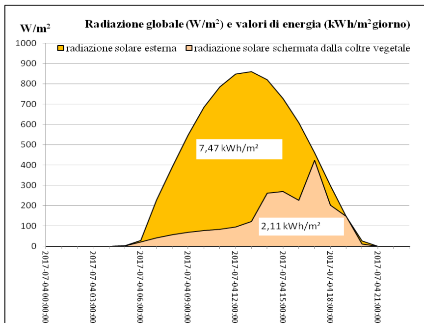
Figura 17 - radiazione solare globale
