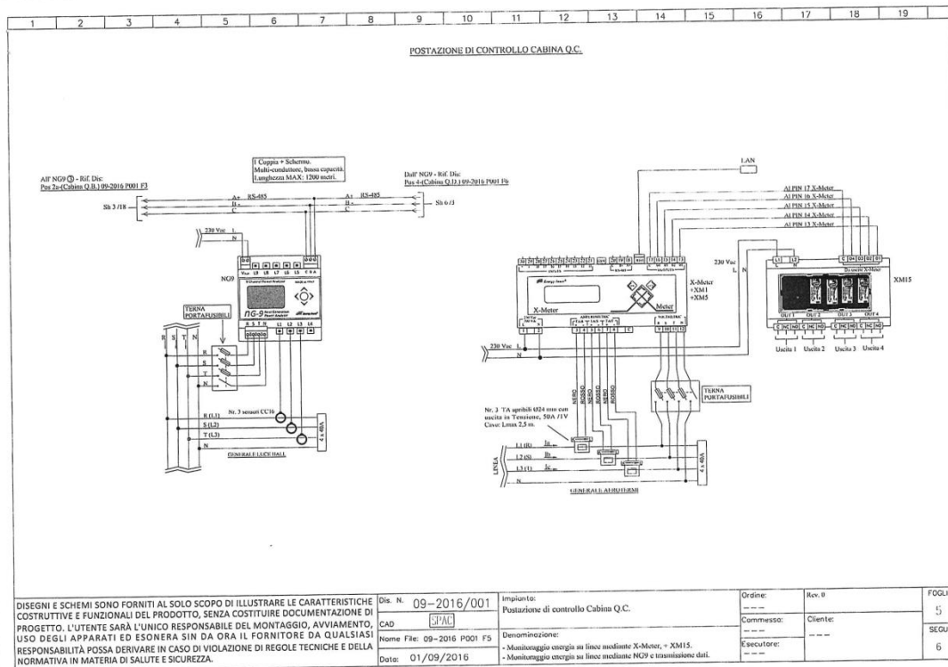
Figura 22 - Quadro C
