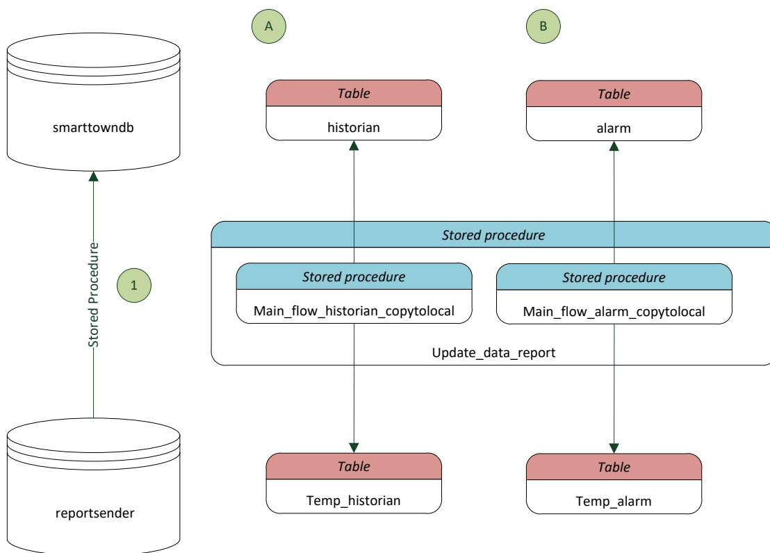
Figura 7 - flusso informazioni
