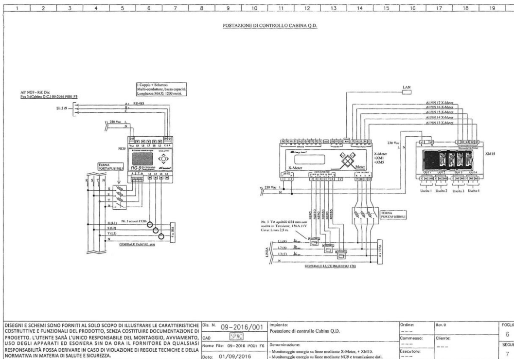
Figura 23 - Quadro D
