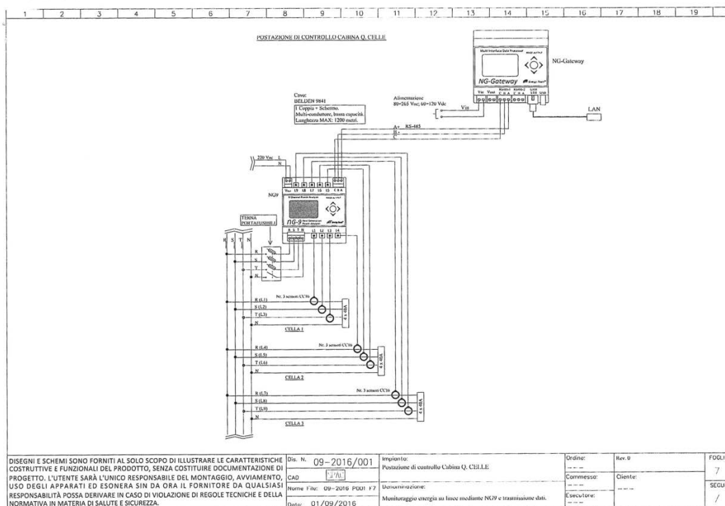
Figura 24 - Quadro Celle
