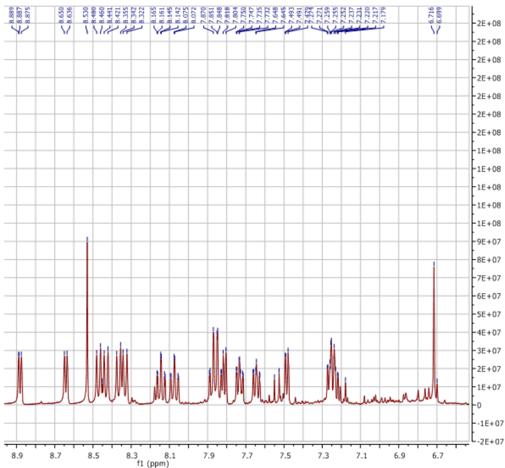
Figura 50. Spettro ^1\text{H} NMR ( \text{CD}_2\text{Cl}_2 ) di 16, espansione regione a bassi campi.
