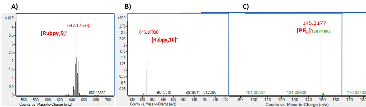
Figura 66. Spettro ESI(+) MS di 16 (A), spettro ESI(+) MS di 17 (B) spettro ESI(-) MS di 16 e 17 (C).
