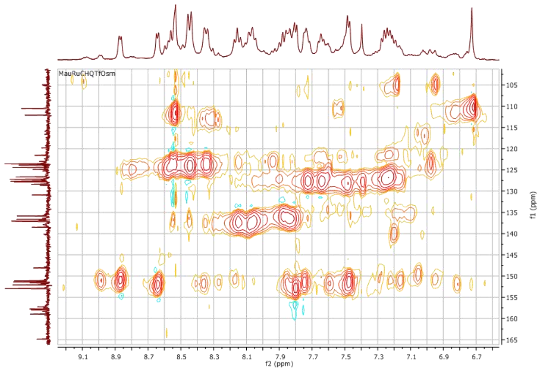
Figura 71. Spettro ^1\text{H} , ^{13}\text{C} HSQC ( \text{CD}_2\text{Cl}_2 ) di 18, espansione regione a campi bassi.
