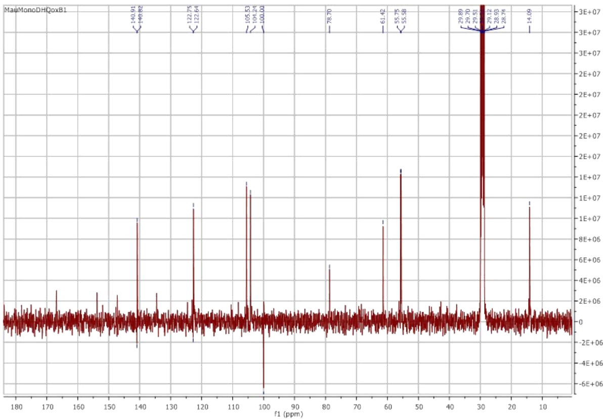
Figura 33. Spettro ^{13}\text{C} NMR (Acetone- d_6 ) di 13.
