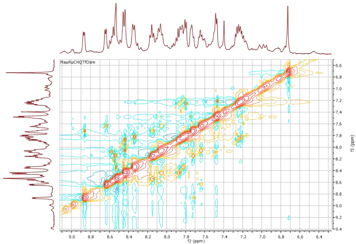
Figura 70. Spettro ^1\text{H},^1\text{H} COSY ( \text{CD}_2\text{Cl}_2 ) di 18, espansione regione a campi bassi.
