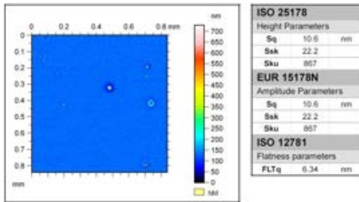
Figura 104: Caratterizzazione al profilometro ottico del film PEDOT:PSS+Blend al 8% di 16 in CBP
