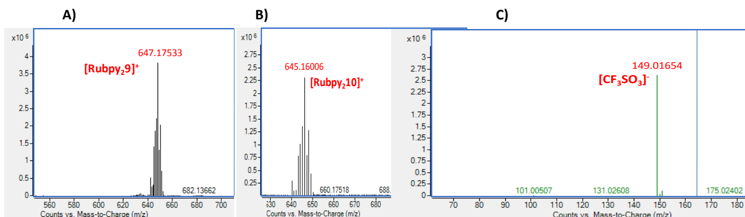
Figura 82. Spettro ESI(+) MS di 18 (A), spettro ESI(+) MS di 19 (B) spettro ESI(-) MS di 18 e 19 (C).
