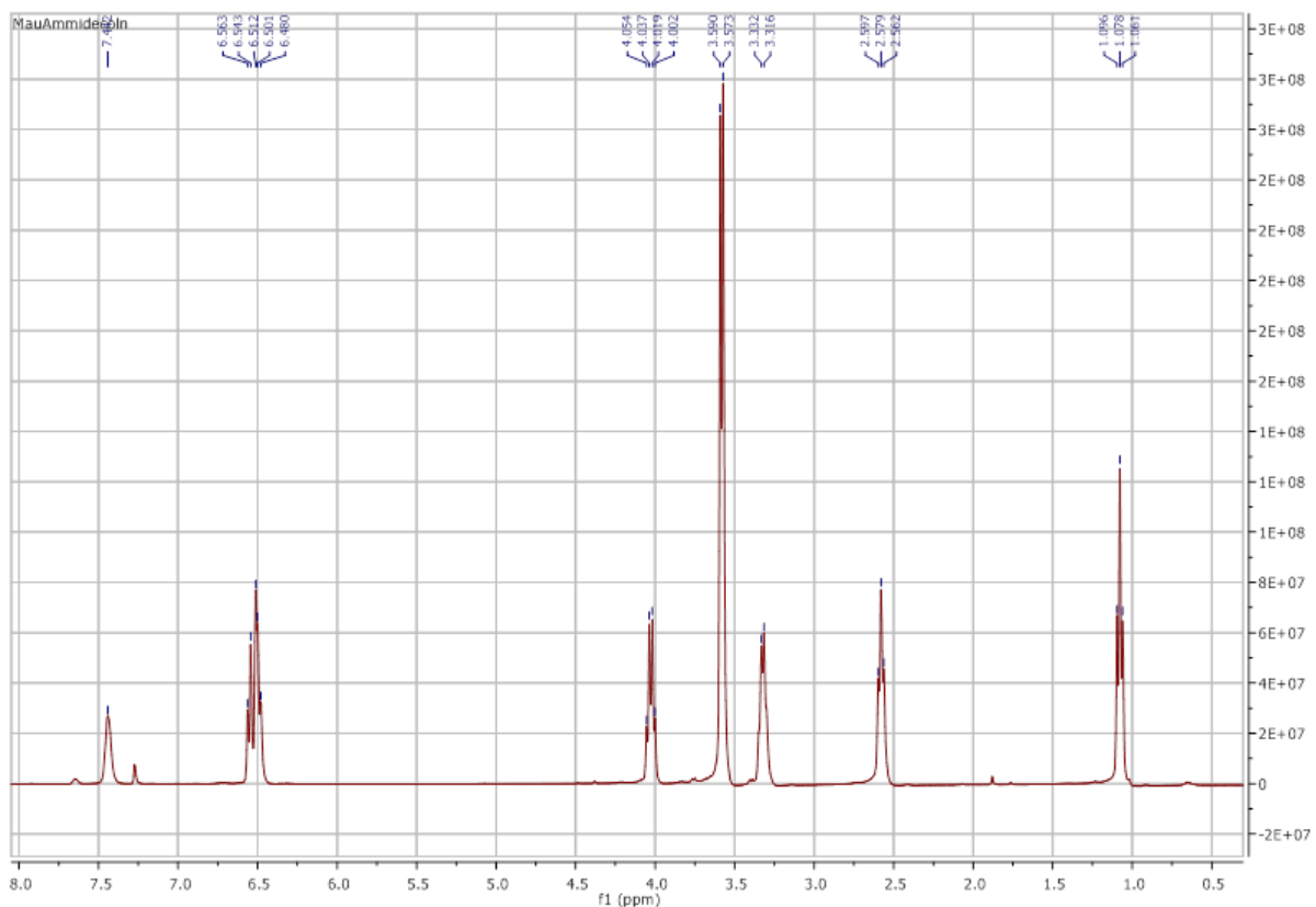
Figura 26. Spettro ^1\text{H} NMR (CDCl 3 ) di 11 .
