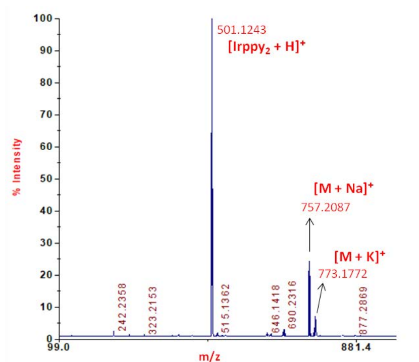
Figura 46. Spettro MALDI MS di 14.
