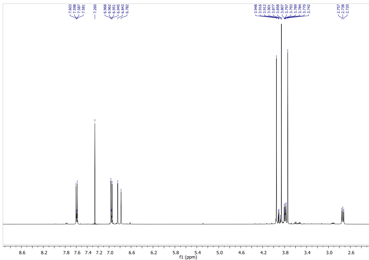
Figura 3. Spettro ^1\text{H} NMR ( \text{CDCl}_3 ) di 1.
