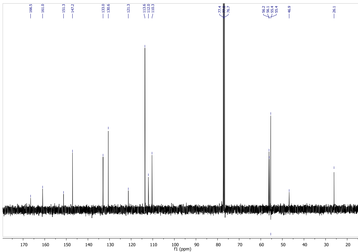
Figura 4. Spettro ^{13}\text{C} NMR ( \text{CDCl}_3 ) di 1.
