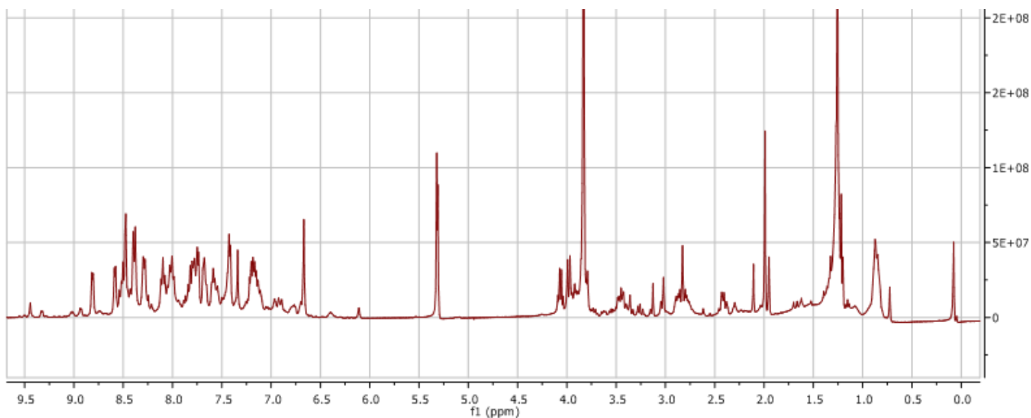
Figura 68. Spettro 1 H NMR (CD 2 Cl 2 ) di 18 .
