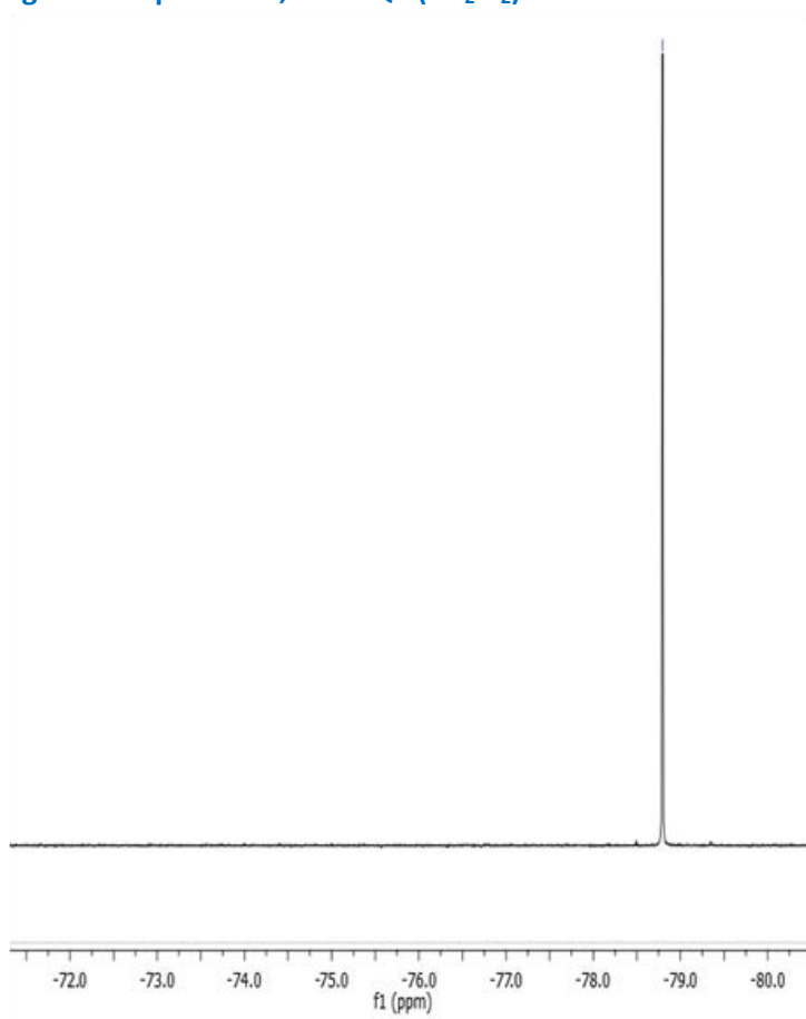
Figura 81. Spettro ^{19}\text{F} NMR ( \text{CD}_2\text{Cl}_2 ) di 19.
