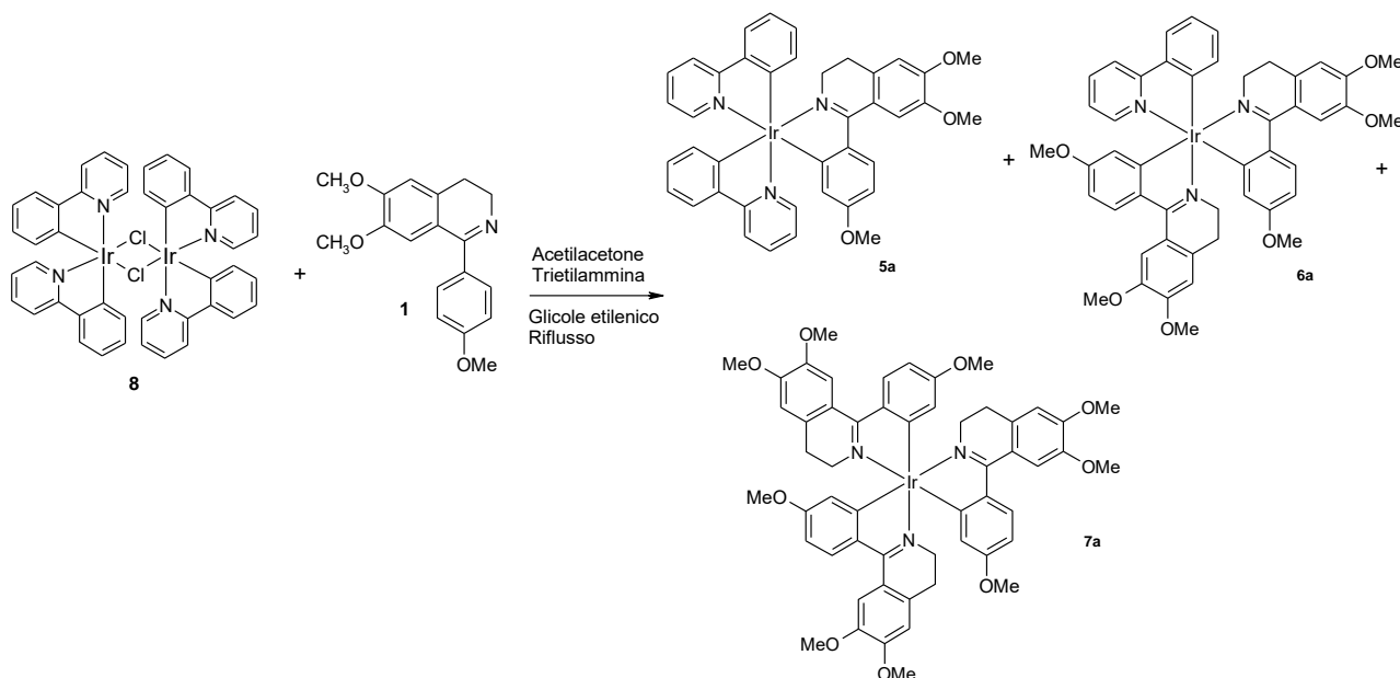
Figura 9. Sintesi dei complessi bio-ispirati 5a, 6a e 7a.
