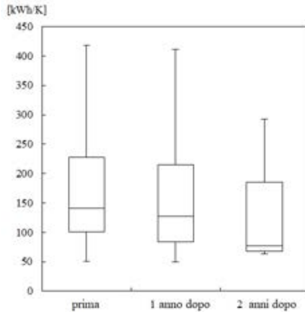
Figura 1 – Consumi energetici prima e dopo l’installazione dei sistemi di contabilizzazione
