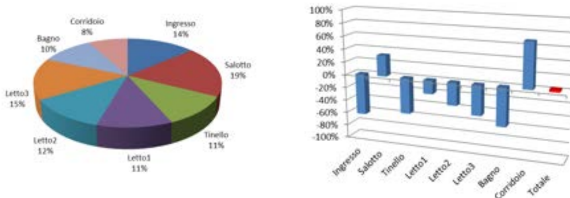
Figura 32 - Ripartizione dei consumi e del risparmio negli ambienti (AP_1)
