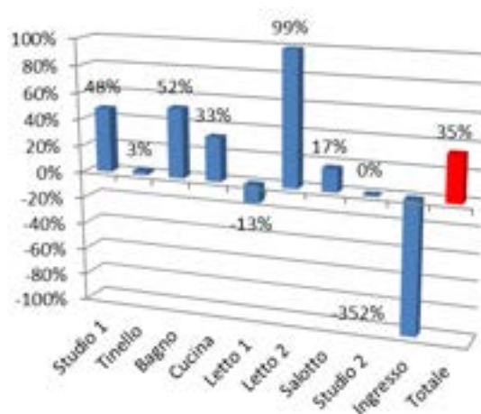
Figura 35 - Ripartizione dei consumi e del risparmio negli ambienti (AP_4)
