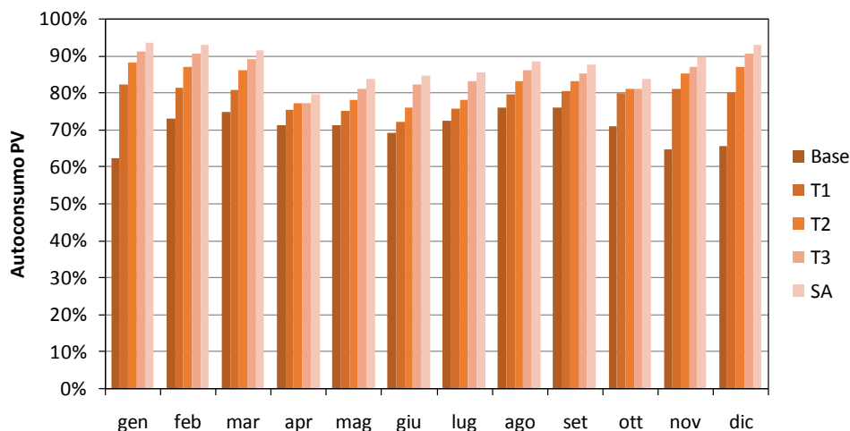
Figura 37. Risultati delle simulazioni: autoconsumo PV
