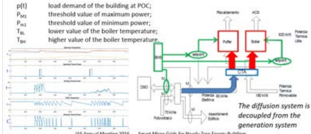
Figura 31. Scheda del controllo del boiler
