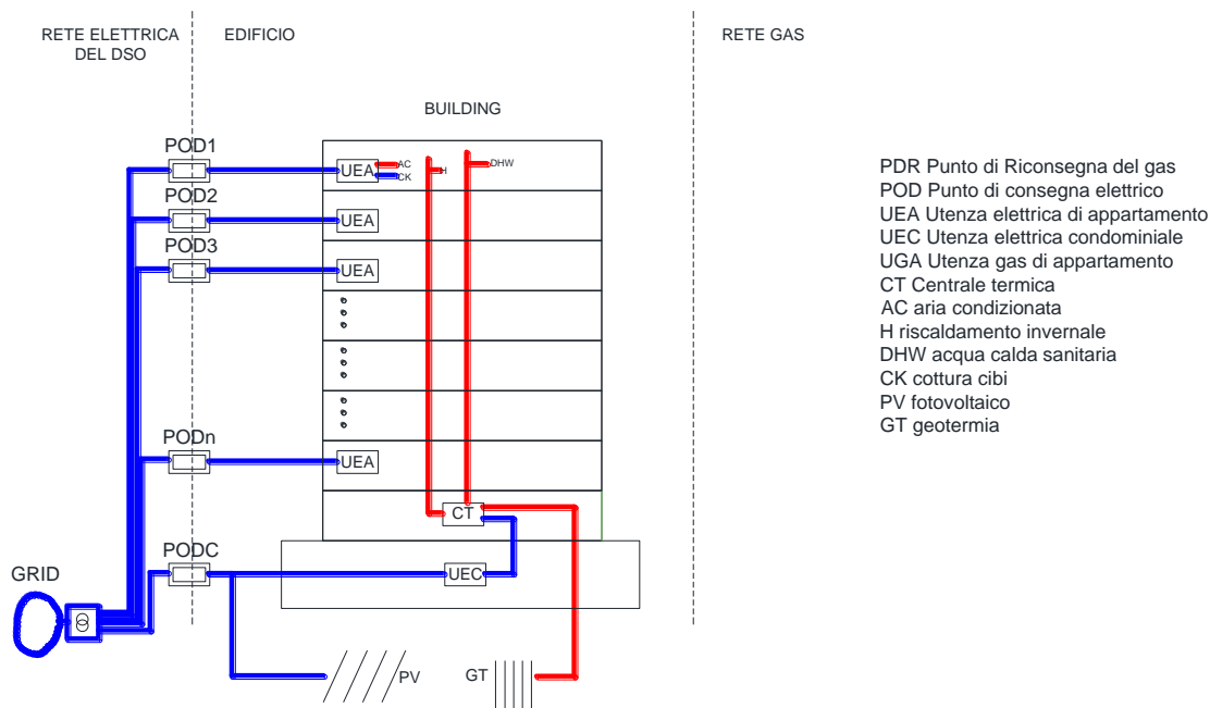
Figura 16. Esempio di microgrid per un MURB. I POD delle singole utenze sono necessari per la ripartizione dei costi energetici.
