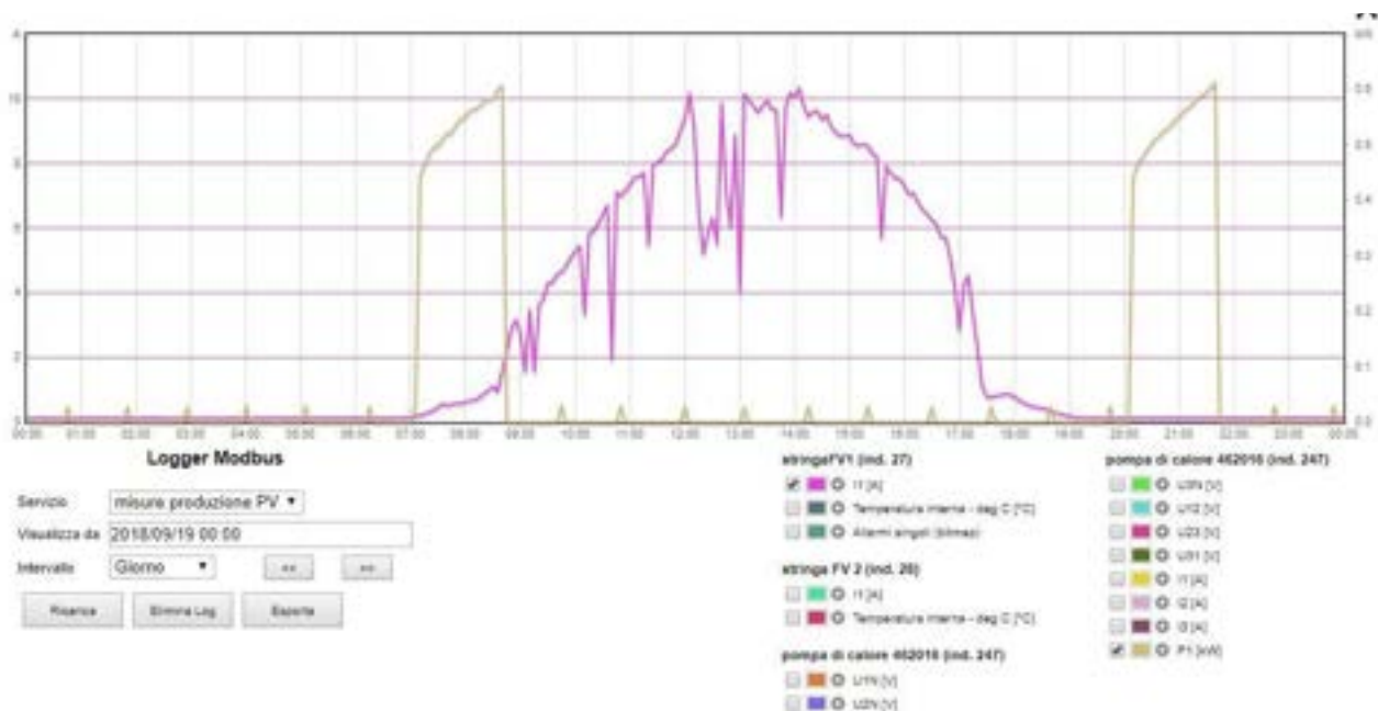
Figura 64: piattaforma web per il monitoraggio e la memorizzazione delle misure dell'impianto sperimentale (giallo: potenza assorbita dalla pompa di calore (kW), fucsia corrente erogata dalla stringa 1 (A))
