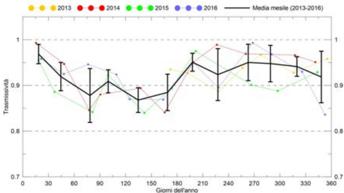
Figura 96. Andamento della trasmissività della finestra del fotometro SP02 dovuta alla deposizione dell'aerosol per i mesi che vanno da Giugno 2013 a Dicembre 2016. La linea nera con le barre di incertezza rappresenta l'andamento medio derivato della trasmissività stimata dai 4 anni di osservazioni.
