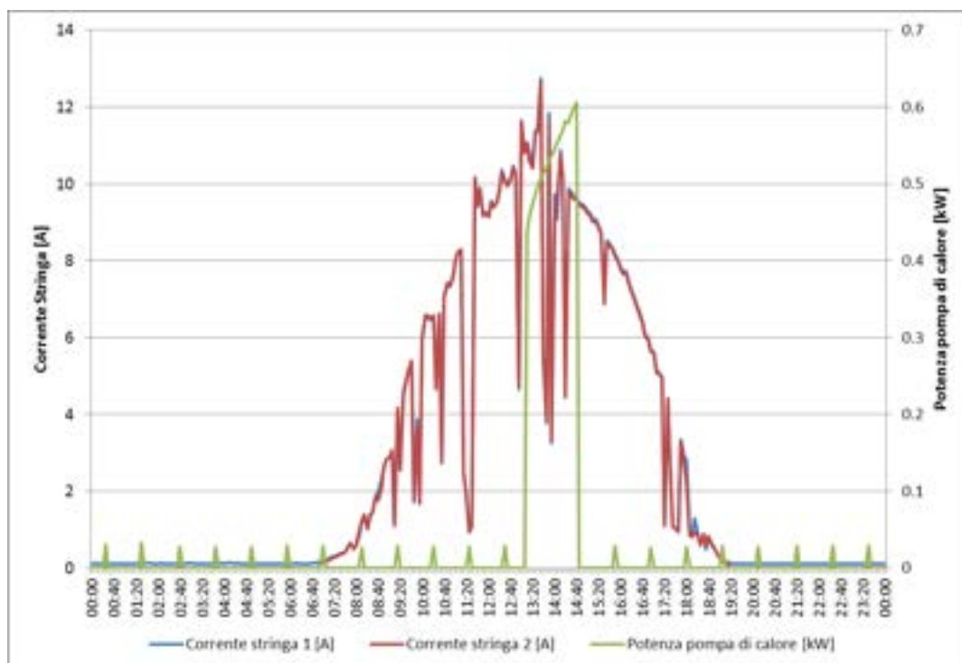
Figura 66: profilo di consumo della pompa di calore e produzione dell'impianto FV locale giorno 15 Settembre
