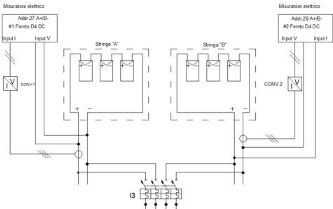
Figura 89: schema di connessione in cortocircuito delle due stringhe FV e inserimento degli strumenti di misura
