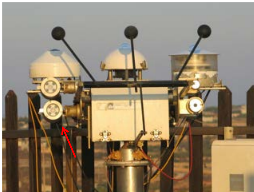
Figura 92. Inseguitore solare Kipp and Zonen 2AP equipaggiato con un pirgeometro, due piranometri, un pireliometro e due fotometri Middleton evidenziati dalla freccia rossa.
