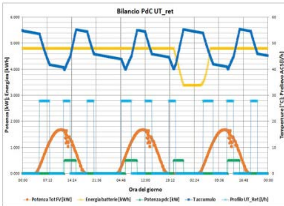
Figura 70: Simulazione sistema ibrido sperimentale – applicazione del profilo di consumo ACS rettangola relativo all’utente reale funzionamento della pompa di calore con termostato
