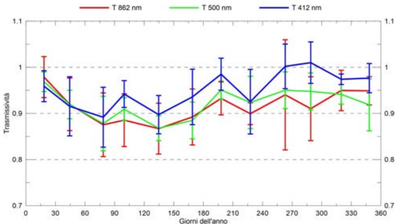
Figura 97. Andamento della trasmissività media mensile per il periodo 2013-2016 a 3 lunghezze d'onda (412, 500 e 862 nm).
