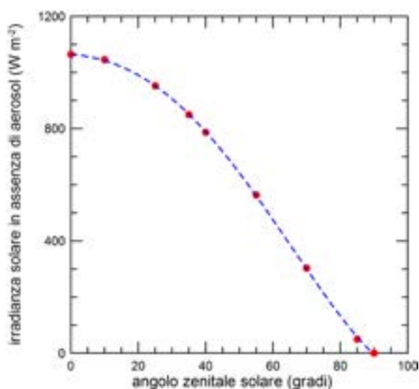
Figura 80. I punti rossi mostrano l'irradianza solare orizzontale calcolata con il modello di trasferimento radiativo MODTRAN a diversi valori di angolo zenitale solare. La curva blu è un fit polinomiale di quarto grado ai dati.
