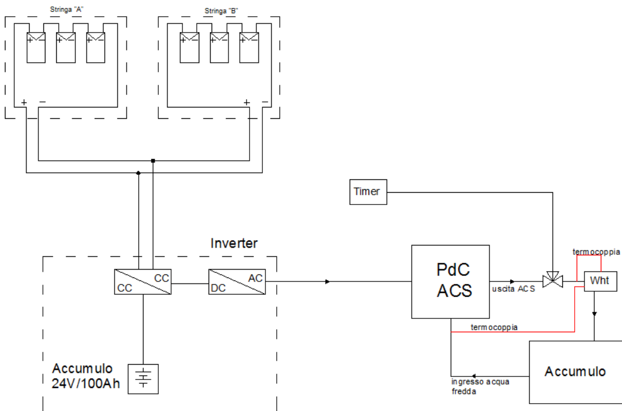
Figura 55: schema semplificato impianto sperimentale Pompa di calore per ACS + FV + accumulo elettrico
