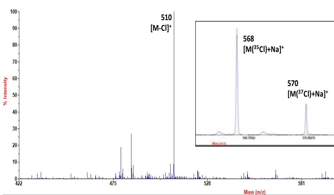
Figura 36. Spettro MALDI del complesso 7.
