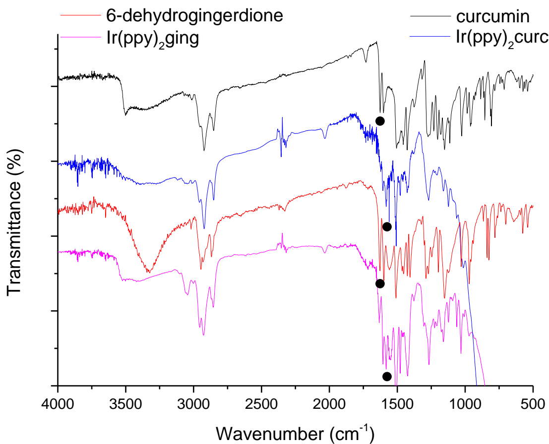
Figura 21. Spettri FT-IR di 1 (traccia nera), 2 (traccia rossa), 3 (traccia blu) e 4 (traccia viola).
