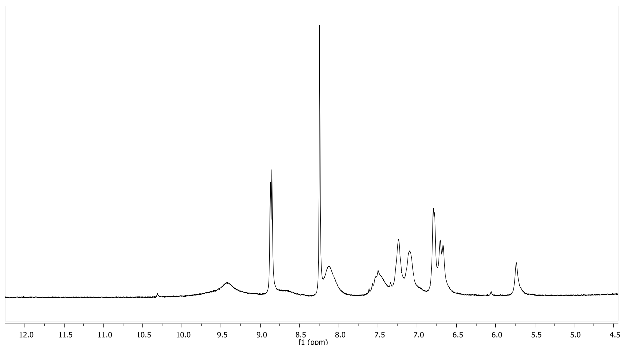
Figura 39. Spettro ^1\text{H} NMR (DMSO- d_6 ) del complesso 6 (espansione della regione a campi bassi).
