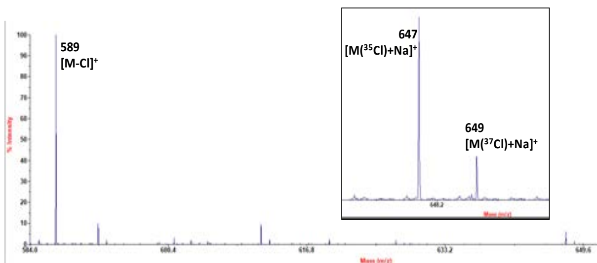
Figura 33. Spettro MALDI del complesso 5.
