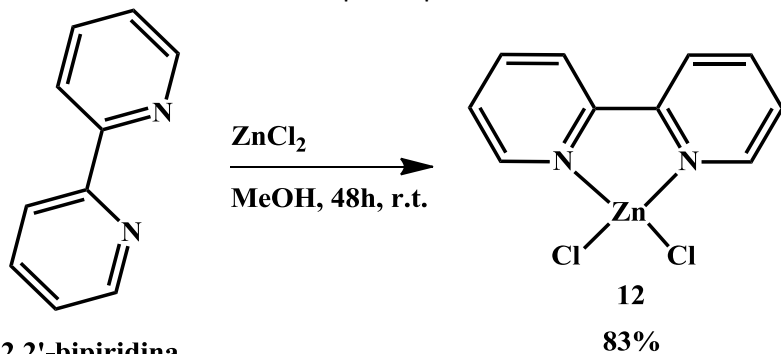
Figura 30. Sintesi del precursore 12.
