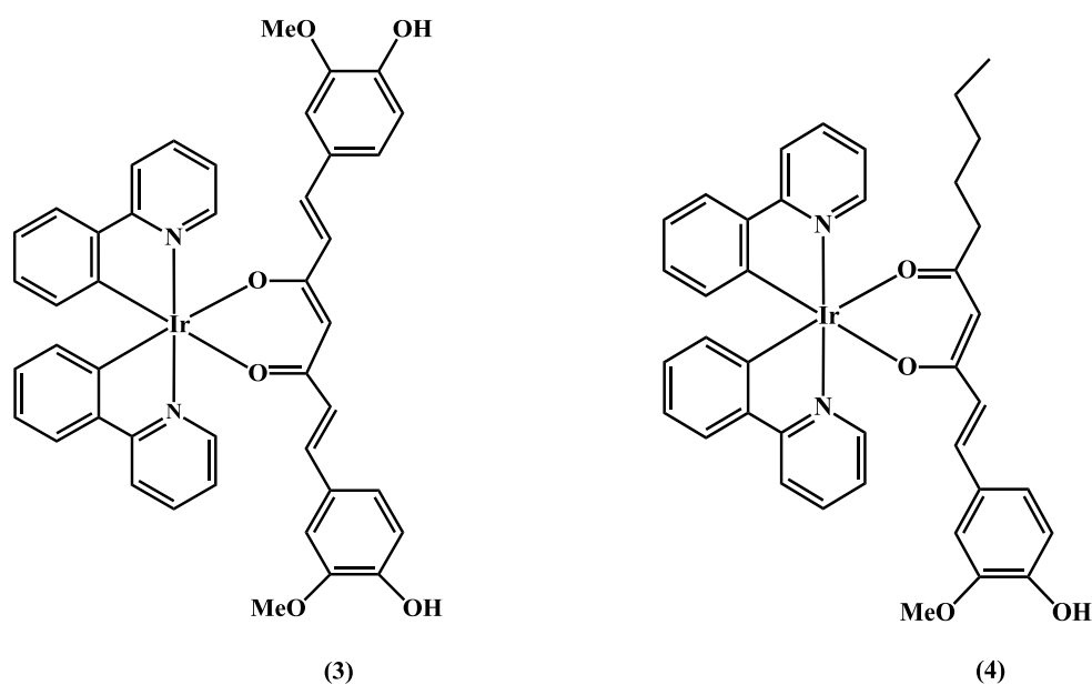
Figura 9. Complessi dell'iridio(III) sintetizzati con i leganti 1 e 2 .
