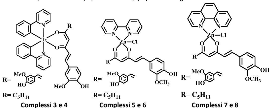
Figura 4. Complessi di metalli di transizione sintetizzati.
