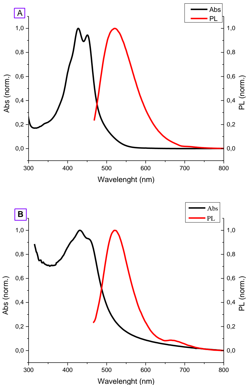
Figura 47. Spettri Uv-vis del complesso 5 in soluzioni diluite di DMSO (A) e su film sottile (B)
