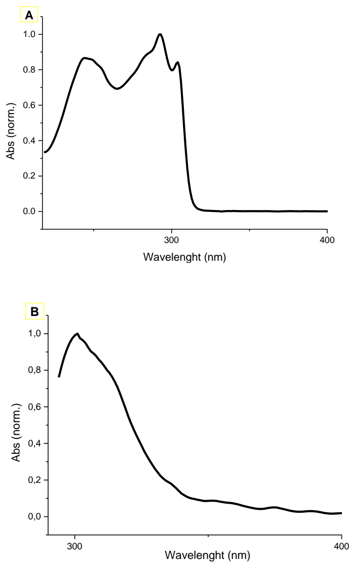
Figura 45. Spettri Uv-vis del complesso 12 in soluzioni diluite di H 2 O (A) e su film sottile (B)
