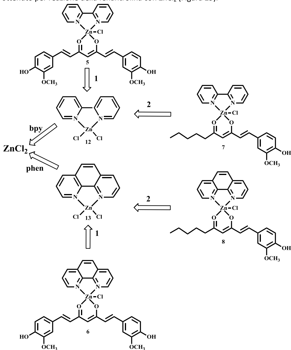
Figura 29. Schema retro-sintetico per la preparazione dei complessi 5-8.
