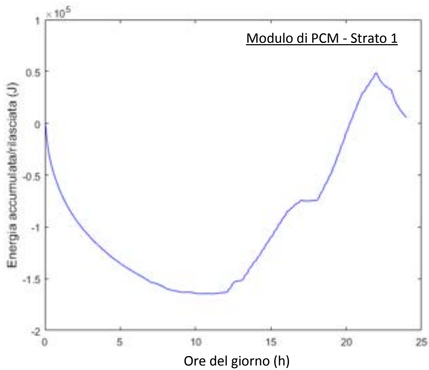
Figura 9. Andamento dell'energia accumulata/riasciata dal modulo di PCM appartenente allo strato 1.
