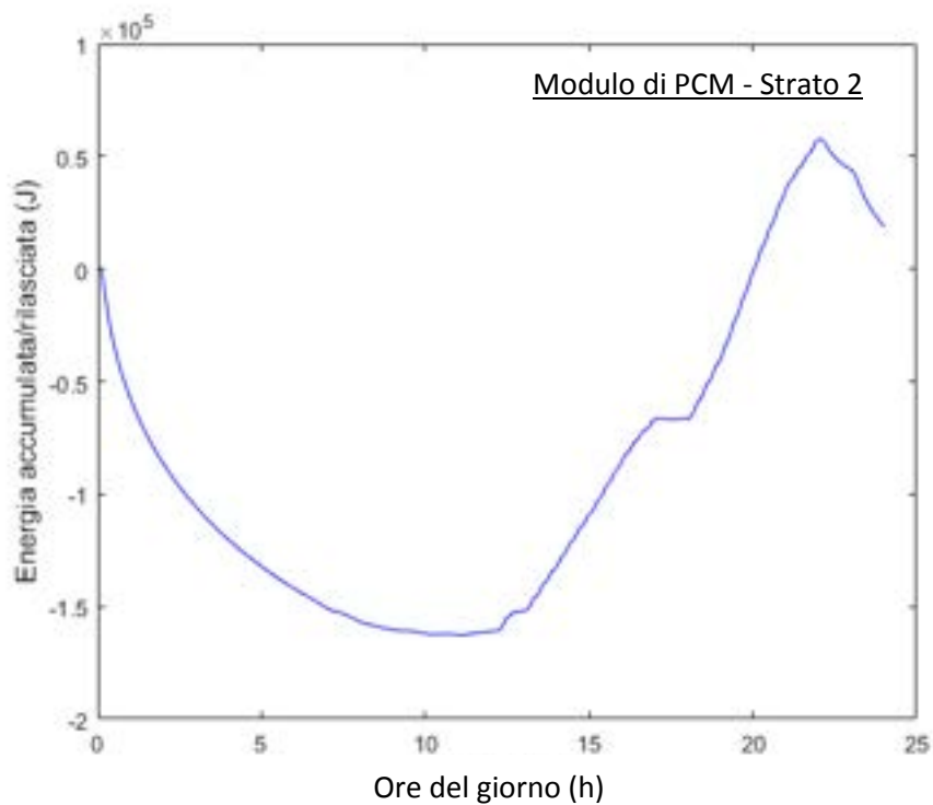
Figura 10. Andamento dell'energia accumulata/riasciata dal modulo di PCM appartenente allo strato 2.
