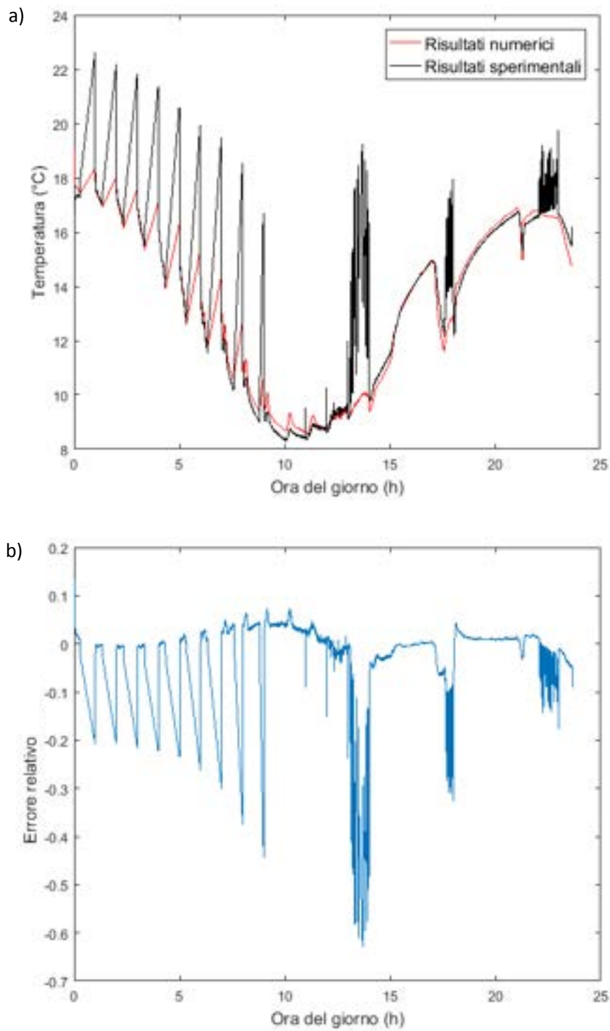
Figura 16. Correlazione di Prabhanjani: a) confronto tra i dati sperimentali e i dati numerici; b) errore relativo medio.
