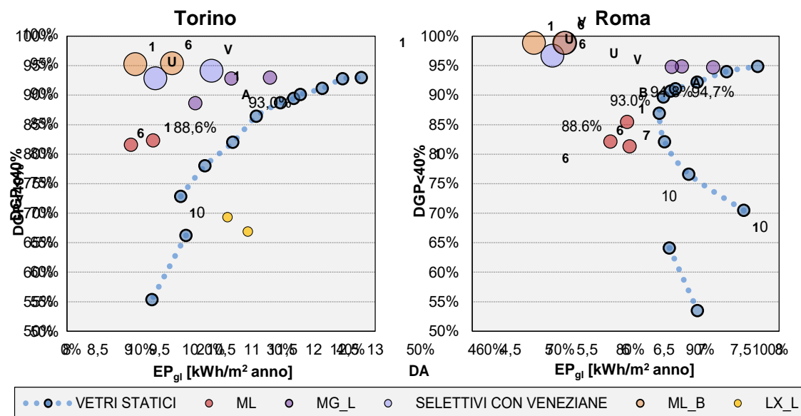
Figura 30. Correlazione di EP_{gl} e DGP < 40\% per le strategie di controllo esaminate nei climi di Torino e Roma.
