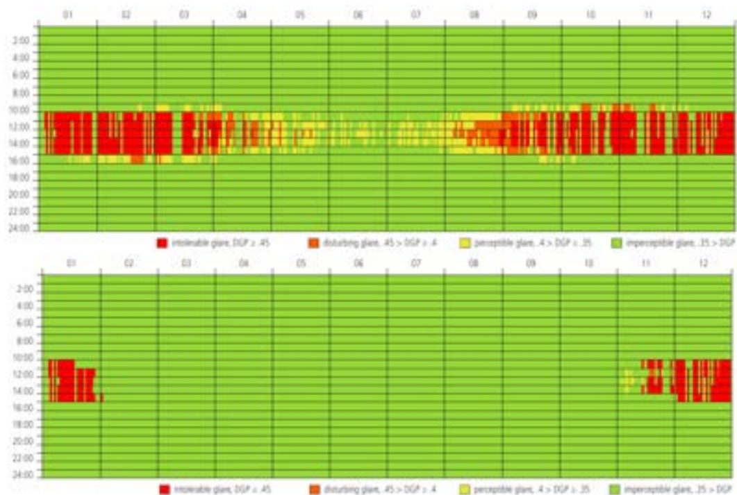
Figura 16. Daylight Glare Probability per vetro elettrocromico allo stato di massima trasparenza (sopra) e di massima colorazione (sotto).
