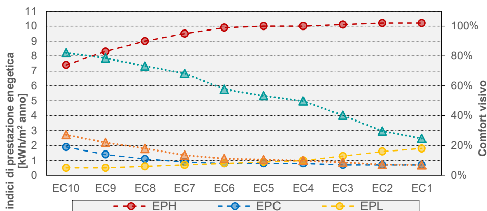
Figura 15. Prestazione energetica e di comfort visivo annuali per i 10 stati di colorazione che il componente elettrocromico può assumere.
