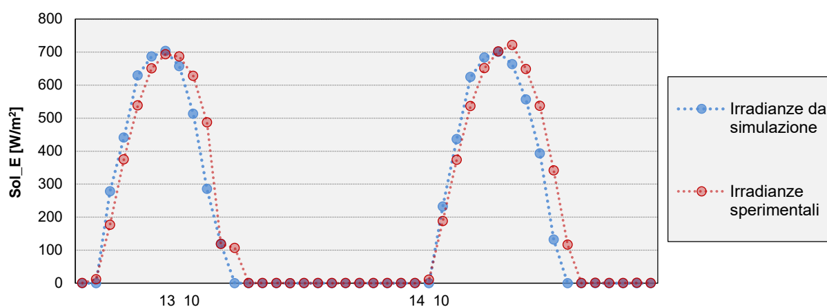
Figura 13. Confronto tra irradianze registrate sperimentalmente e immesse in simulazione per giornate comparabili.
