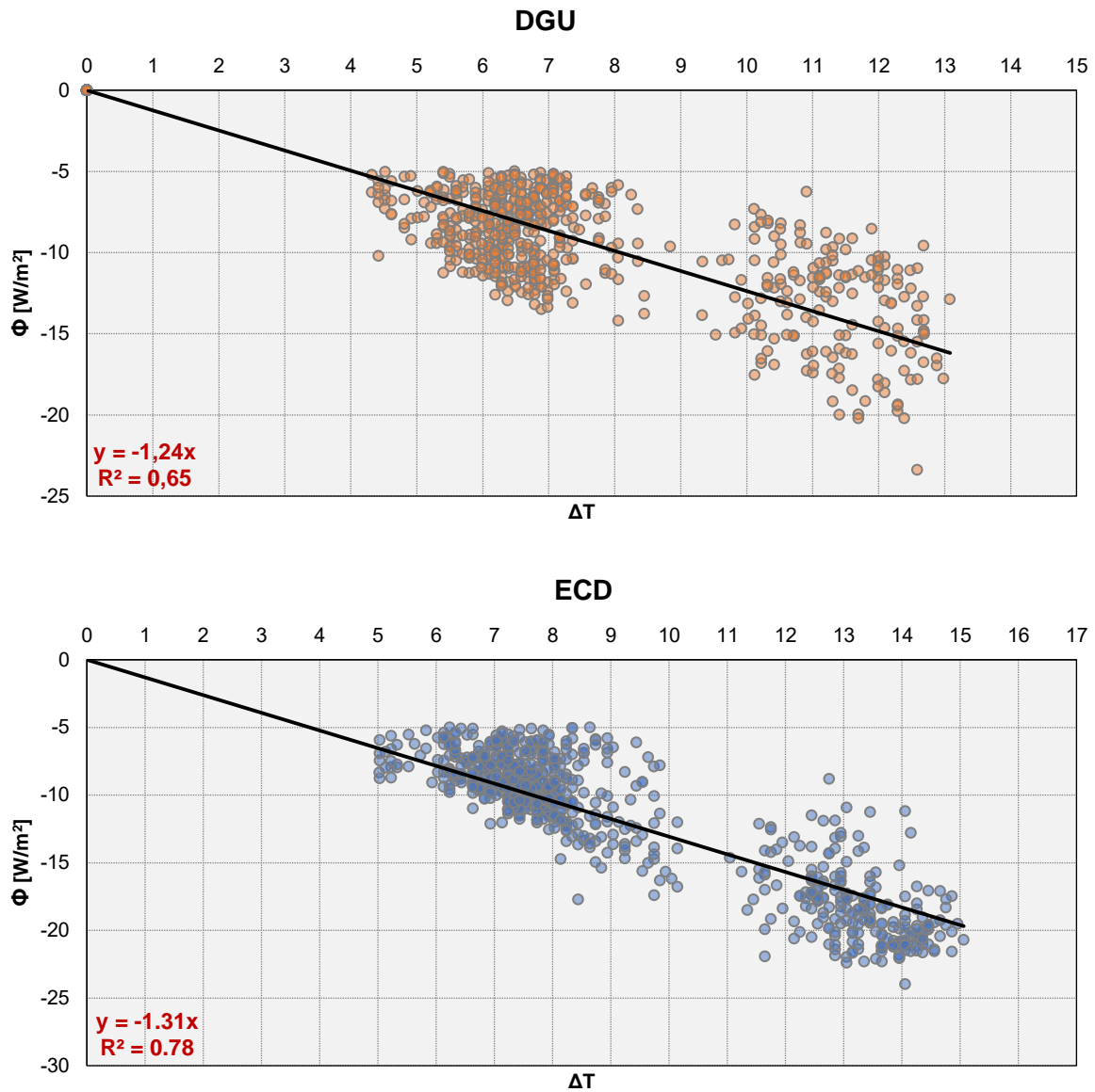
Figura 6. Interpolazione lineare per il calcolo della trasmittanza termica per vetrocamera convenzionale DGU (in alto) ed elettrocromico assemblato in vetrocamera ECD (in basso).
