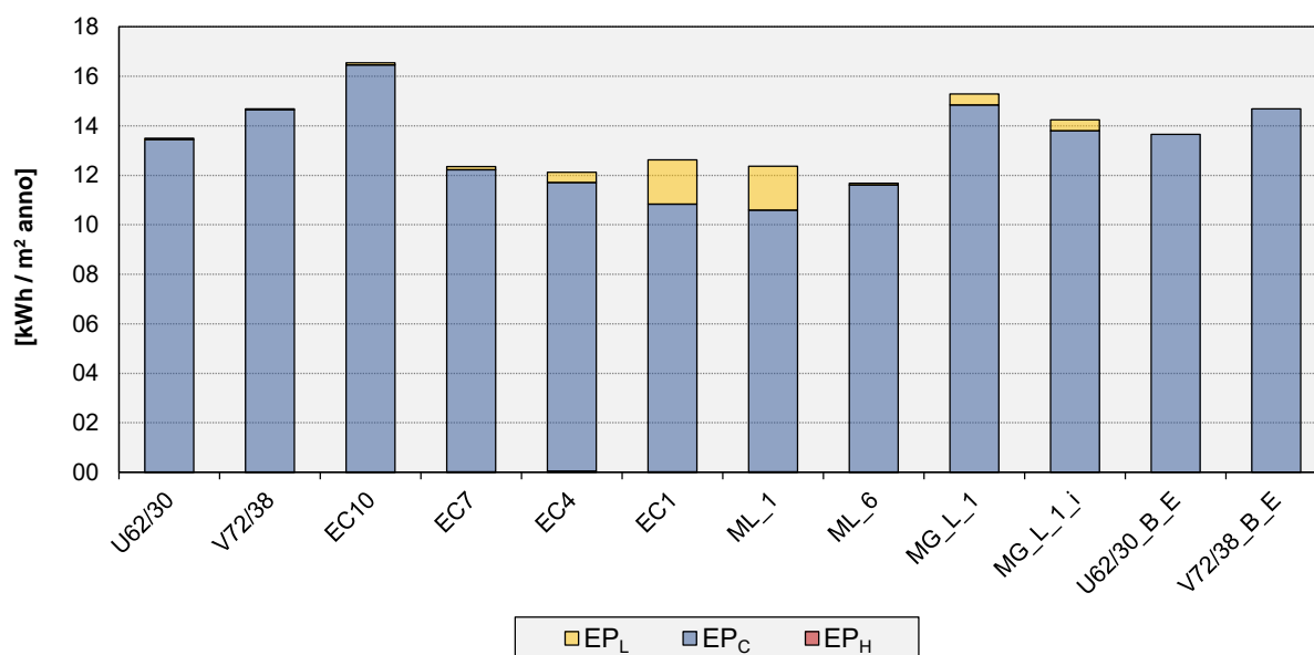
Figura 25. Indice di prestazione energetica per riscaldamento, raffrescamento ed illuminazione per i vetri statici e le strategie di controllo investigate per il clima di Abu Dhabi.
