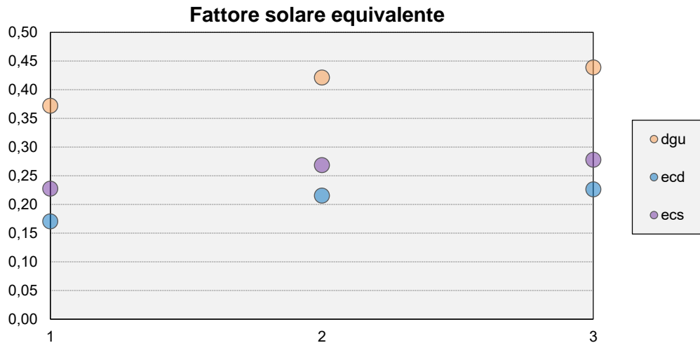
Figura 7. Fattore solare dei tre sistemi vetrati per tre condizioni climatiche diverse: 1) cielo coperto, 2) parzialmente coperto e 3) sereno. I dati relativi all'elettrocromico fanno riferimento allo stato intermedio 4.
