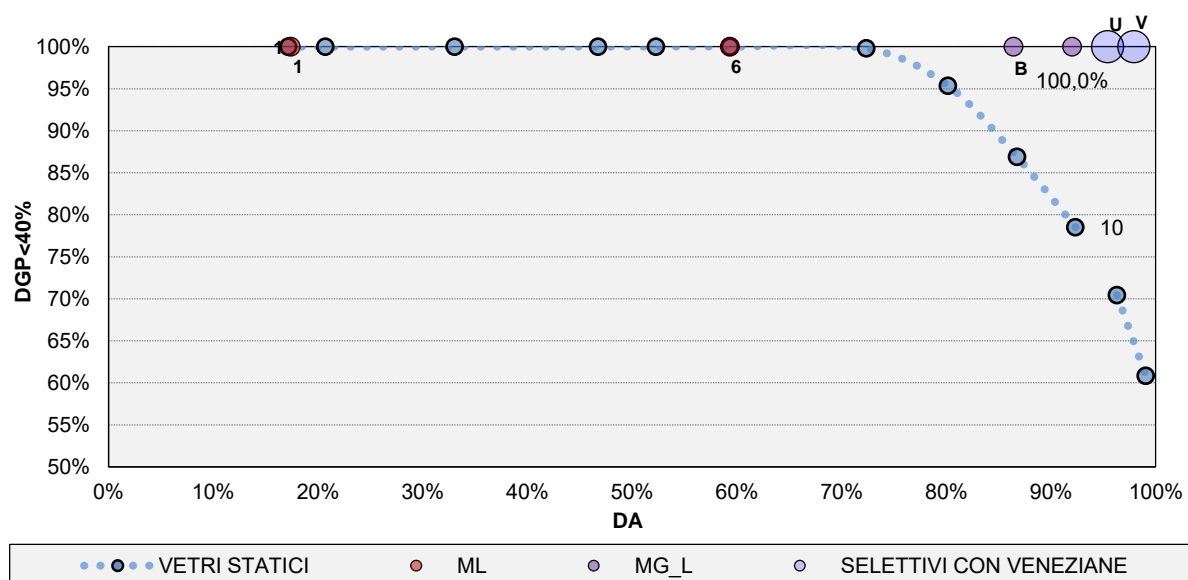
Figura 27. Correlazione di DA e DGP < 40\% per le strategie di controllo esaminate nel clima di Abu Dhabi.
