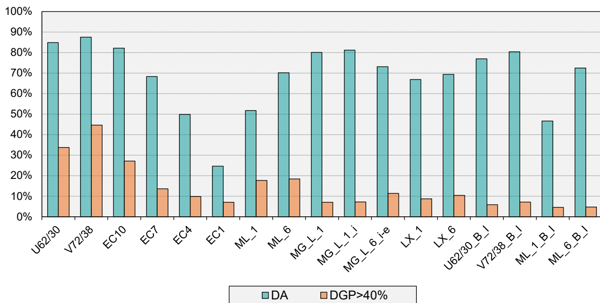
Figura 18. Daylight Autonomy (DA) e Daylight Glare probability (DGP) ottenuti per i vetri statici e le strategie di controllo investigate per il clima di Torino.
