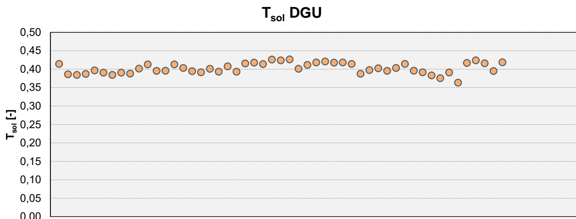
Figura 9. Trasmissione solare del vetrocamera di riferimento DGU.
