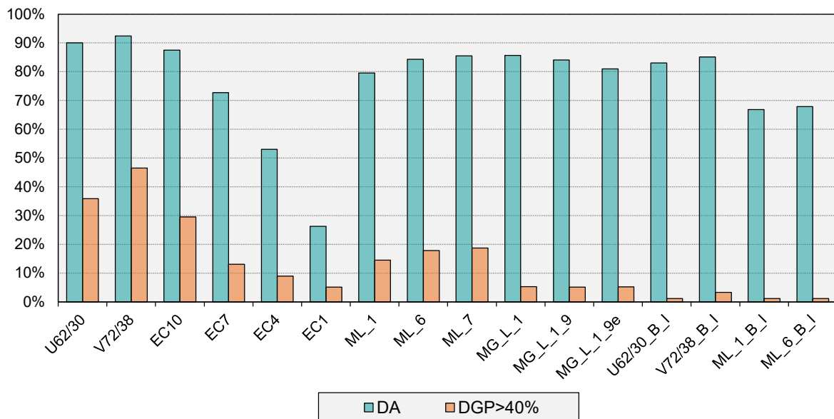
Figura 22. Daylight Autonomy (DA) e Daylight Glare probability (DGP) ottenuti per i vetri statici e le strategie di controllo investigate per il clima di Roma.
