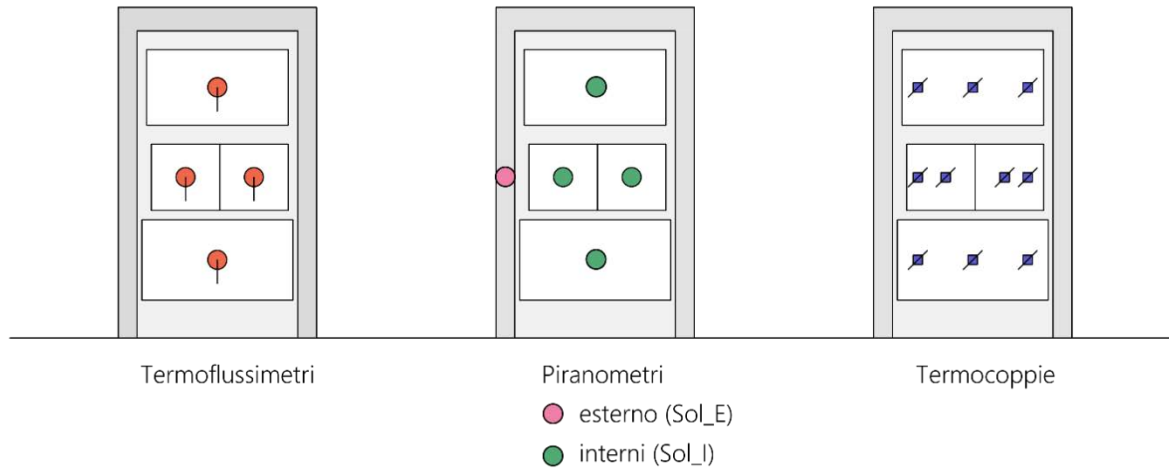
Figura 5. Schema dettagliato dei sensori utilizzati, con indicazione della loro posizione.
