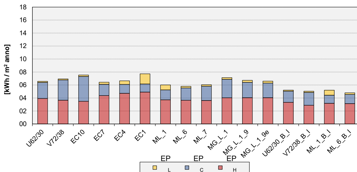
Figura 21. Indice di prestazione energetica per riscaldamento, raffrescamento ed illuminazione per i vetri statici e le strategie di controllo investigate per il clima di Roma.
