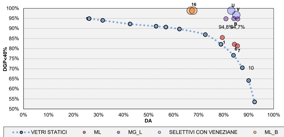
Figura 23. Correlazione di DA e DGP<40% per le strategie di controllo esaminate nel clima di Roma.
