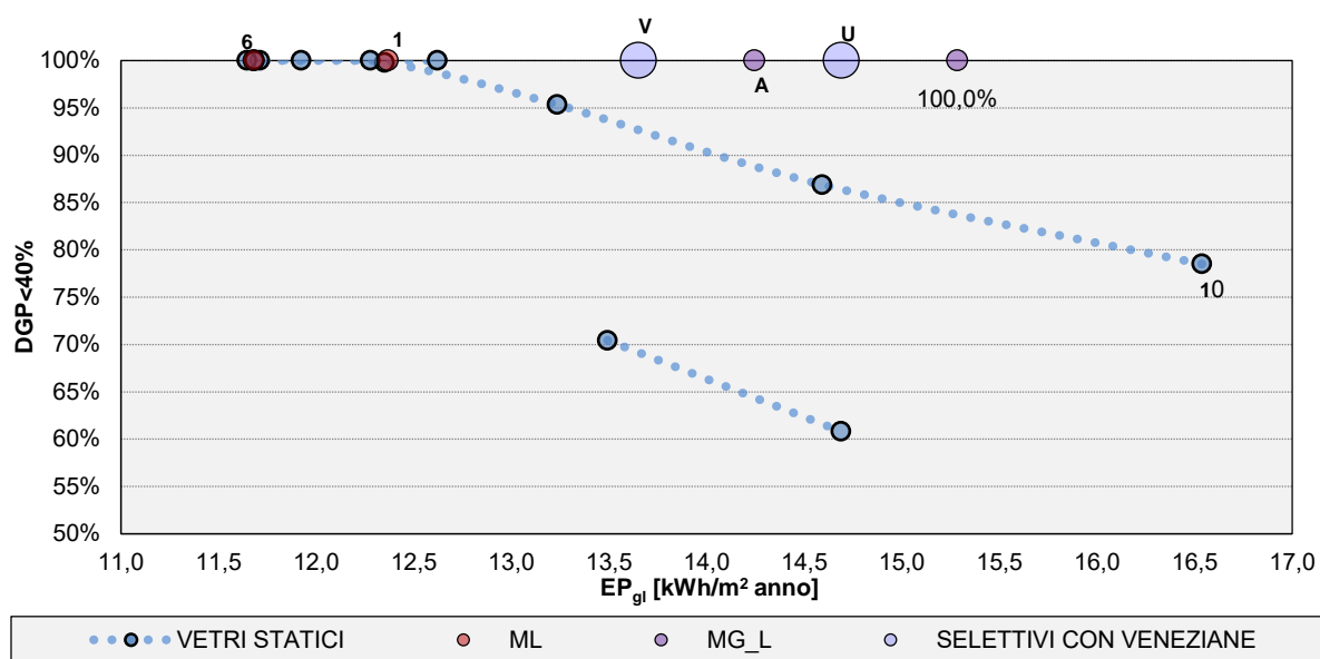
Figura 28. Correlazione di EP GL e DGP<40% per le strategie di controllo esaminate nel clima di Abu Dhabi.
