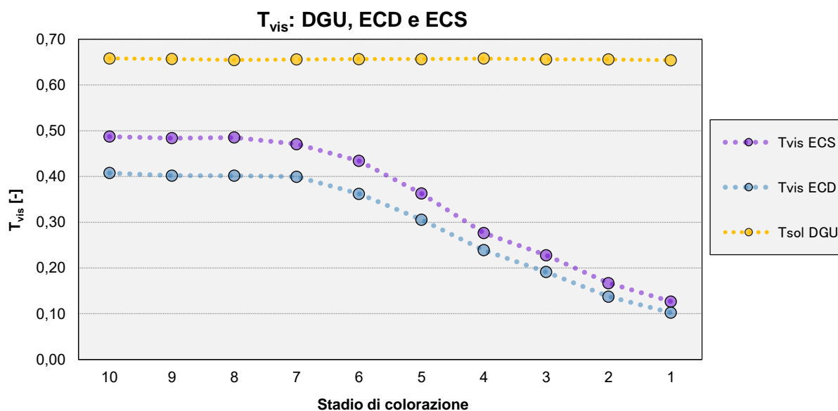
Figura 12. Trasmissione visibile del vetro chiaro e del vetro elettrocromico nei 10 stati di colorazione.
