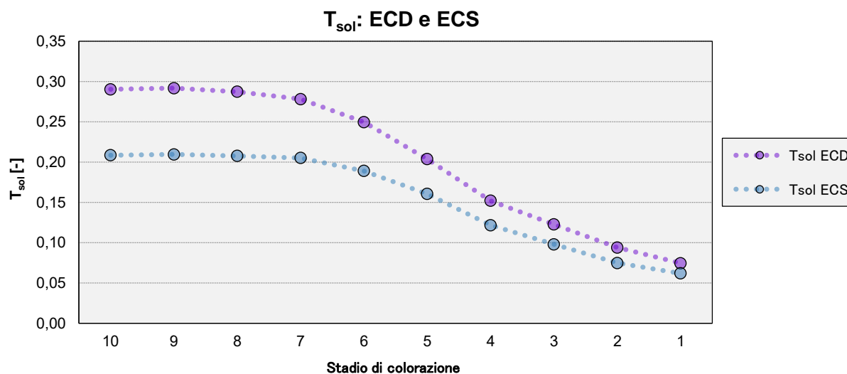
Figura 10. Trasmissione solare media del vetro elettrocromico per i 10 stadi di colorazione.
