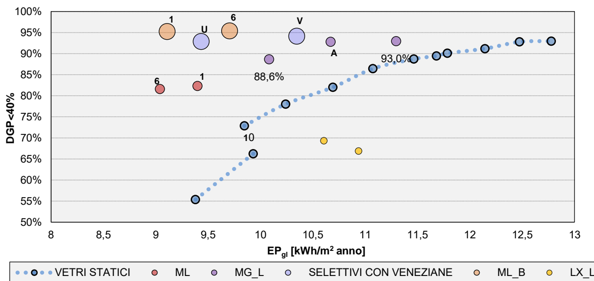
Figura 20. Correlazione di EP_{GL} e DGP < 40\% per le strategie di controllo esaminate nel clima di Torino.
