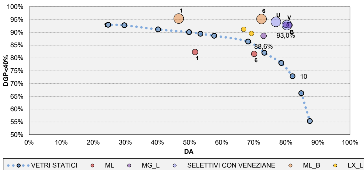
Figura 19. Correlazione di DA e DGP < 40\% per le strategie di controllo esaminate nel clima di Torino.
