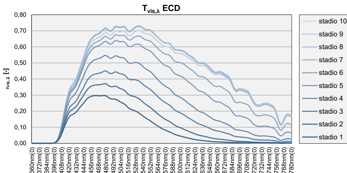
Figura 11. Trasmissione luminosa per lunghezza d'onda per vetro elettrocromico per i 10 stati di colorazione del vetro elettrocromico.
