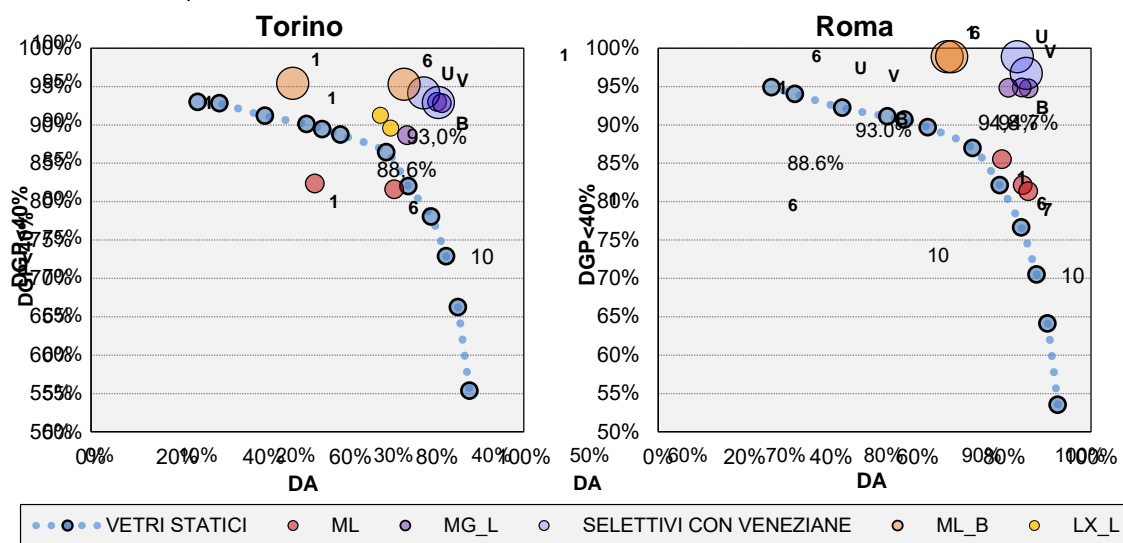
Figura 29. Correlazione di DA e DGP < 40\% per le strategie di controllo esaminate nei climi di Torino e Roma.
