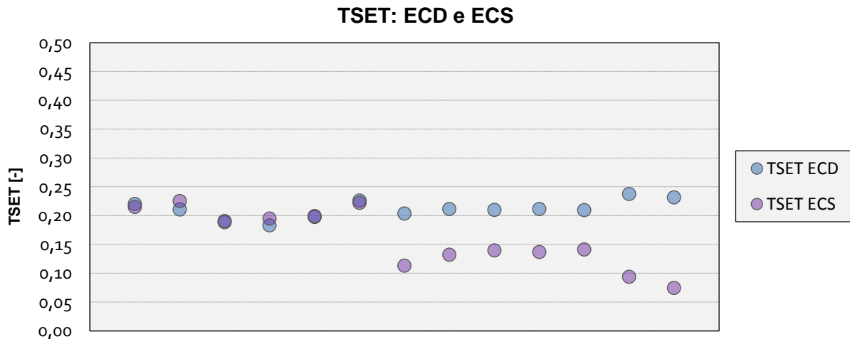
Figura 8. Fattore solare equivalente per tre diversi stati di colorazione.
