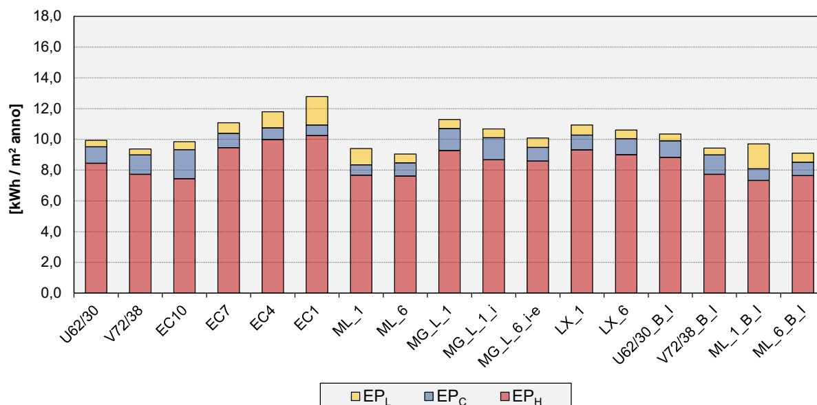
Figura 17. Indice di prestazione energetica per riscaldamento, raffrescamento ed illuminazione per i vetri statici e le strategie di controllo investigate per il clima di Torino.
