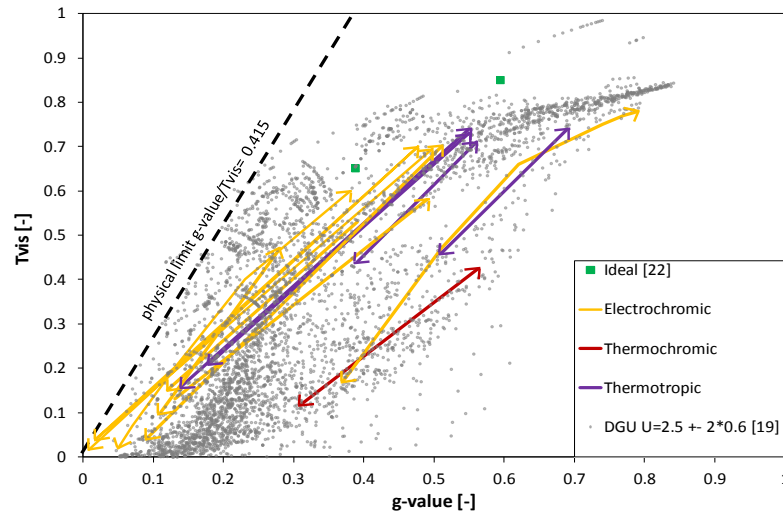
Figura 1. T_{vis} e g-value di vetri dinamici attivi e passivi (attualmente sul mercato) confrontato con diverse configurazioni di vetri camera tradizionali [12].
