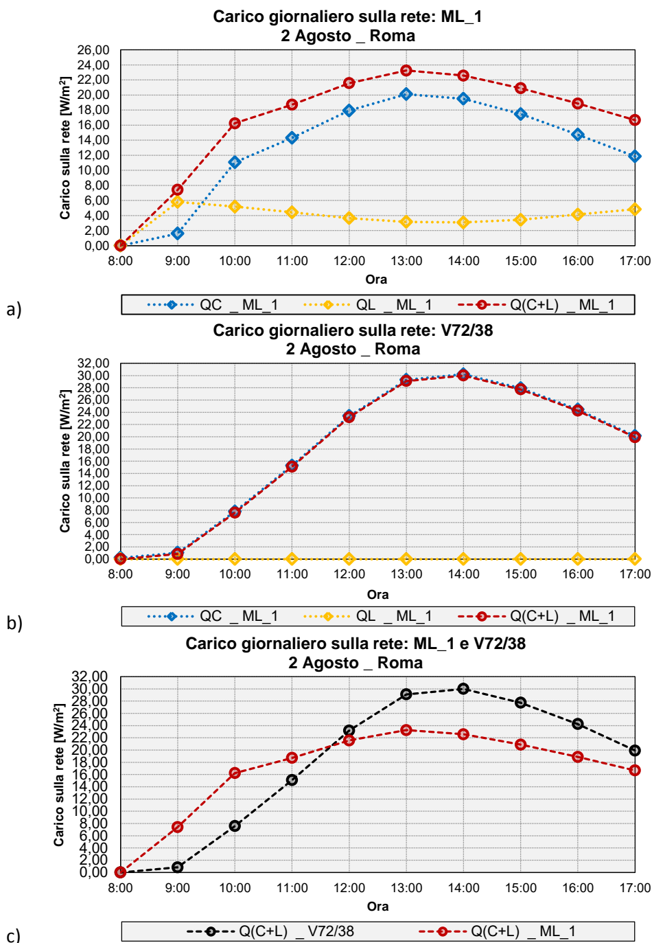
Figura 31. Carico giornaliero sulla rete elettrica al 2 Agosto nel clima di Roma per la strategia di controllo a) ML_1, b) il vetro selettivo dalle prestazioni standard (V72/30) e c) confronto tra i carichi totali relativi a questi due casi.
