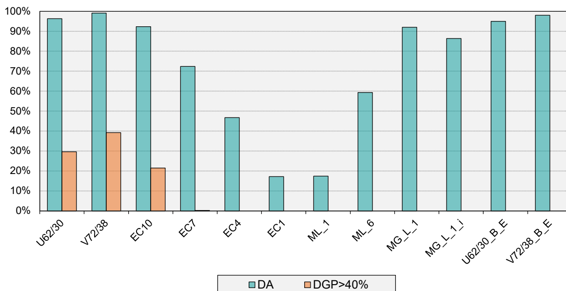
Figura 26. Daylight Autonomy (DA) e Daylight Glare probability (DGP) ottenuti per i vetri statici e le strategie di controllo investigate per il clima di Abu Dhabi.
