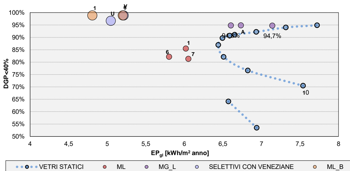
Figura 24. Correlazione di EP GL e DGP<40% per le strategie di controllo esaminate nel clima di Roma,
