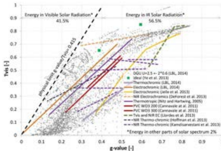
Figura 2. T_{vis} e g-value di vetri dinamici attivi e passivi attualmente sul mercato (linea continua) e innovativi (linea tratteggiata) confrontato con diverse configurazioni di vetri camera tradizionali [13].
