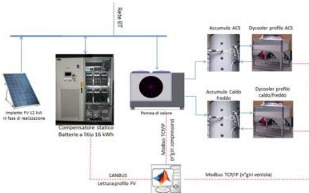
Figura 1: schema impianto ibrido sperimentale installato presso il C.R ENEA Casaccia
