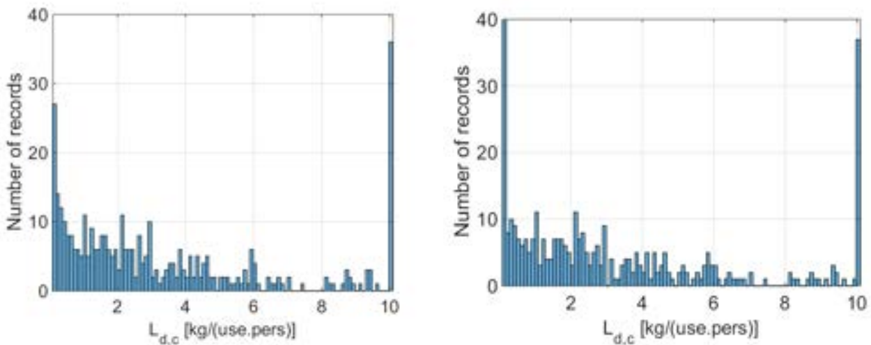
Figura 6. Ottimizzazione della massa equivalente per ciclo di cottura con i fornelli elettrici. Ottimizzazione con ModeFRONTIER (a sinistra) e con il modello Matlab (a destra)
