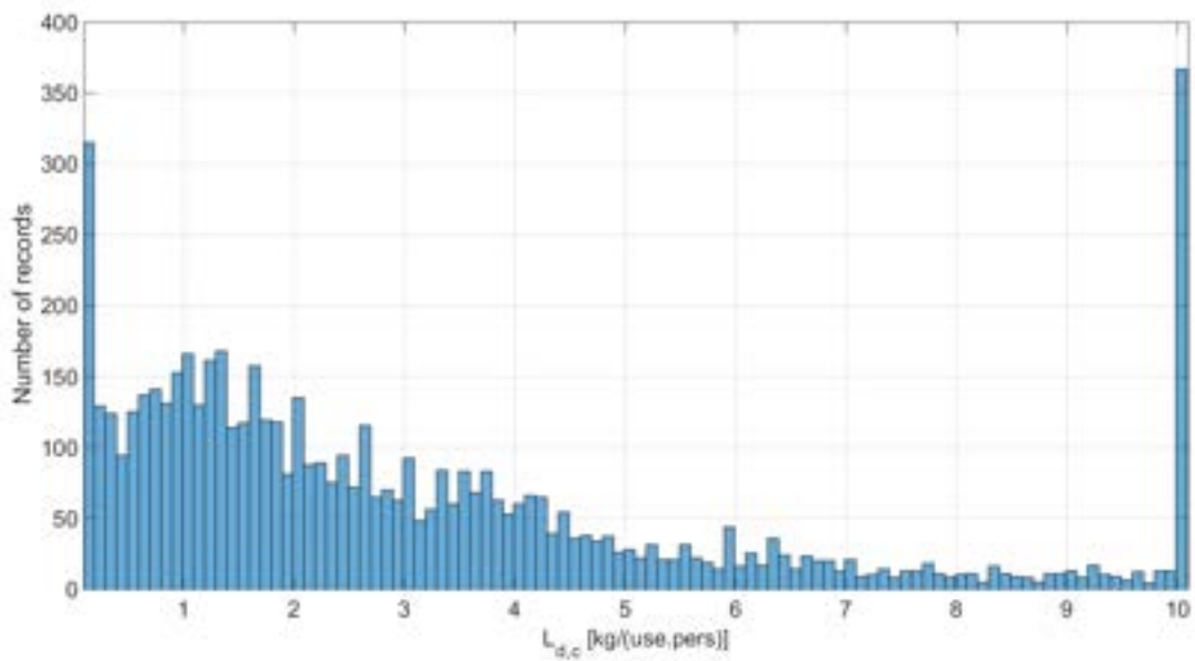
Figura 4. Distribuzione della massa equivalente per ciclo preparata con i piani cottura
