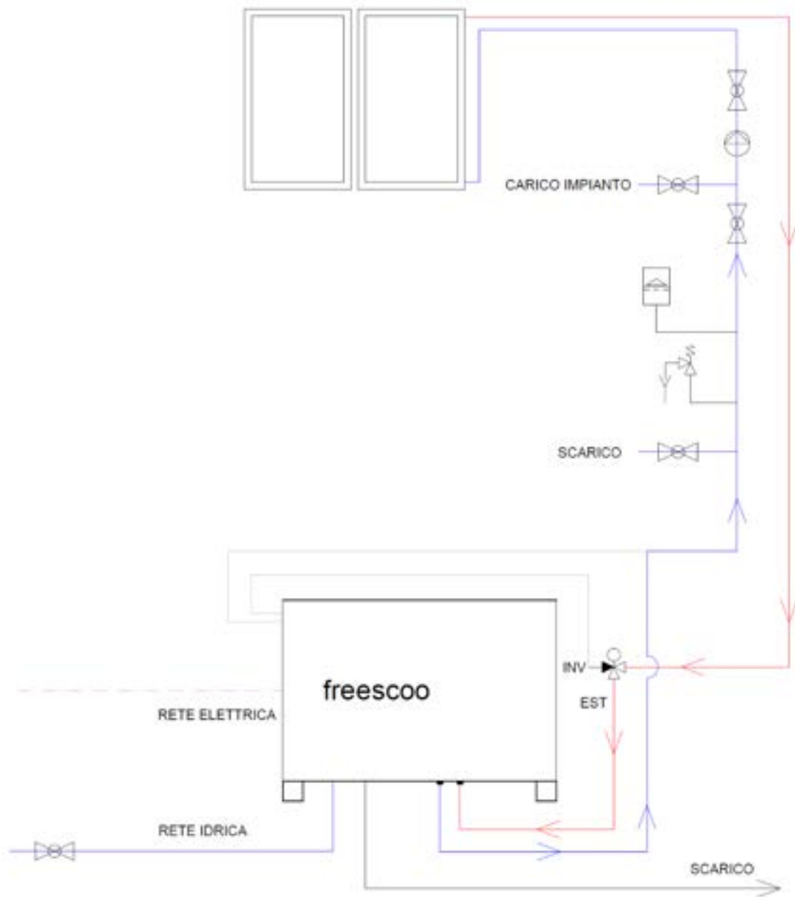
Figura 8: Schema impiantistico per l'allacciamento del sistema di climatizzazione all'impianto solare termico
