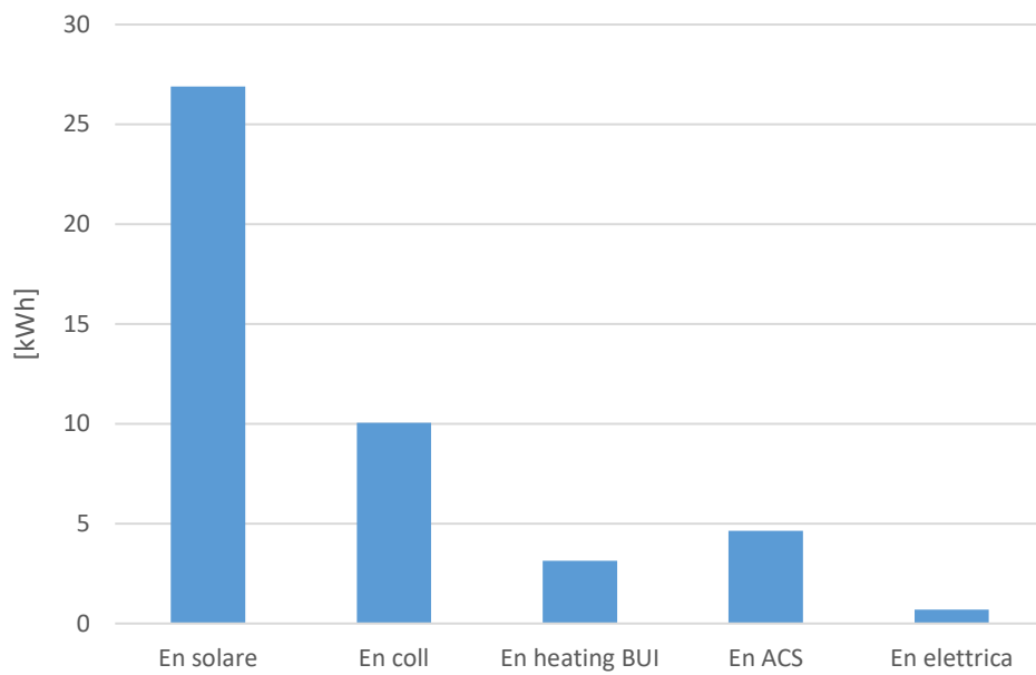
Figura 22: Risultati energetici – 20 Dicembre 2018
