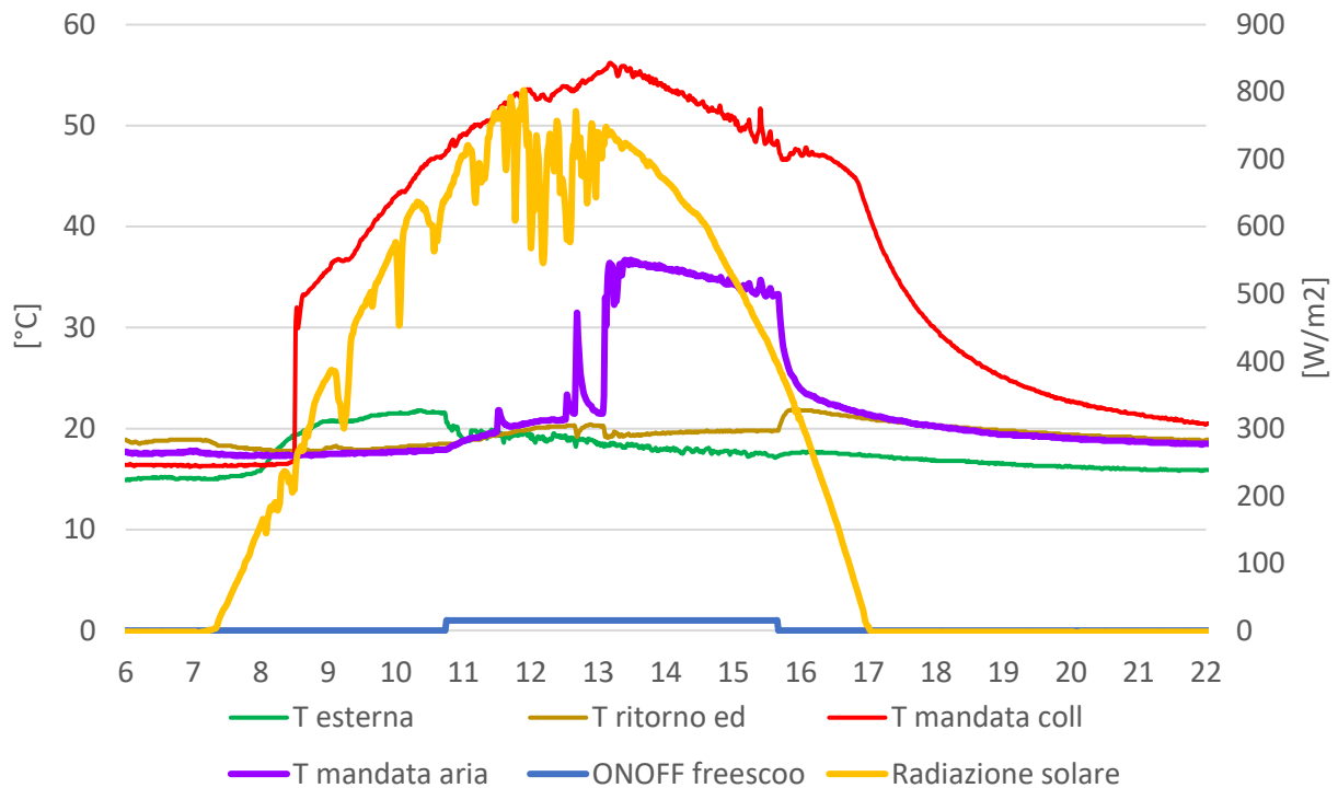
Figura 18: Temperature ACS – 20 Dicembre 2018
