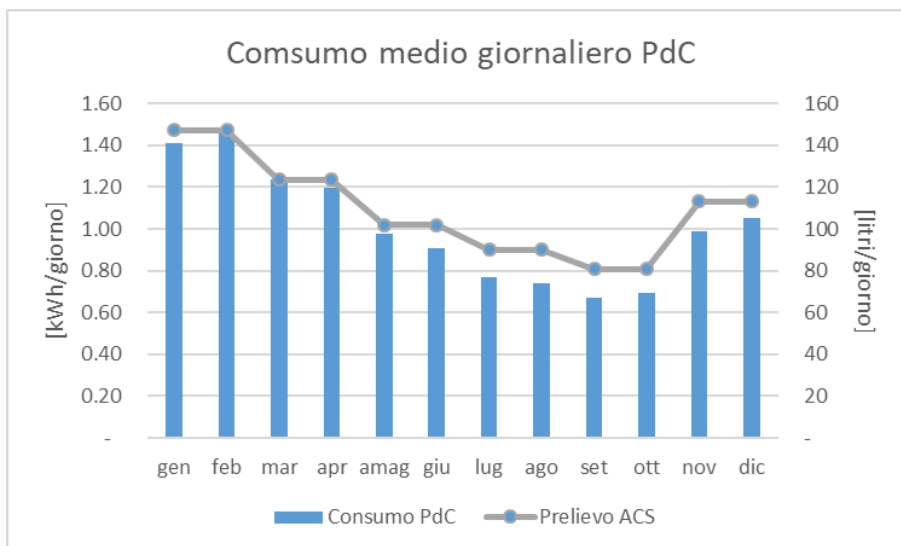
Figura 36 Consumi giornalieri della Pompa di Calore per ACS
