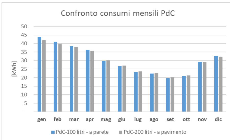
Figura 35 Confronto fra i consumi elettrici per la produzione di ACS fra le due tecnologie di PdC proposte
