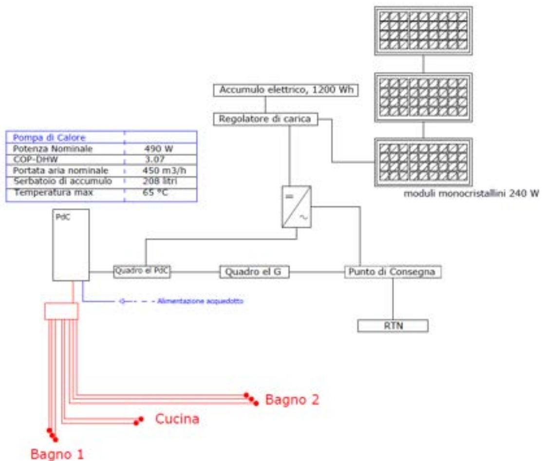
Figura 50 Layout di impianto per l'utenza analizzata
