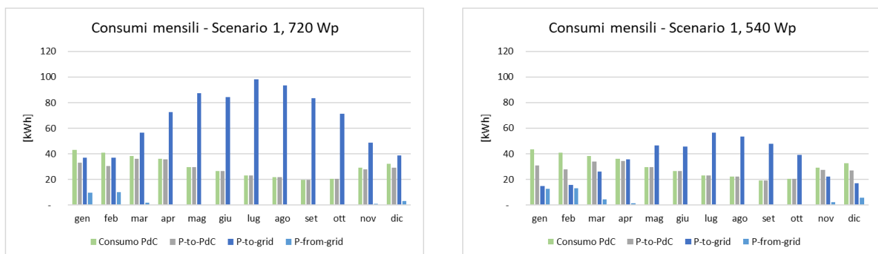
Figura 38 Risultati in condizioni di funzionamento standard al variare della potenza fotovoltaica installata
