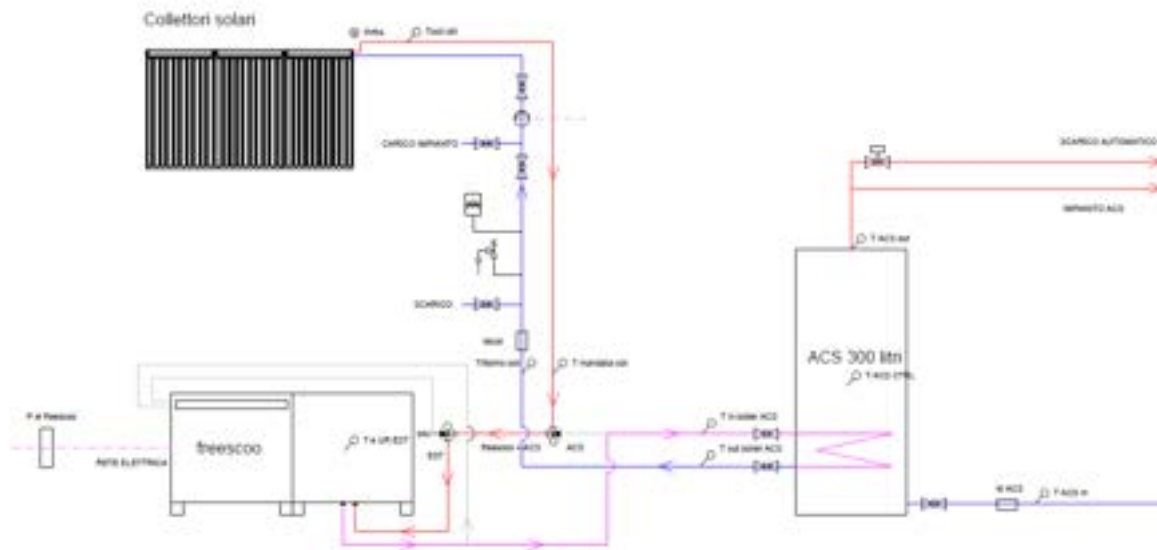
Figura 13: Schema impiantistico del sistema freescoo installato presso il centro ENEA al faro di Grecale a Lampedusa
