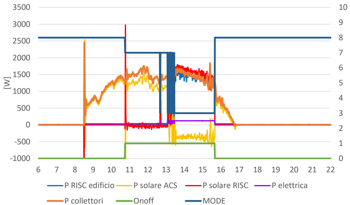
Figura 19: Potenze e modalità di funzionamento – 20 Dicembre 2018
