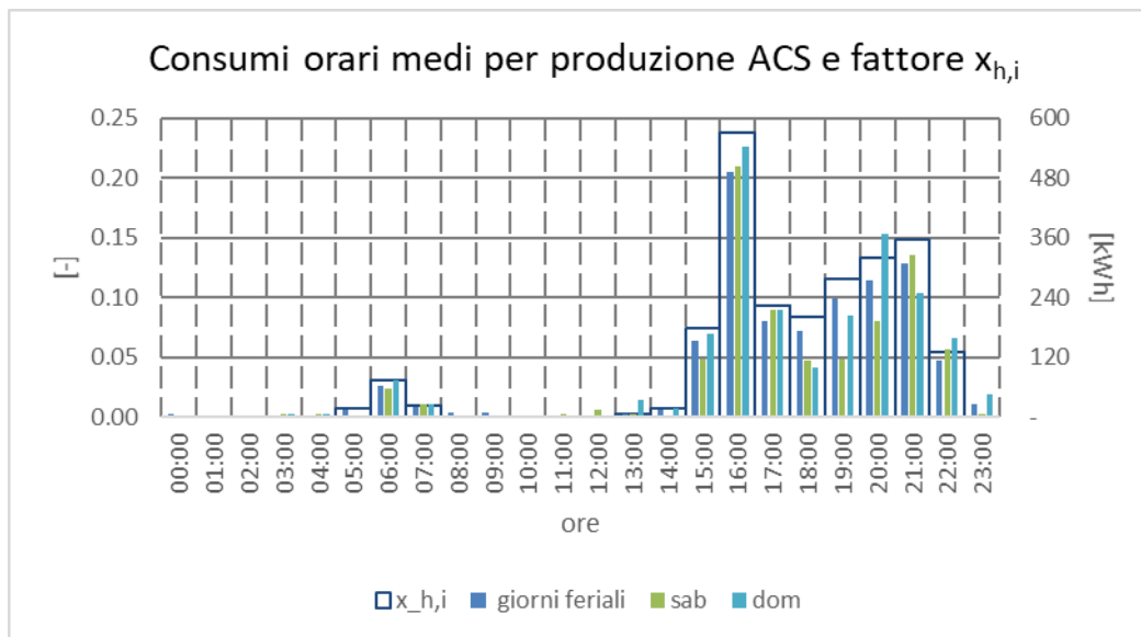
Figura 32 Consumi scaldacqua monitorati e curva oraria di prelievo
