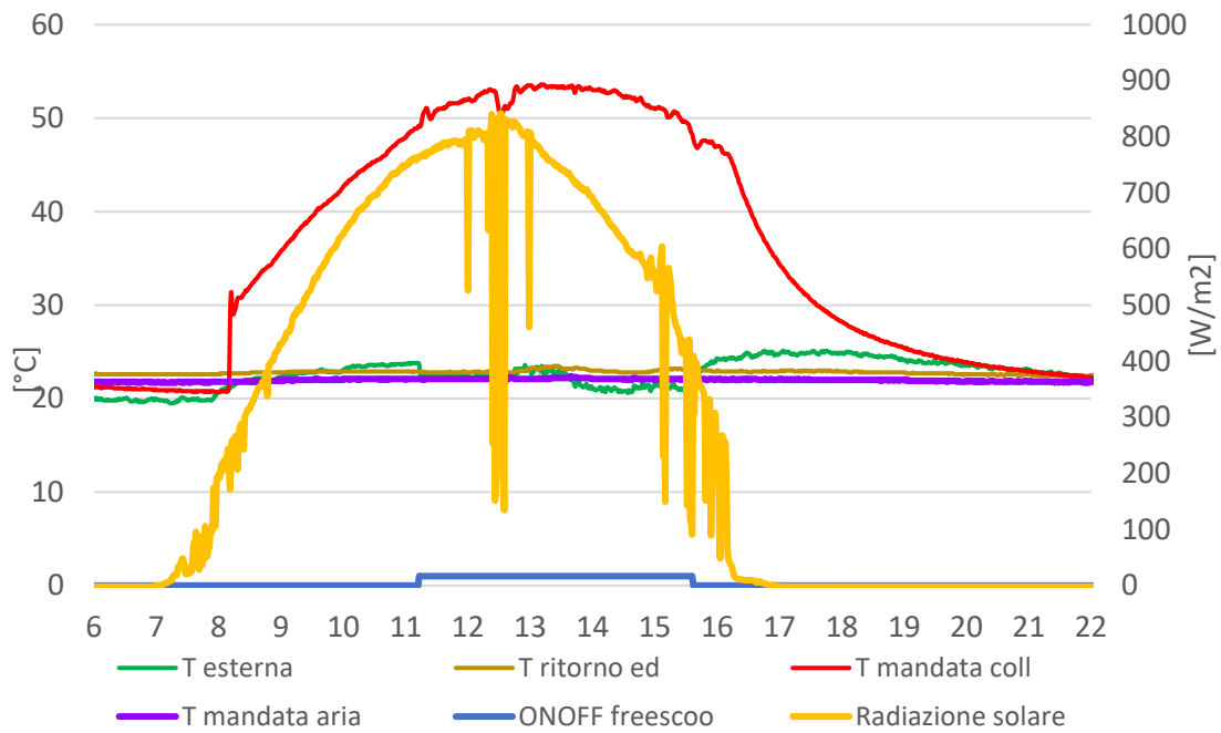
Figura 14: Temperature registrate - 25 Novembre 2018
