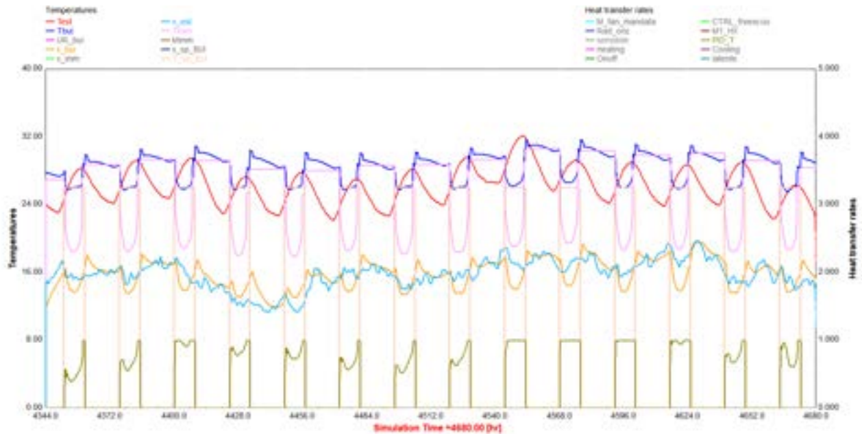
Figura 11: Andamento delle condizioni dell'aria nel locale climatizzato per le prime due settimane di luglio
