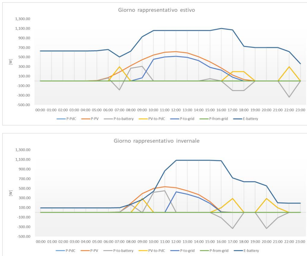
Figura 45 Funzionamento standard dell'impianto nei giorni rappresentativi
