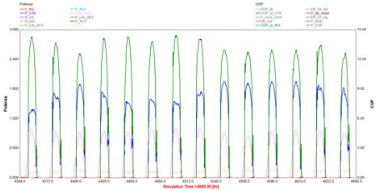
Figura 12: Andamento della potenza frigorifera (blu), EER (verde) e radiazione solare (rosa) per le prime due settimane di luglio
