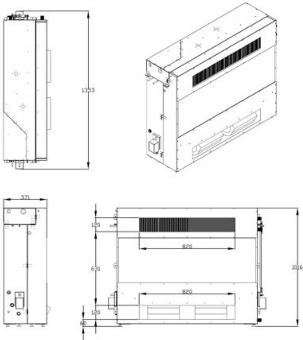
Figura 9: Disegni dell'unità di climatizzazione solare
