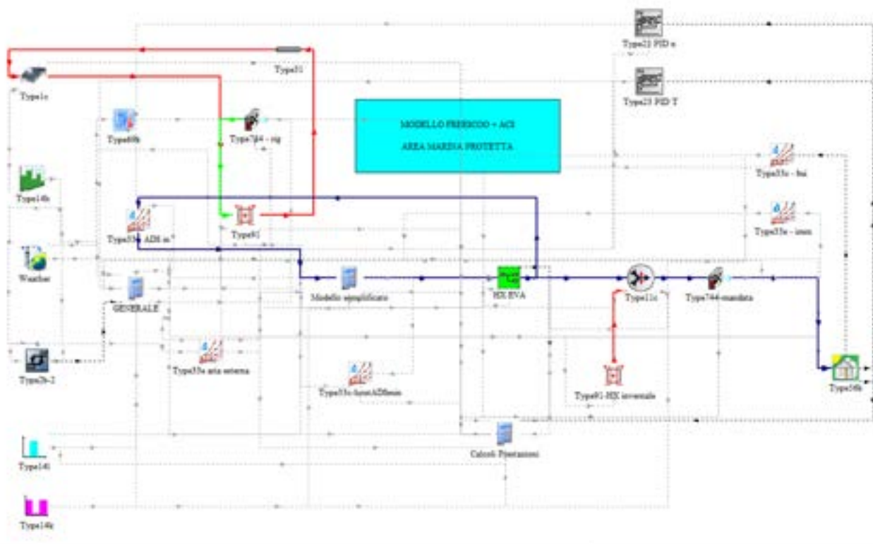
Figura 10: Progetto TRNSYS utilizzato per la simulazione del sistema edificio – impianto
