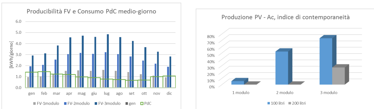
Figura 37 Analisi produzione fotovoltaica sulla base dei dati climatici orari dell'isola (fonte Meteonorm)
