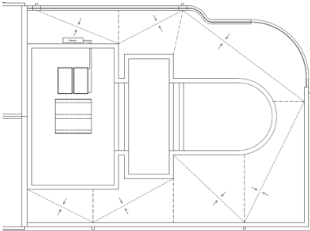
Figura 5: Pianta della copertura con i collettori solari
