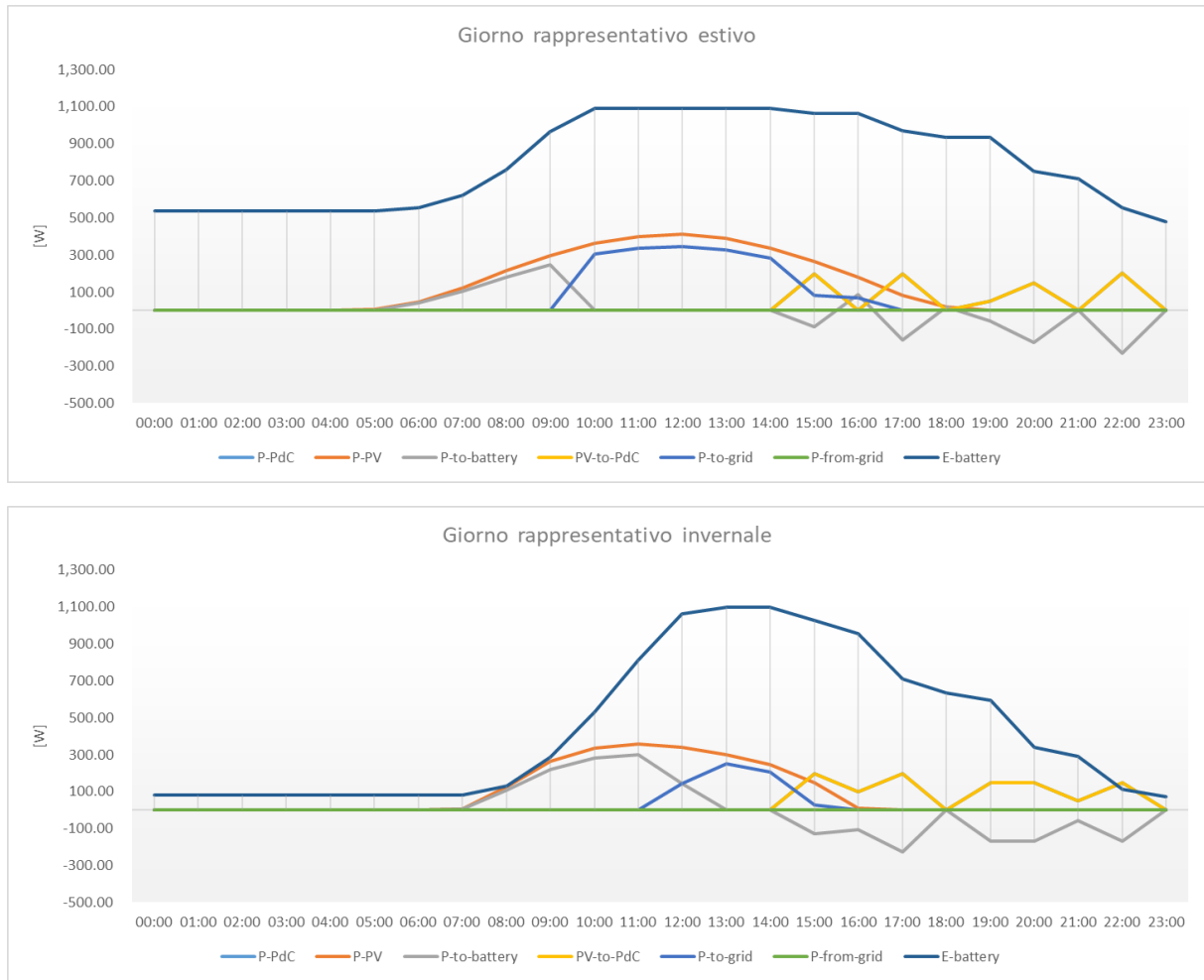
Figura 39 Funzionamento dell'impianto da 540 W nei giorni rappresentativi
