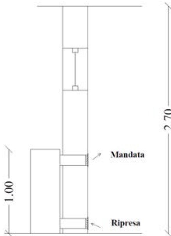
Figura 7: Posizionamento dell'unità freesco e sezione della parete Sud
