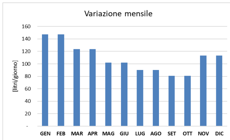
Figura 33 Consumi giornalieri di ACS al variare del mese
