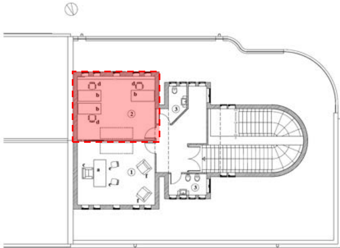
Figura 2 Pianta dell'edificio e del locale scelto per l'installazione del sistema freesco (tratteggiato in rosso)
