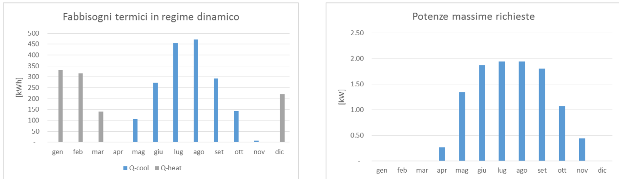
Figura 3 Risultati della simulazione in regime dinamico.
