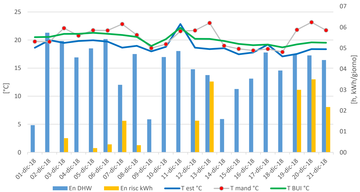
Figura 26 Temperature e produzione di calore solare per ACS e riscaldamento – dicembre 2018
