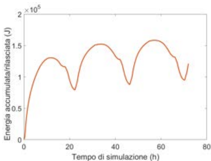
Figura 12. Energia accumulata/rilasciata dal modulo di PCM: Caso base.
