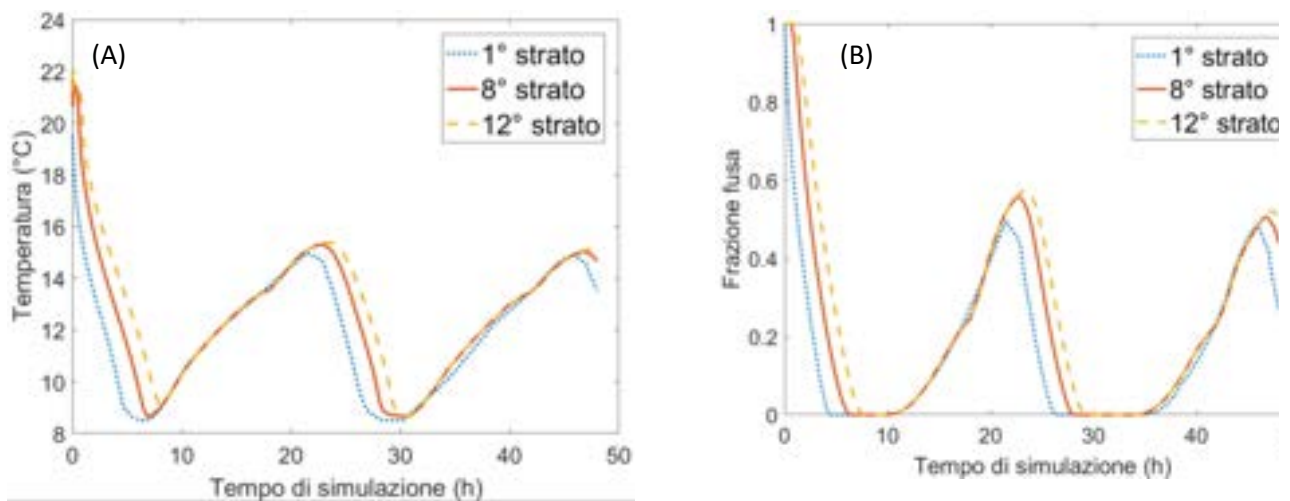
Figura 10. (A) Temperatura nel PCM, (B) Frazione fusa del PCM: Caso 3.
