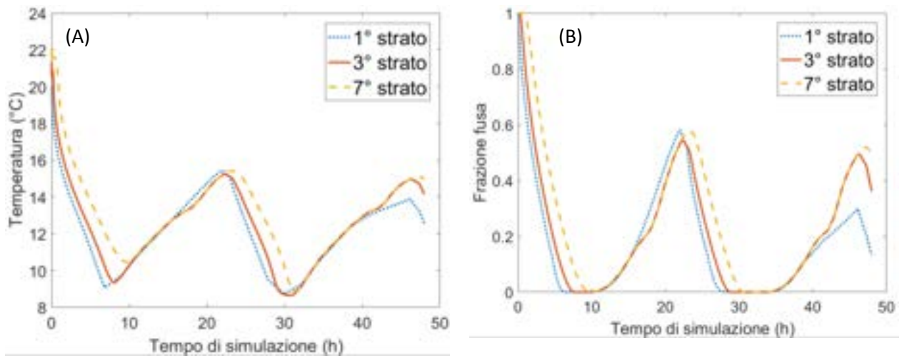
Figura 9. (A) Temperatura nel PCM, (B) Frazione fusa del PCM: Caso 2.
