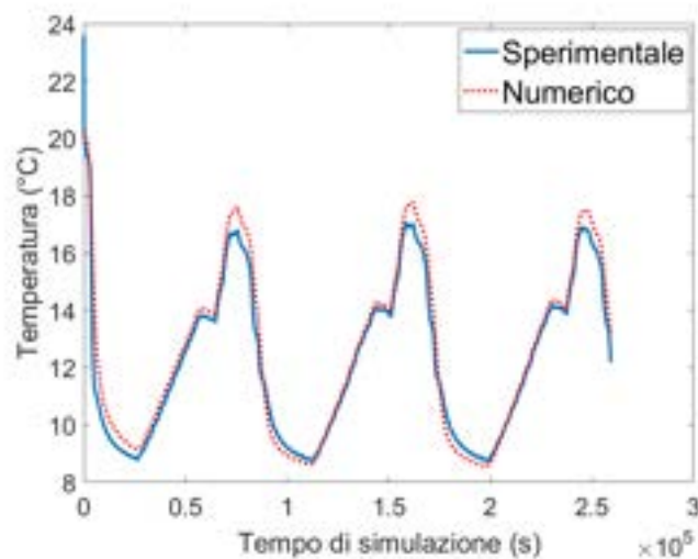
Figura 17. Confronto tra i risultati numerici e sperimentali relativamente alla simulazione del caso base.
