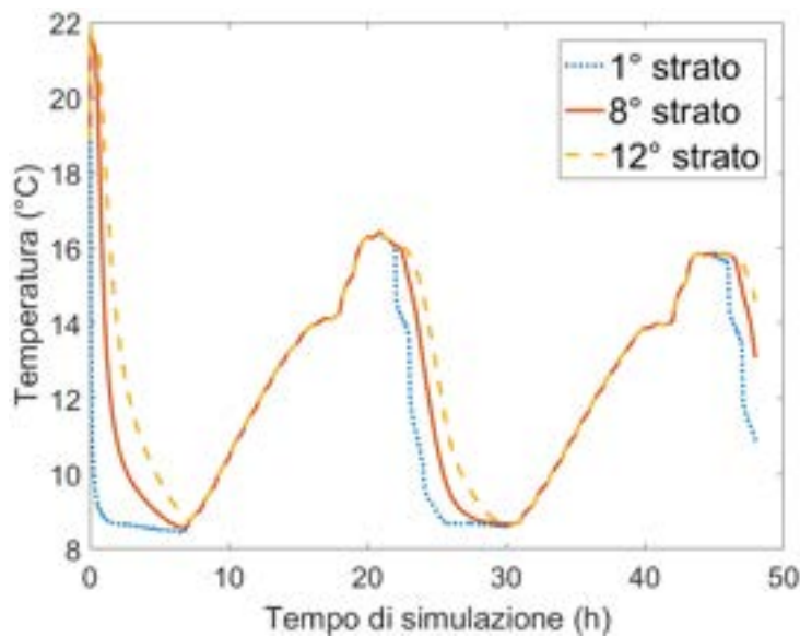
Figura 5. Temperatura dell'acqua nel serbatoio: Caso 3 ( V_{\text{cont}} = 1/10 L).
