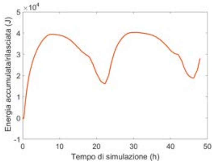
Figura 14. Energia accumulata/riasciata dal modulo di PCM: Caso 2.
