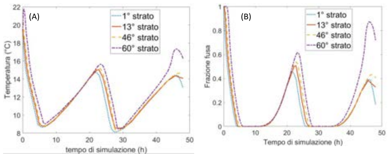
Figura 11. (A) Temperatura nel PCM, (B) Frazione fusa del PCM: Caso 4.
