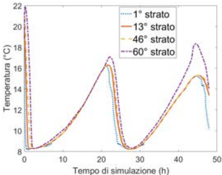
Figura 6. Temperatura dell'acqua nel serbatoio: Caso 4 ( V_{\text{cont}} = 1/636,6 L).
