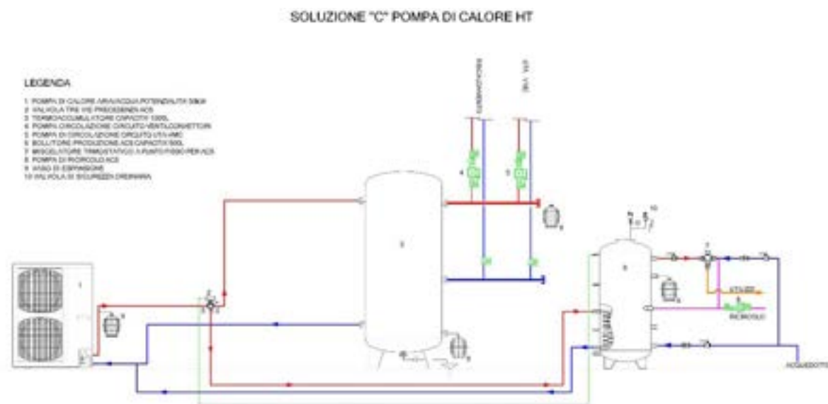
Figura 10 - Schema funzionale impianto di riscaldamento e produzione di ACS ipotizzato per lo scenario con pompa di calore ad alta temperatura.
