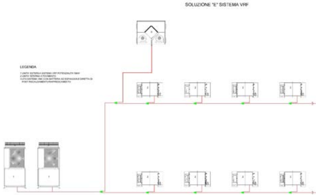
Figura 12 - Schema funzionale impianto di riscaldamento ipotizzato per lo scenario sistema di riscaldamento VRF.
