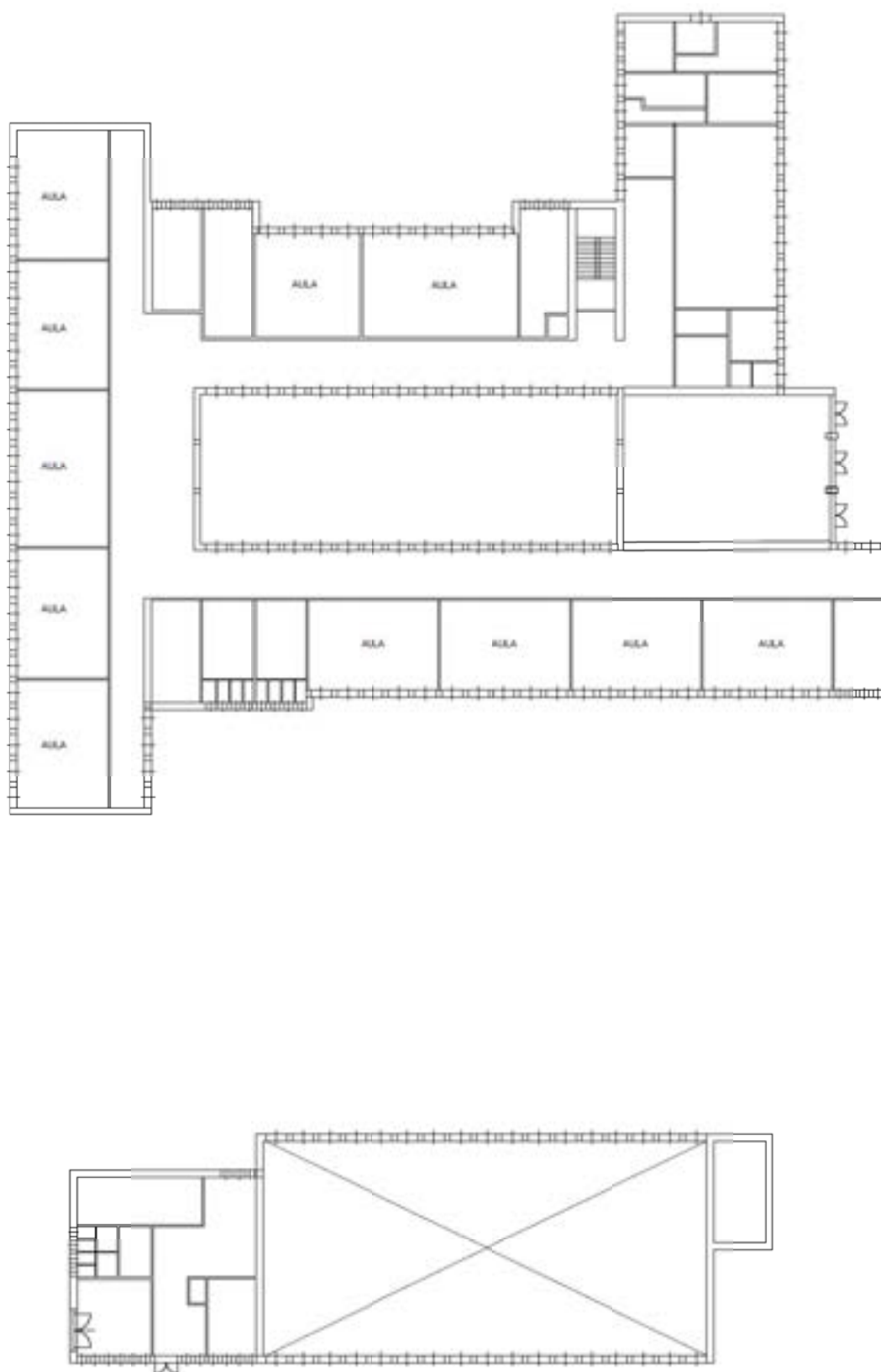
Figura B19 - Edificio 3 – Pianta piano terra.
