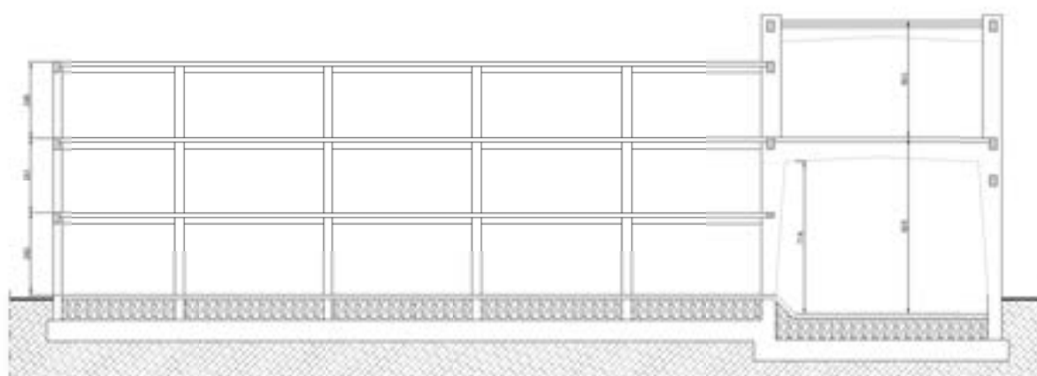
Figura B17 - Edificio 2 - Sezione B-B'.
