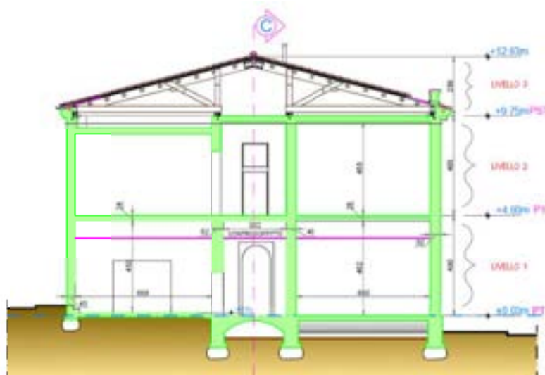
Figura B7 - Edificio 1 - Sezione A-A'.
