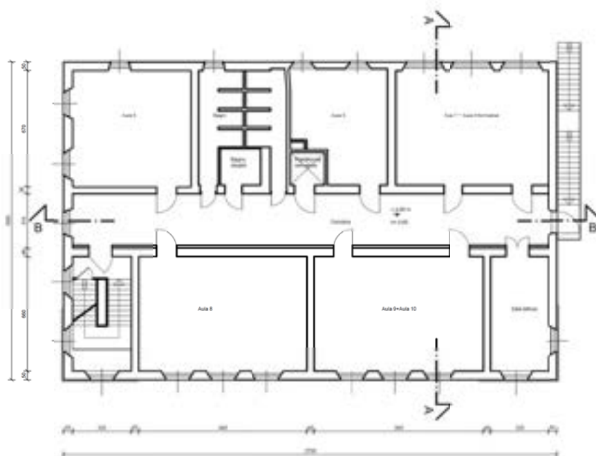
Figura B2 - Edificio 1 - Pianta piano primo.
