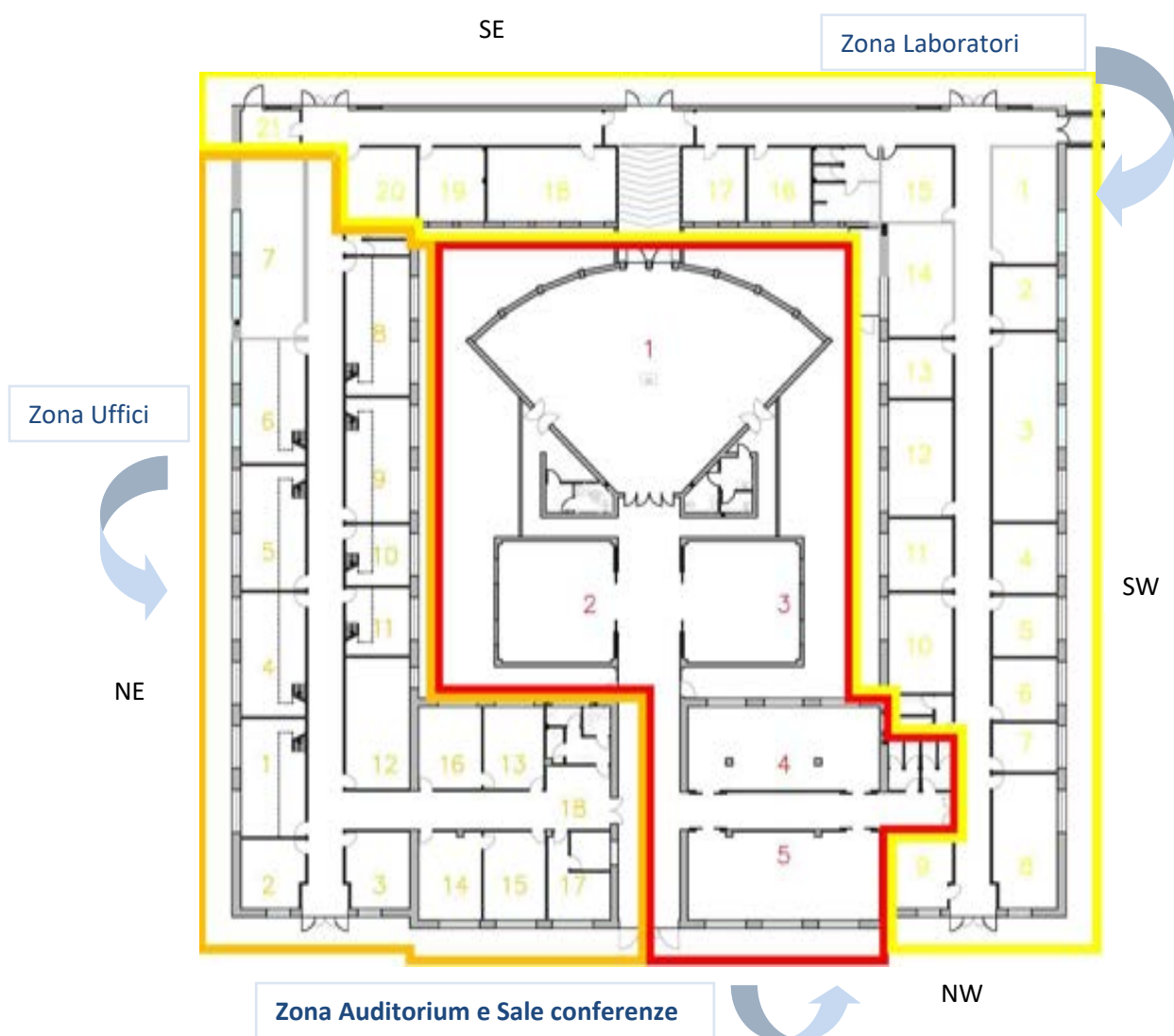
Figura 3 Planimetria generale
