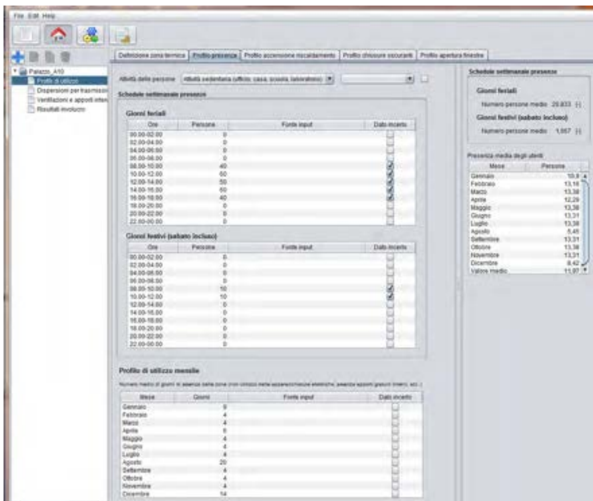
Figura 17: Profili di utilizzo di Palazzo A10 da parte degli utenti, schermata dei dati inseriti in SEAS.
