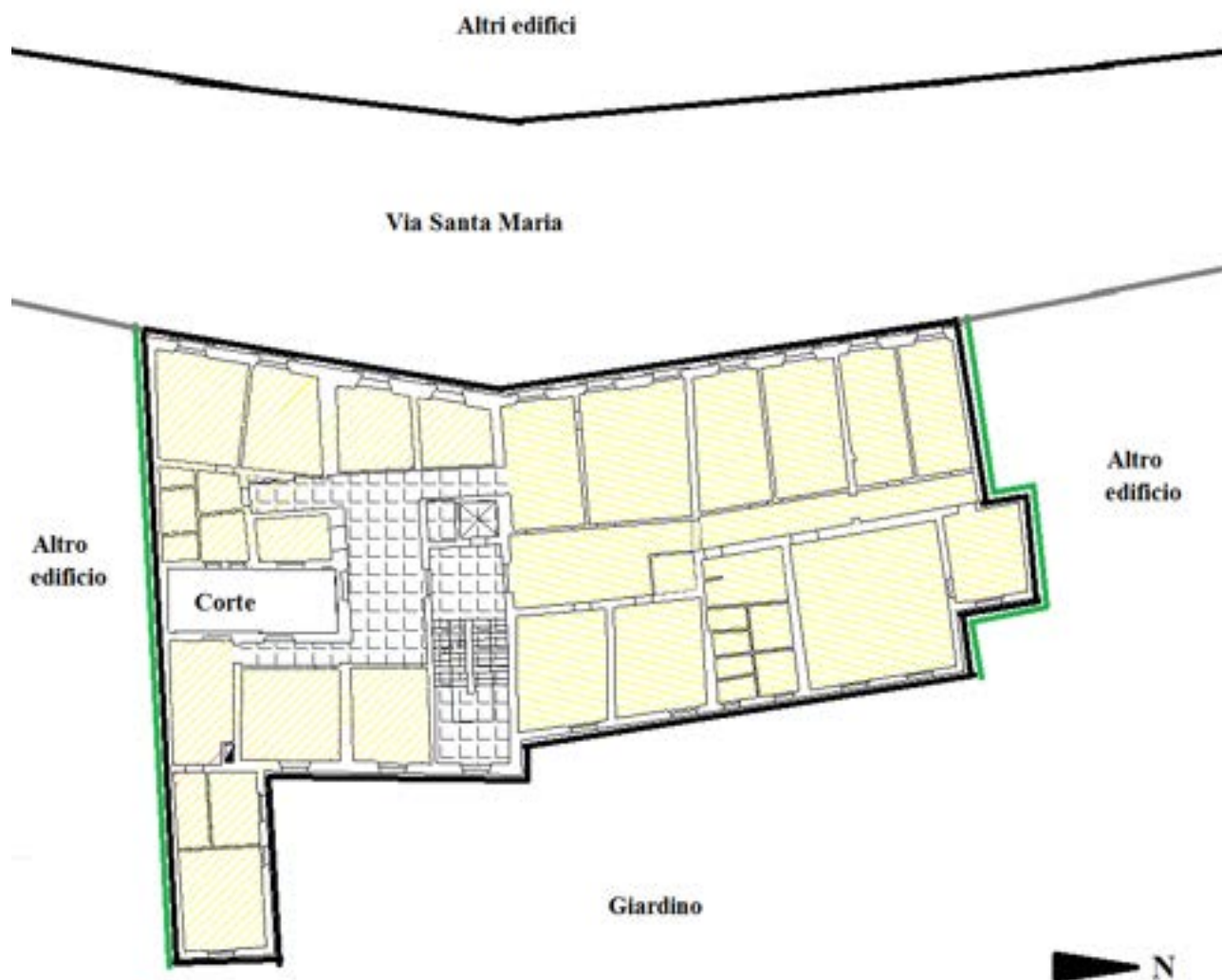
Figura 15: Pianta del secondo piano di Palazzo A10. In giallo è evidenziata le aree oggetto di analisi. I confini verdi indicano le pareti adiabatiche verso altri edifici.
