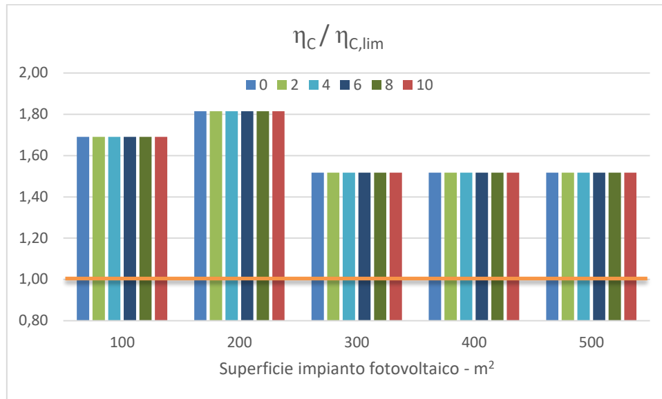
Figura 37: Rapporto tra il valore effettivo e limite del parametro \eta_c al variare della temperatura di switch invernale e della superficie di captazione solare del sistema fotovoltaico. Soddissano i requisiti NZEB le soluzioni impiantistiche con valore superiore all'unità.
