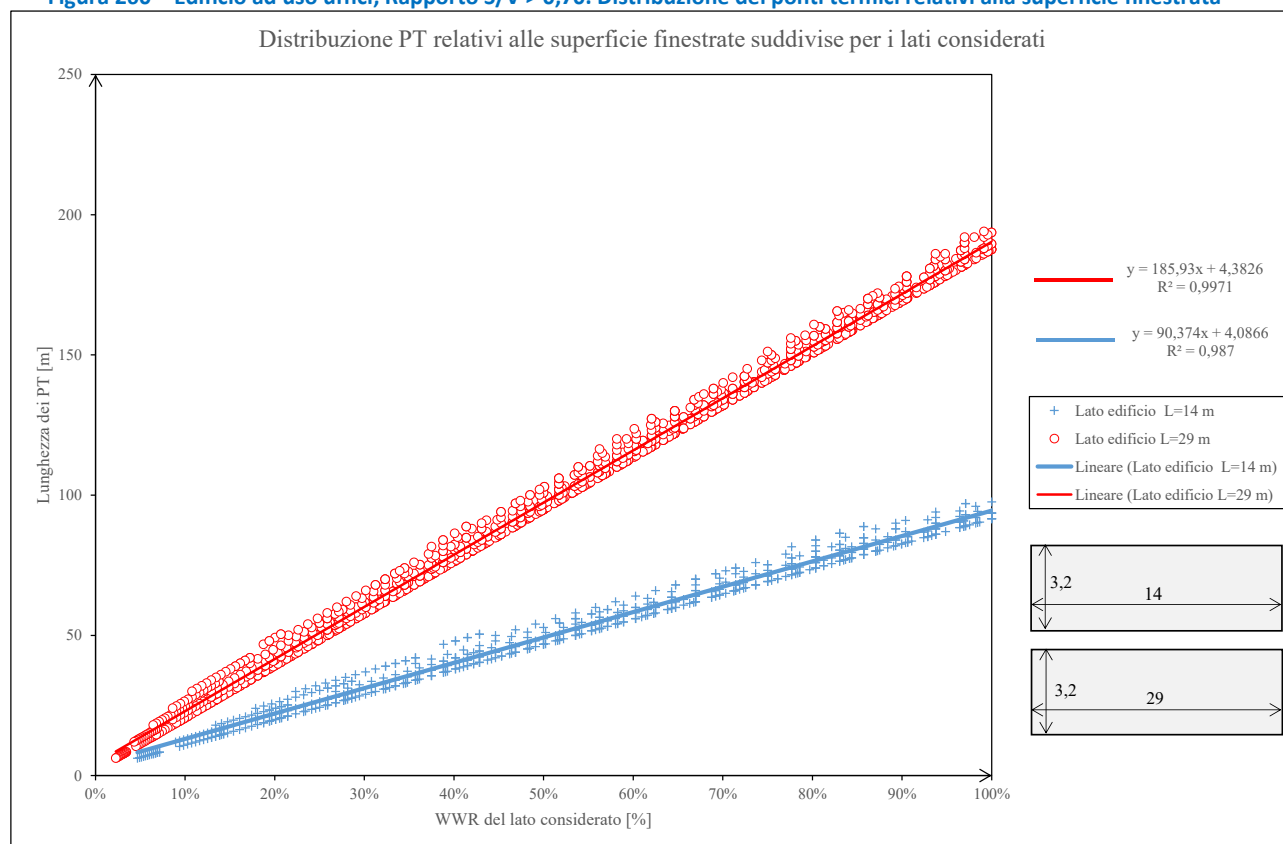
Figura 260 – Edificio ad uso uffici, Rapporto S/V > 0,70. Distribuzione dei ponti termici relativi alla superficie finestrata
