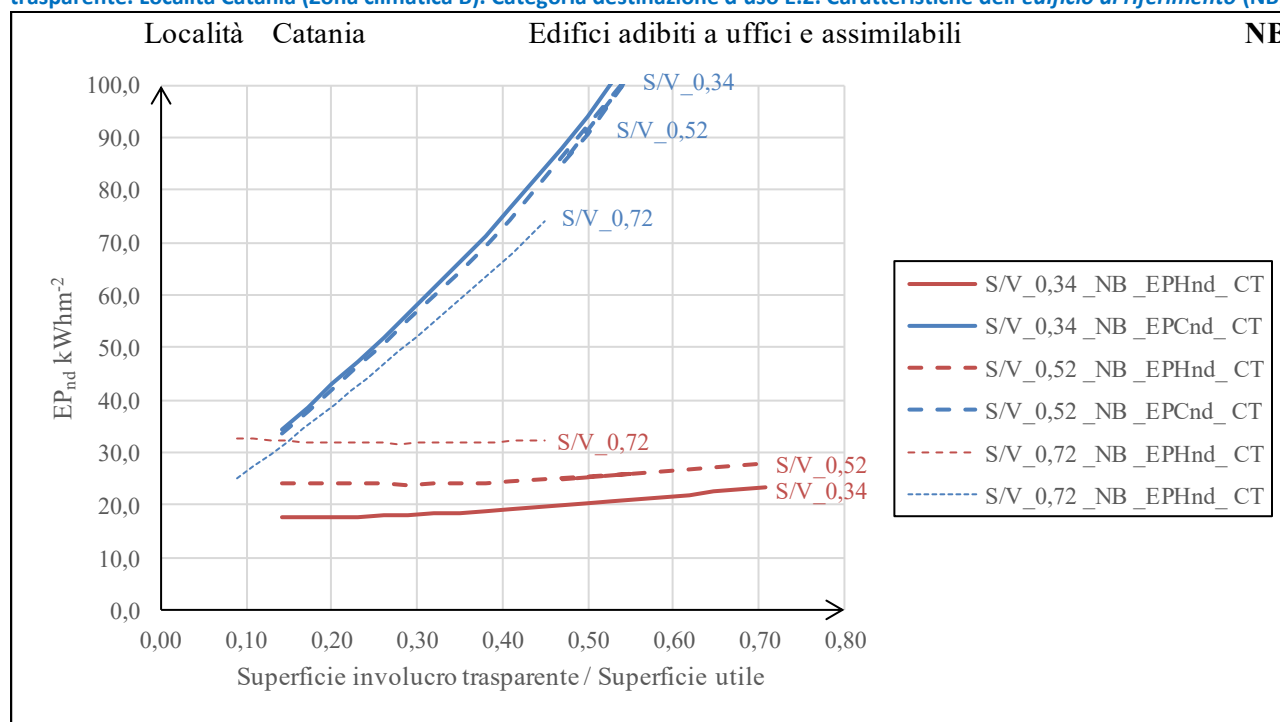
Figura 19 – Prestazioni energetiche degli edifici analizzati al variare del rapporto di forma S/V_L e della superficie dell'involucro trasparente. Località Catania (Zona climatica B). Categoria destinazione d'uso E.2. Caratteristiche dell'edificio di riferimento (NB).
