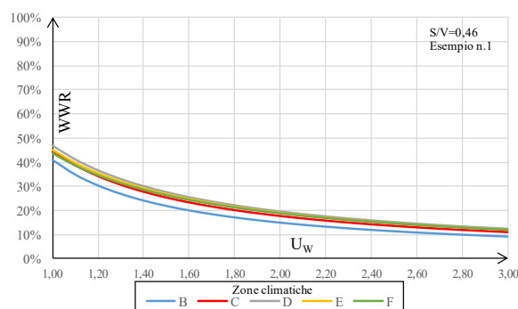
Figura 401 – Caso studio "Esempio n.1" – Variazione della superficie trasparente massima realizzabile (WWR) per un edificio con diverso rapporto di forma S/V=1 (sinistra) e S/V= 0,46 utilizzando le caratteristiche dell' edificio di riferimento (NB)
