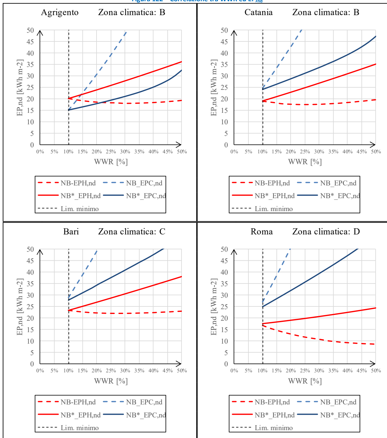
Figura 122 – Correlazione tra WWR ed EP_{nd}
