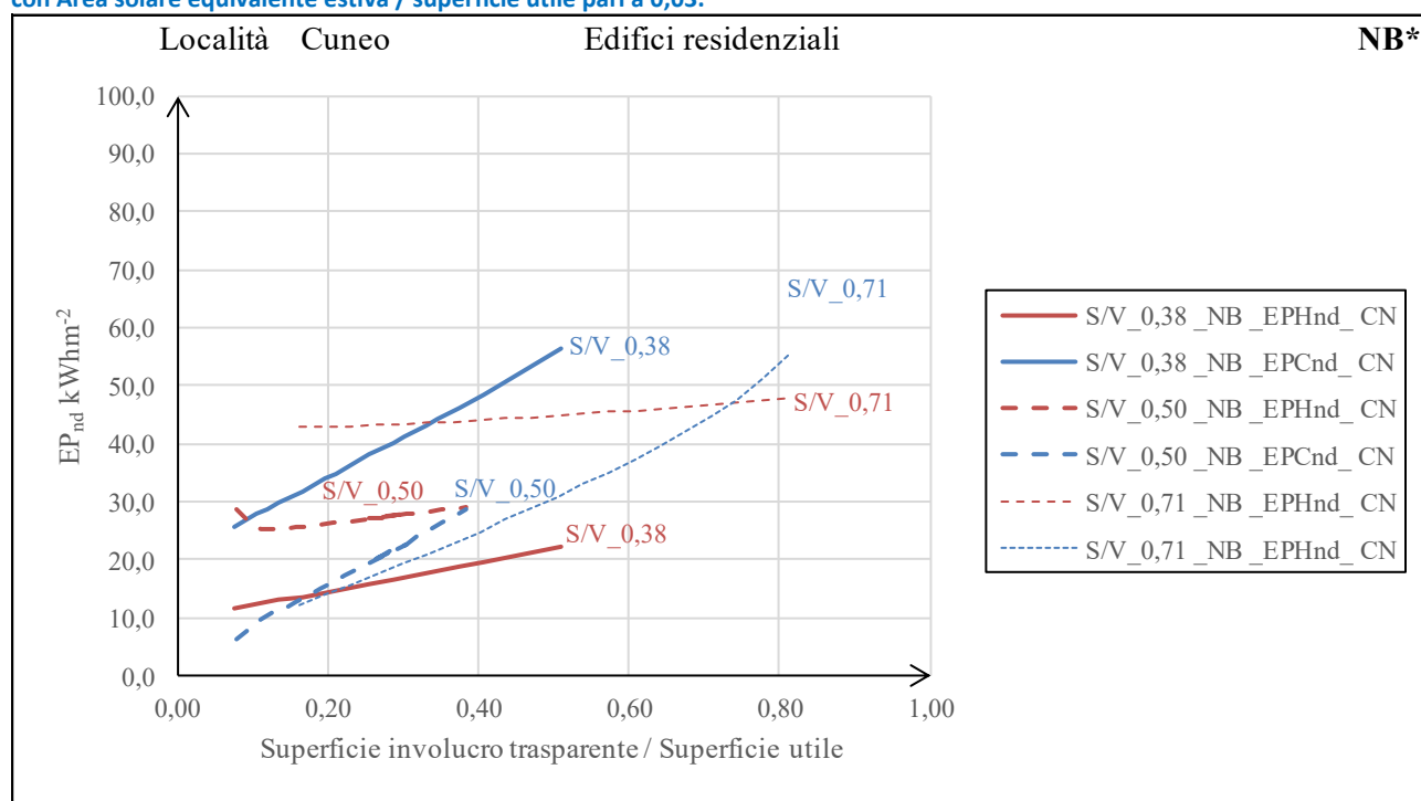
Figura 15 – Prestazioni energetiche degli edifici analizzati del rapporto di forma S/V_L e della superficie dell'involucro trasparente. Località Cuneo (Zona climatica F). Categoria destinazione d'uso E.1. Caratteristiche dell'edificio di riferimento (NB).
