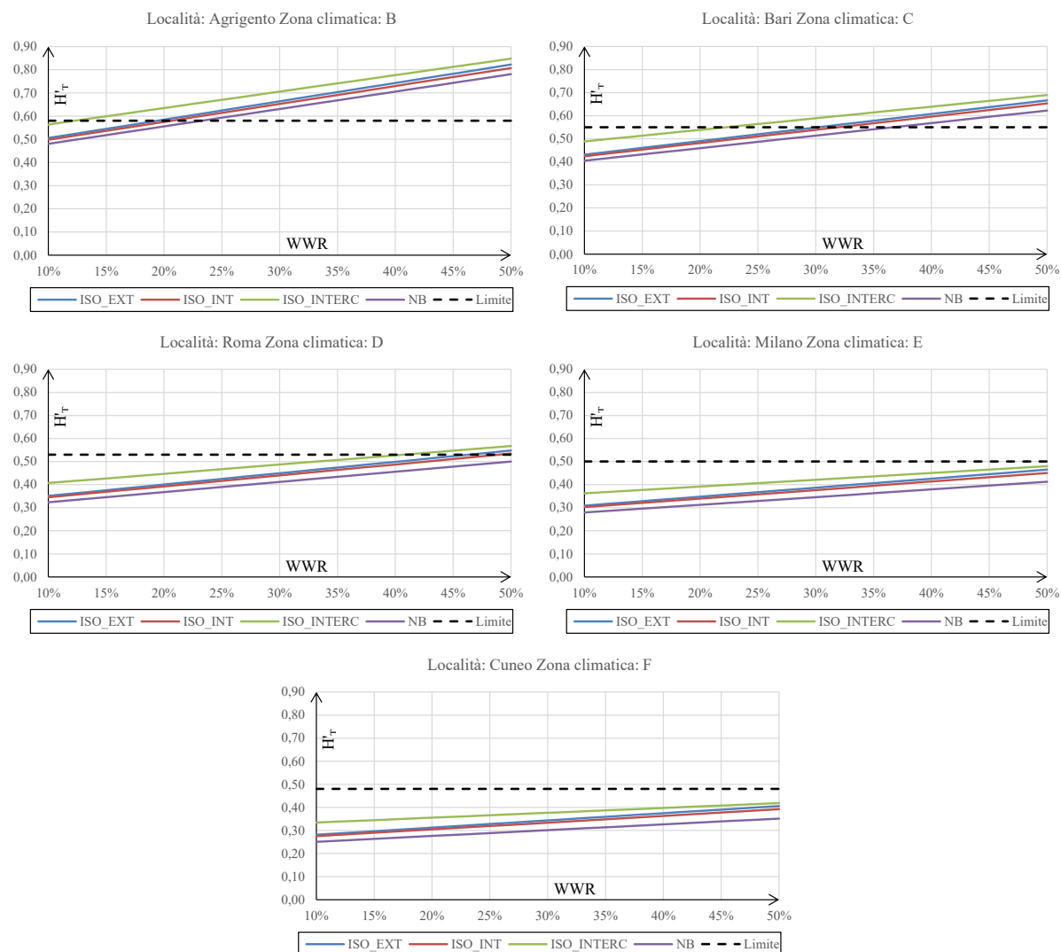
Figura 262 – Edificio ad uso uffici, Rapporto di forma S/V > 0,70. Correlazione tra WWR e parametro H'_{\tau}
