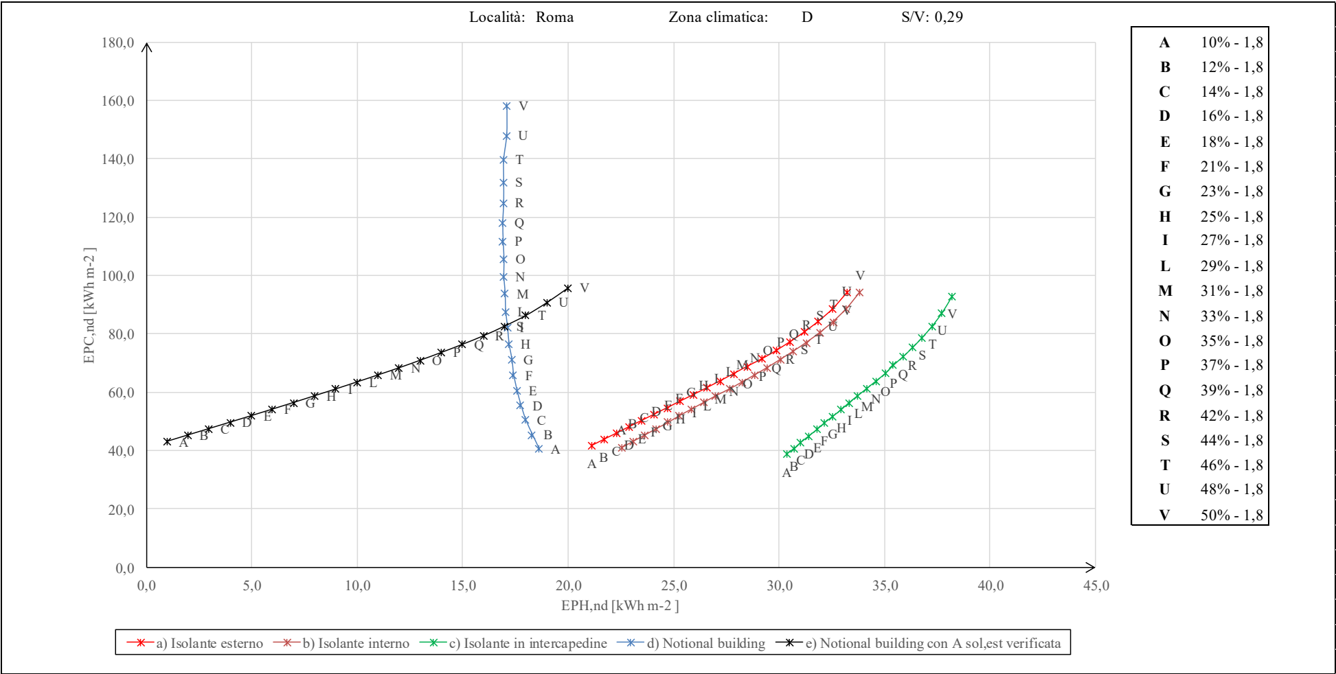
Figura 312 – Correlazione tra gli indici di prestazione energetica per un edificio adibito ad attività commerciali con rapporto di forma S/V < 0,40 . Località Roma (zona climatica D). Variazione dell'indice WWR
