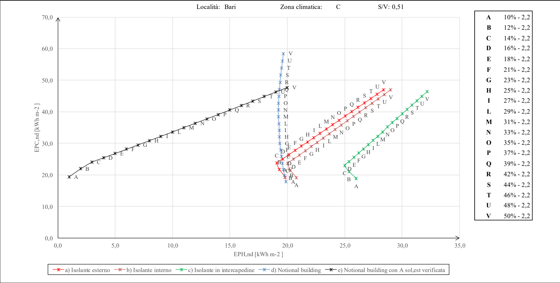
Figura 98 – Correlazione tra gli indici di prestazione energetica per un edificio residenziale con rapporto di forma 0,40 < S/V < 0,70 . Località Bari (zona climatica C). Variazione dell'indice WWR
