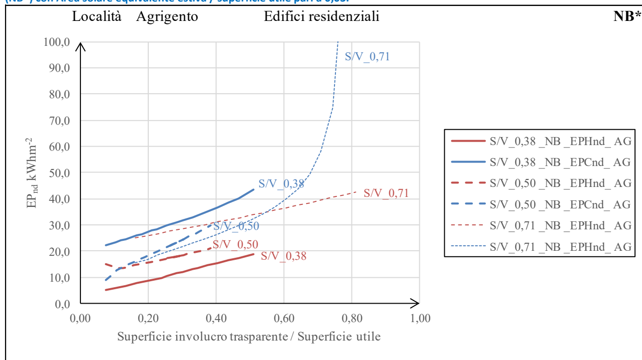
Figura 2 – Prestazioni energetiche degli edifici analizzati al variare del rapporto di forma S/V_L e della superficie dell'involucro trasparente. Località Agrigento (Zona climatica B). Categoria destinazione d'uso E.1. Caratteristiche dell'edificio di riferimento (NB*) con Area solare equivalente estiva / superficie utile pari a 0,03.
