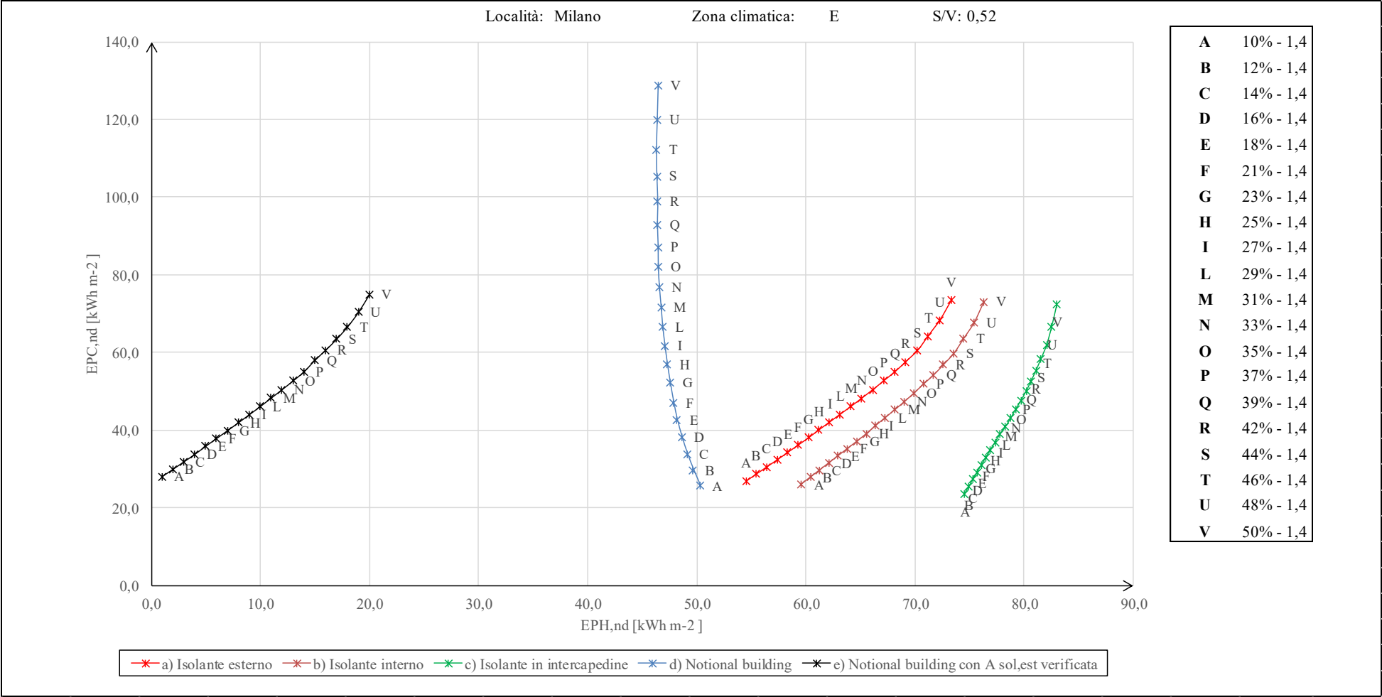
Figura 248 – Correlazione tra gli indici di prestazione energetica per un edificio ad uso uffici con rapporto di forma 0,40 < S/V < 0,70. Località Milano (zona climatica E). Variazione dell'indice WWR.
