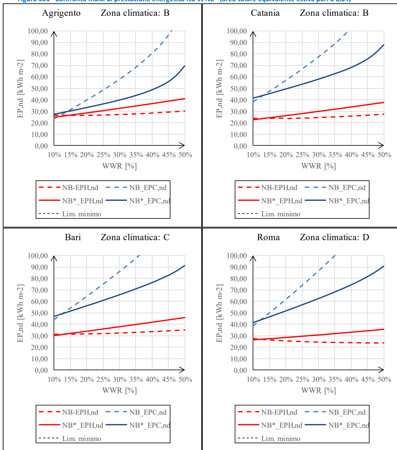
Figura 331 –Confronto indici di prestazione energetica NB vs NB* (area solare equivalente estiva pari a 0,04)
