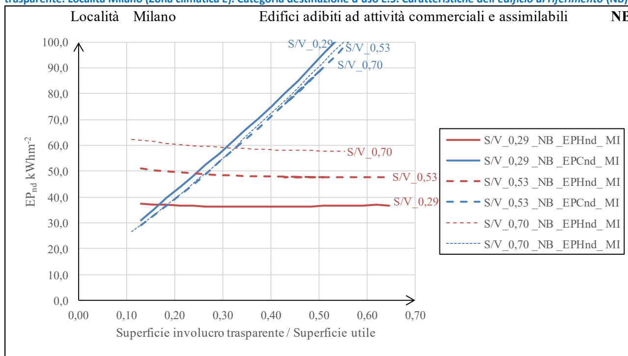
Figura 39 – Prestazioni energetiche degli edifici analizzati al variare del rapporto di forma S/V_L e della superficie dell'involucro trasparente. Località Milano (Zona climatica E). Categoria destinazione d'uso E.5. Caratteristiche dell'edificio di riferimento (NB).
