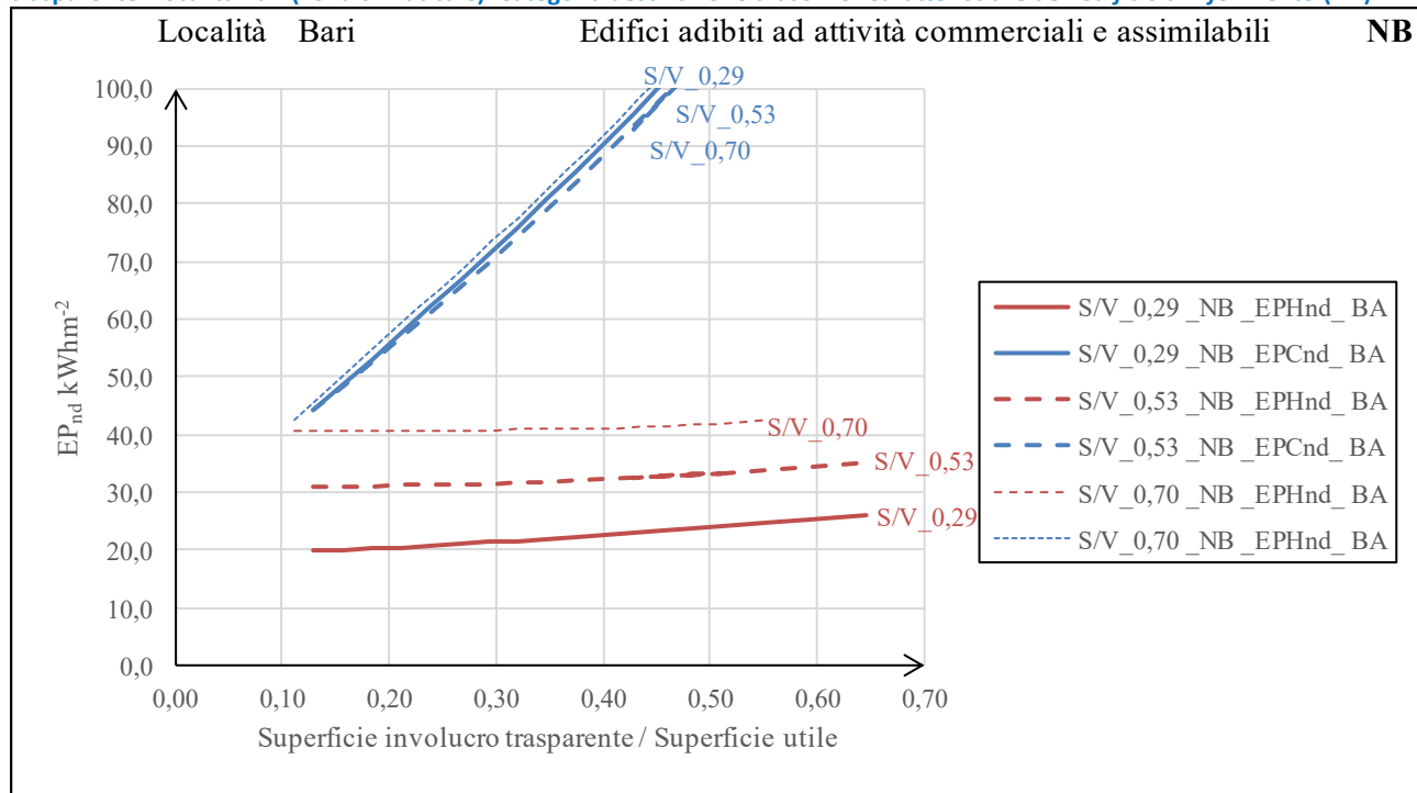
Figura 33 – Prestazioni energetiche degli edifici analizzati al variare del rapporto di forma S/V_L e della superficie dell'involucro trasparente. Località Bari (Zona climatica C). Categoria destinazione d'uso E.5. Caratteristiche dell'edificio di riferimento (NB).
