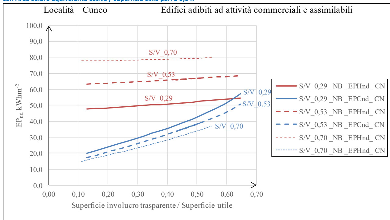
Figura 42 – Prestazioni energetiche degli edifici analizzati al variare del rapporto di forma S/V_L e della superficie dell'involucro trasparente. Località Cuneo (Zona climatica F). Categoria destinazione d'uso E.5. Caratteristiche dell'edificio di riferimento (NB*) con Area solare equivalente estiva / superficie utile pari a 0,04.
