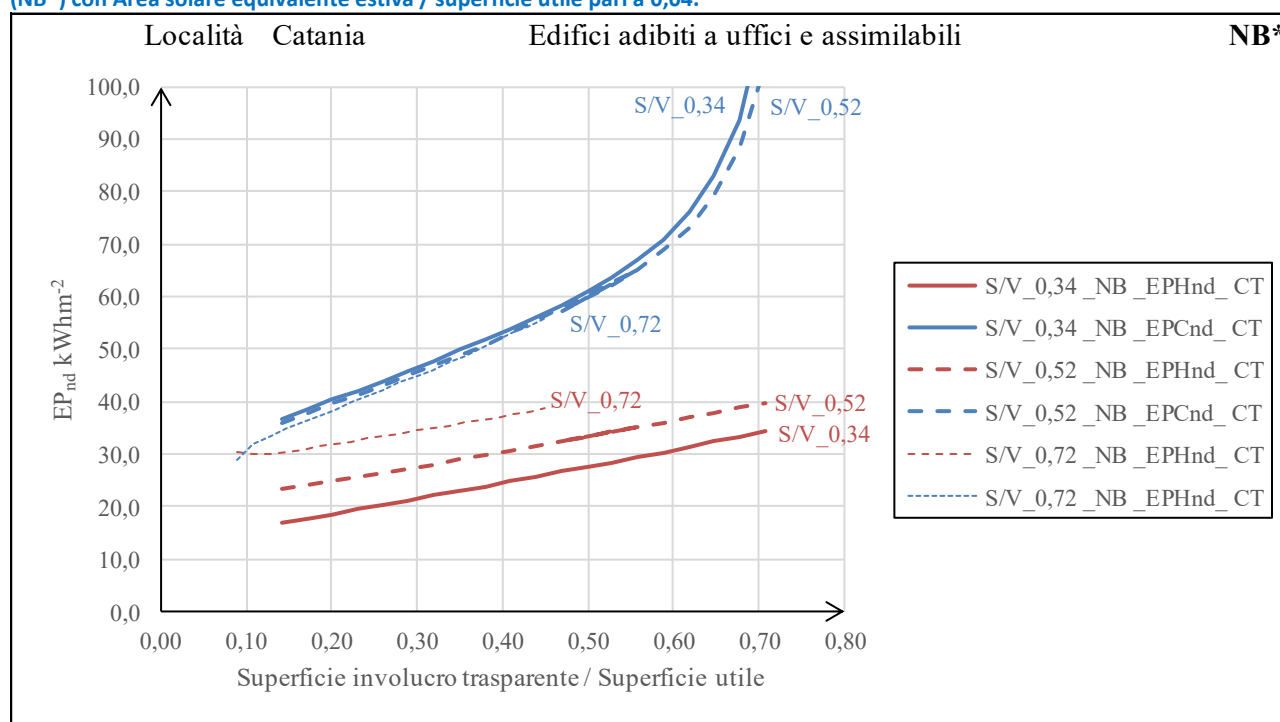
Figura 18 – Prestazioni energetiche degli edifici analizzati al variare del rapporto di forma S/V_L e della superficie dell'involucro trasparente. Località Catania (Zona climatica B). Categoria destinazione d'uso E.2. Caratteristiche dell'edificio di riferimento (NB*) con Area solare equivalente estiva / superficie utile pari a 0,04.
