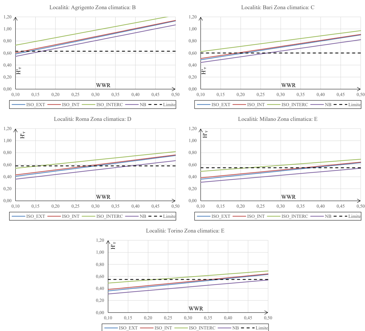
Figura 123 –Correlazione tra WWR e parametro H'_T
