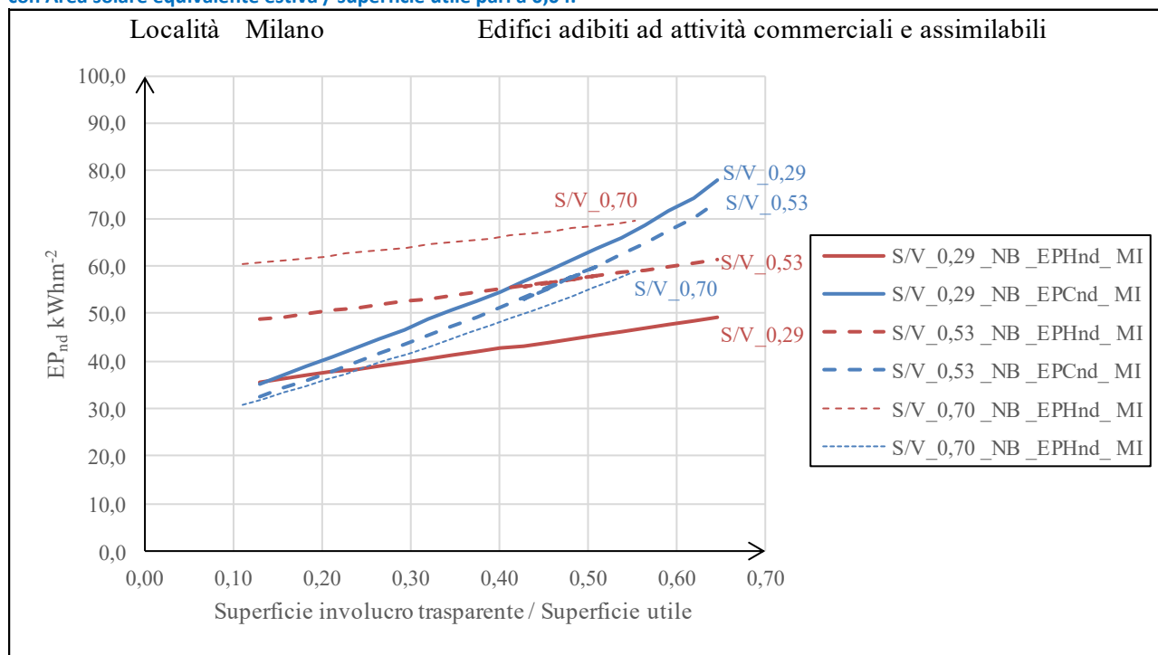
Figura 38 – Prestazioni energetiche degli edifici analizzati al variare del rapporto di forma S/V_L e della superficie dell'involucro trasparente. Località Milano (Zona climatica E). Categoria destinazione d'uso E.5. Caratteristiche dell'edificio di riferimento (NB*) con Area solare equivalente estiva / superficie utile pari a 0,04.
