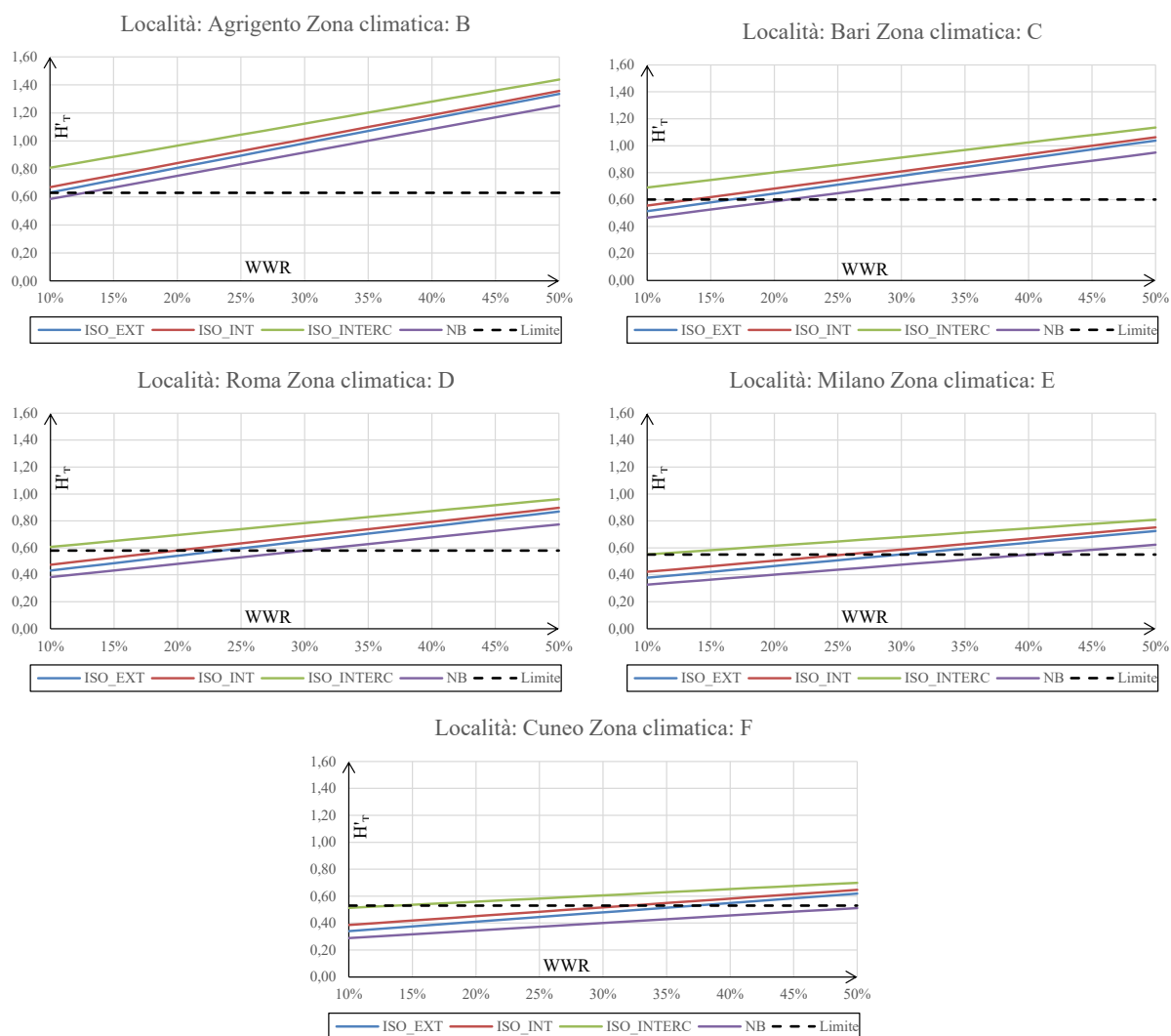
Figura 227 – Edificio ad uso uffici, Rapporto di forma 0,40 < S/V < 0,70 . Correlazione tra WWR e parametro H'_T
