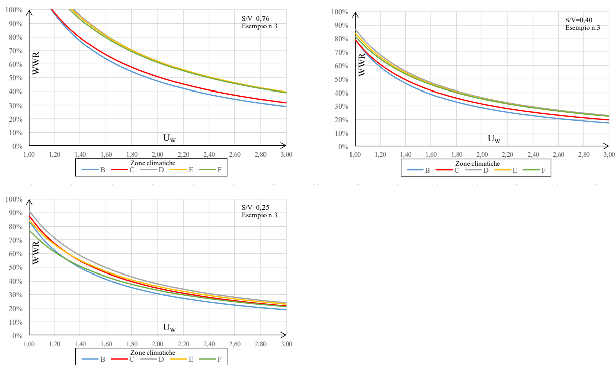
Figura 403 – Caso studio “Esempio n.3” Variazione della superficie trasparente massima realizzabile per un edificio con diverso rapporto di forma S/V=0,76 (primo), S/V=0,40 (secondo) e S/V=0,25 (terzo)
