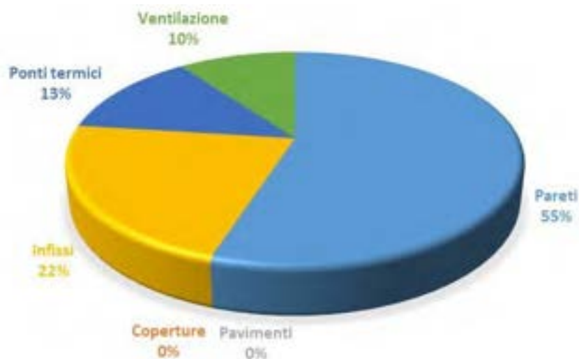
Figura 31. Incidenza delle voci di dispersione sulla potenza termica invernale – unità U1 del piano tipo
