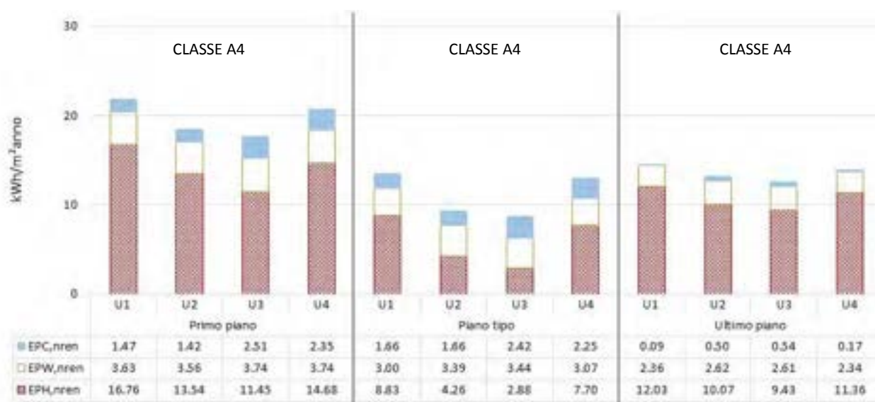
Figura 72. Fabbisogni specifici di energia primaria non rinnovabile
