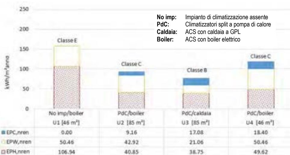
Figura 33. Fabbisogno di energia primaria non rinnovabile – primo piano
