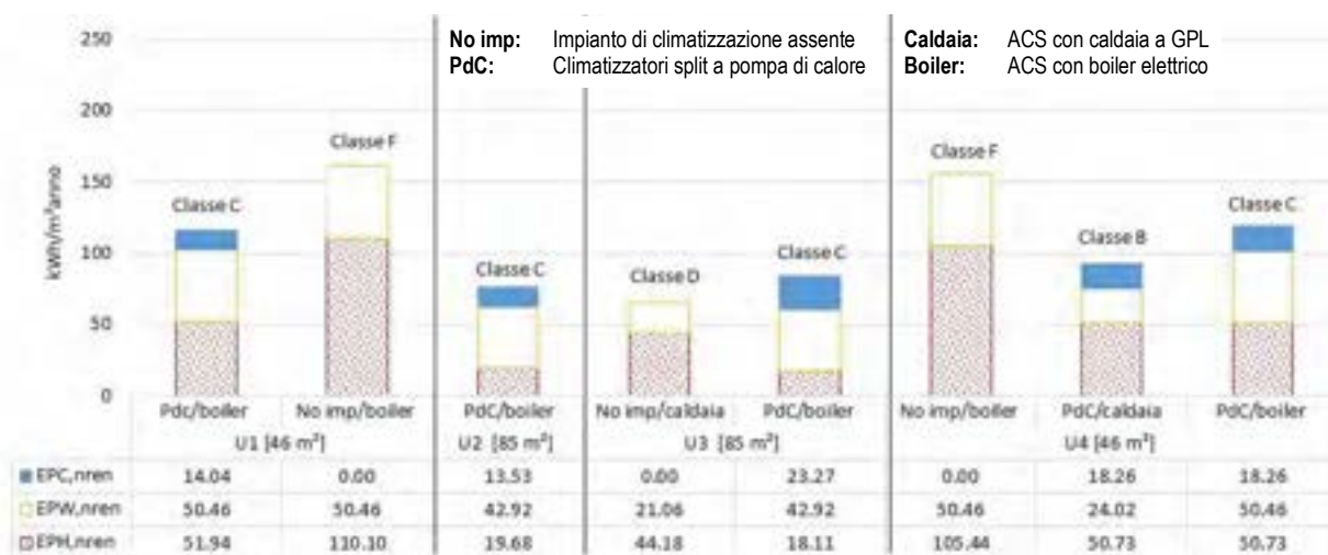
Figura 34. Fabbisogno di energia primaria non rinnovabile – piano tipo
