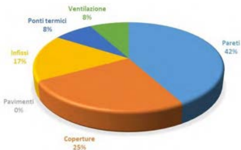
Figura 32. Incidenza delle voci di dispersione sulla potenza termica invernale – unità U1 dell'ultimo piano
