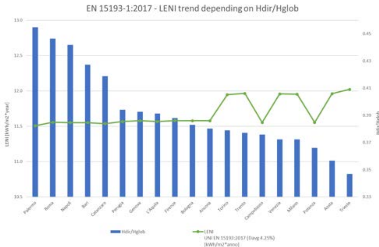
Figura 13 Andamento del LENI al variare del rapporto H_{dir}/H_{glob}
