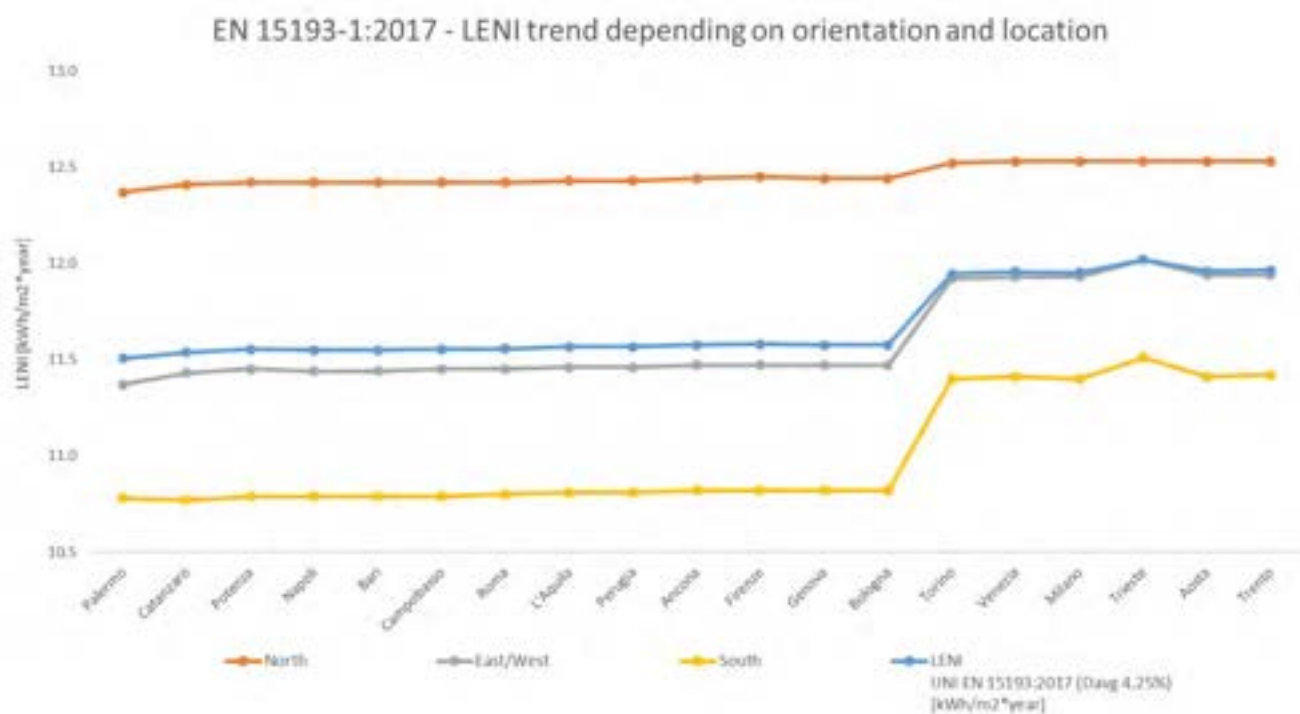
Figura 12 Valori del LENI al variare dell'orientamento e della località ("Metodo 1" della UNI EN 5193:2017)
