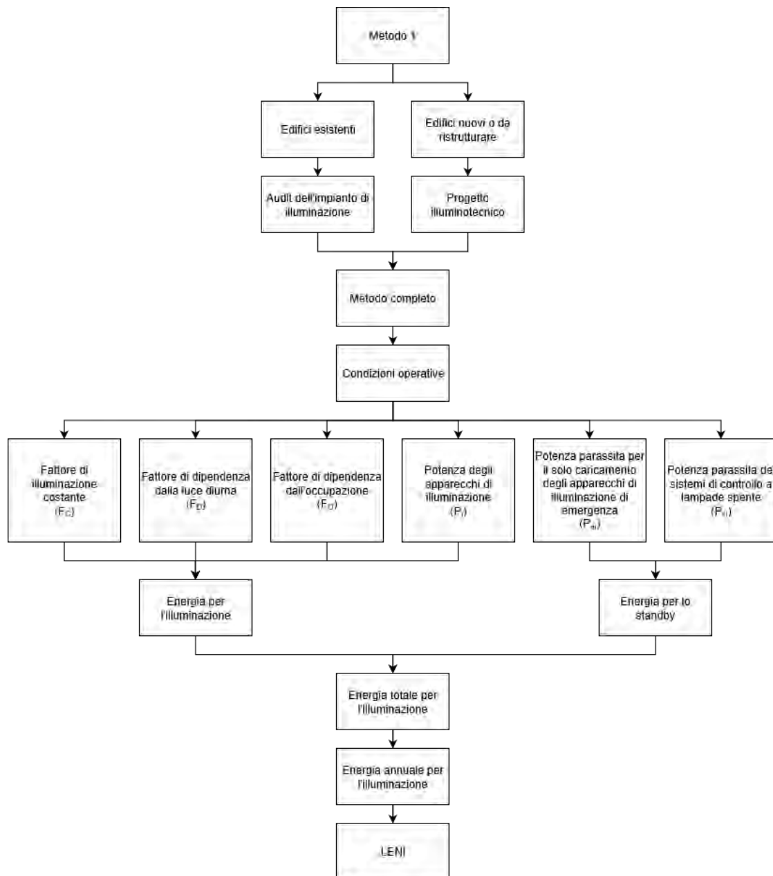
Figura 1 Schema a blocchi del “Metodo 1” della UNI EN 15193-1:2017 per il calcolo del LENI
