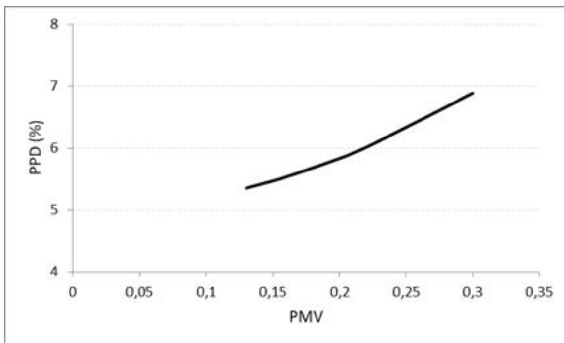
Figura 4.8.8. Andamento dell'indice PPD in funzione del PMV – 18/05/2018.
