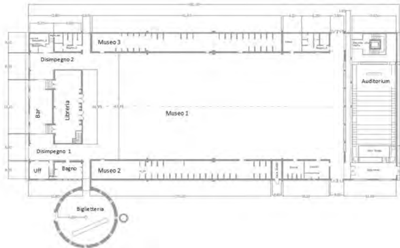
Figura 5.1.1. Planimetria museo del carbone
