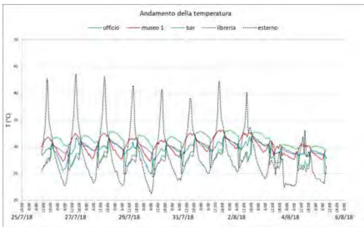
Figura 5.5.2. Profilo di temperatura all'esterno e all'interno degli ambienti del museo del carbone 27/7/18 – 05/8/18.
