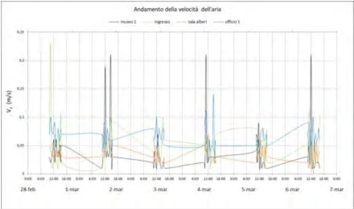
Figura 4.2.8. Andamento della velocità nei locali del museo dei Paleo Ambienti Sulcitani – 01/3/18 – 06/3/18.
