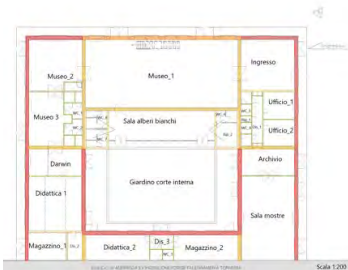
Figura 4.1.1. Planimetria piano terra - museo Paleo Ambienti Sulcitani.
