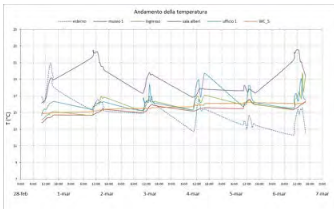
Figura 4.2.6. Profilo di temperatura all'esterno e all'interno degli ambienti del museo PAS – 01/3/18 – 6/3/18.
