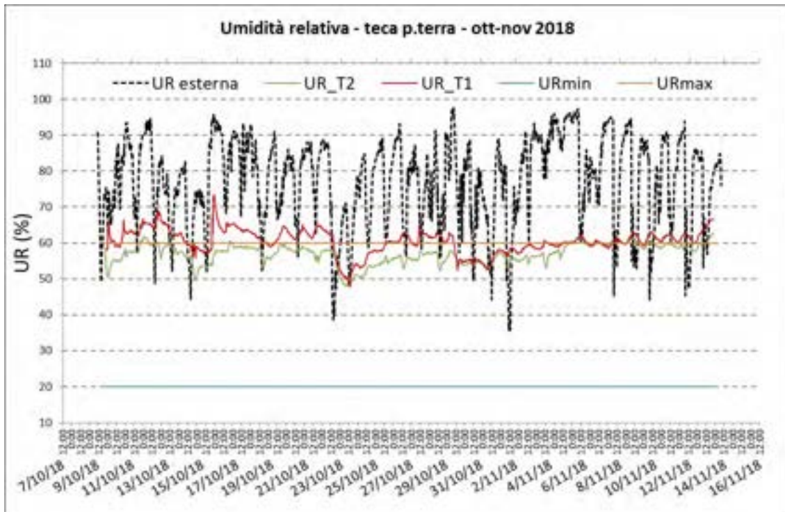
Figura 3.18. Andamento dell'umidità relativa al piano terra (UR_T2) e all'interno della teca (UR_T1) – 9 ott – 8 nov 2018.
