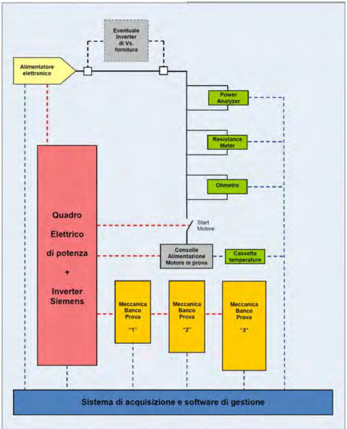
Figura 3: Schema funzionale della facility
