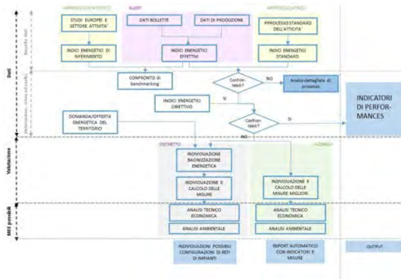
Figura 3 – Flow chart dell'approccio sistemico proposto SPAS
