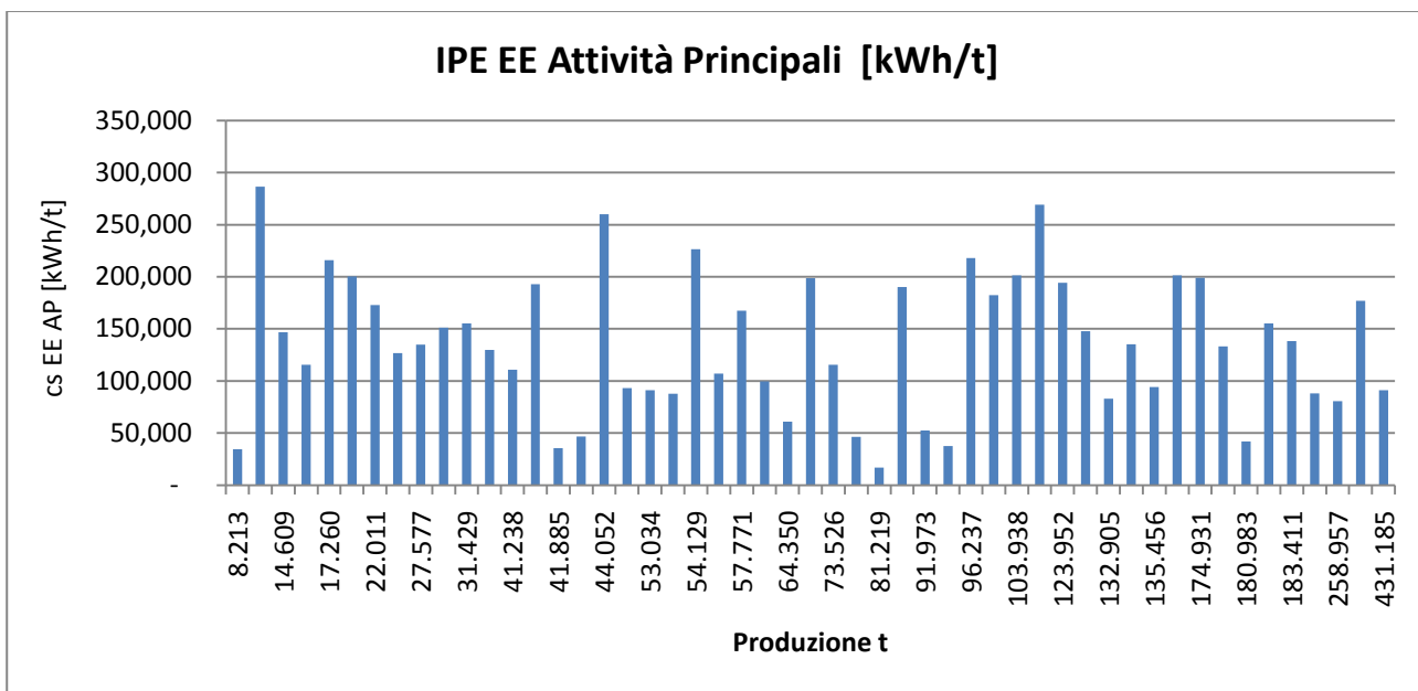
Figura 36 Settore ceramico: IPE energia elettrica attività principali
