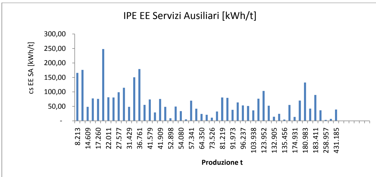
Figura 37 Settore ceramico: IPE energia elettrica servizi ausiliari
