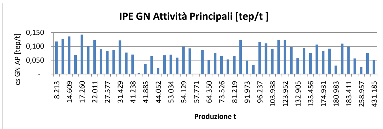
Figura 38 Settore ceramico: IPE gas naturale attività principali
