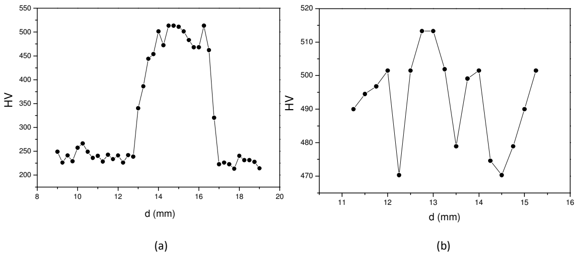
Fig. 26- Cordone di saldatura su acciaio S460 (campione 1): profili di microdurezza Vickers attraverso il cordone (a) e verticalmente lungo l'asse centrale.
