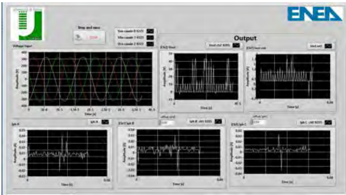
Fig. 13- Pannello del software di supervisione realizzato in LabVIEW
