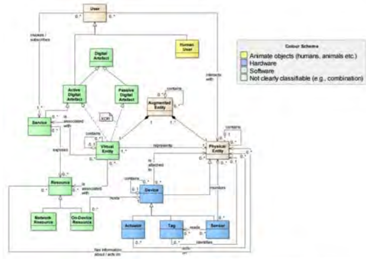
Figura 6 Architettura IoT-A.
