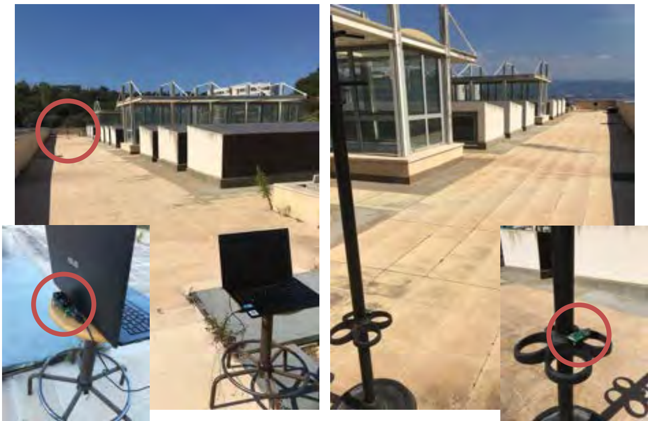
Figura 18 Scenario di propagazione outdoor relativo alle misure di Tabella 7.
