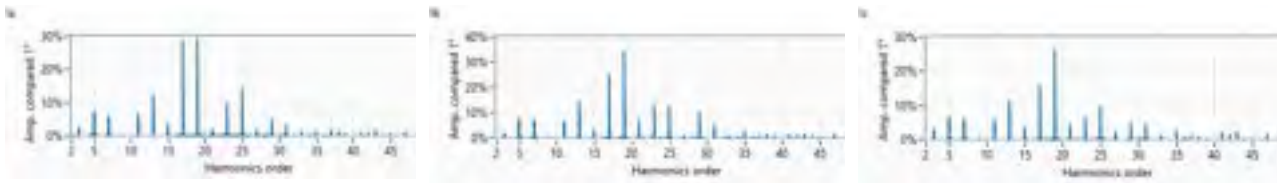
Figura 73 - Analisi del contenuto armonico delle correnti
