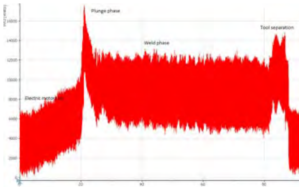
Figura 71 - Andamento della potenza assorbita durante il processo di saldatura totale
