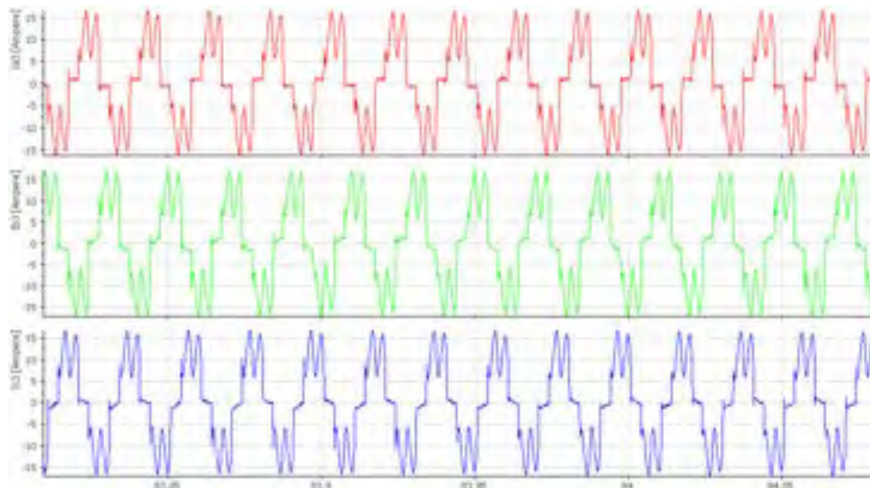
Figura 15 – Dettaglio delle correnti sul primario
