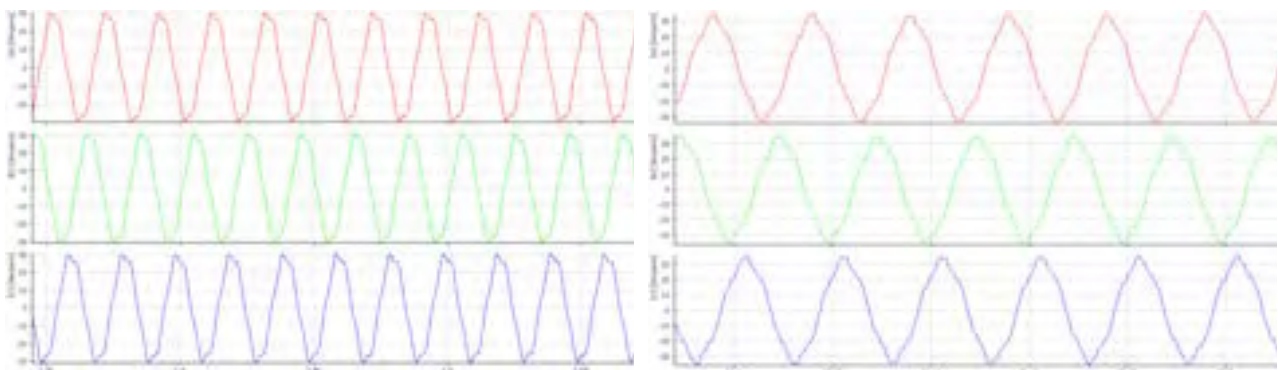
Figura 64 - Forme d'onda corrente trifase nelle 2 fasi di saldatura
