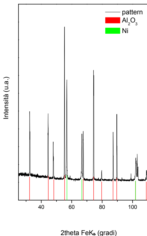
Figura 13. Spettro di diffrazione eseguito su campioni impregnati da soluzioni di formiati. In questo esempio il substrato di allumina è stato impregnato con formiato di nichel e successivamente trattato in atmosfera inerte per evitare la formazione di carburi osservabile quando il campione è trattato in atmosfera riducente.
