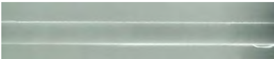
Fig. 5 Radiografia giunto saldato
