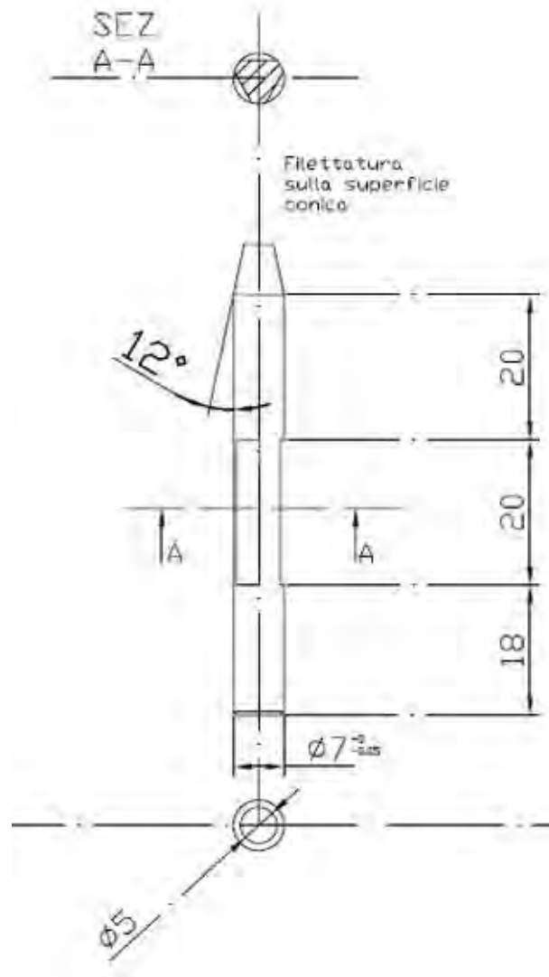
Fig. 3 Punta dell'utensile
