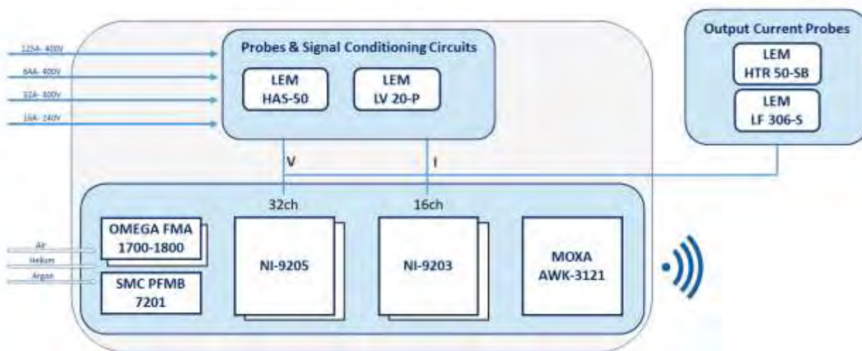
Figura 18. Schema a blocchi del sistema di misura
