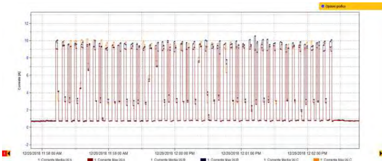
Figura 15. Clinchiatura: Correnti in ingresso alla macchina
