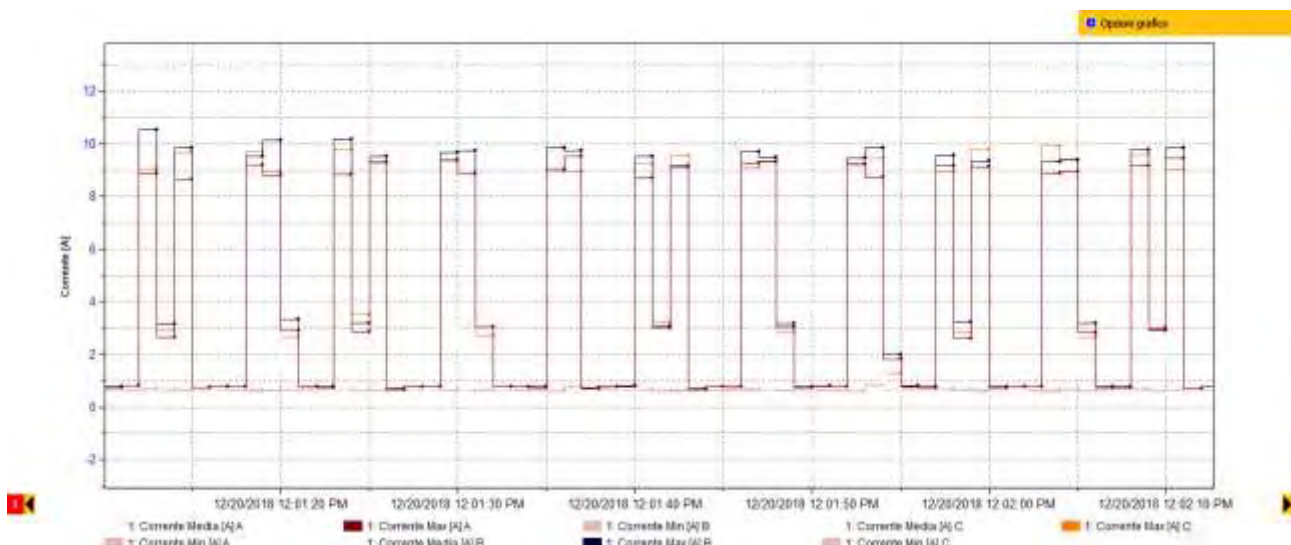
Figura 16. Clinchiatura: Dettaglio delle correnti in ingresso alla macchina
