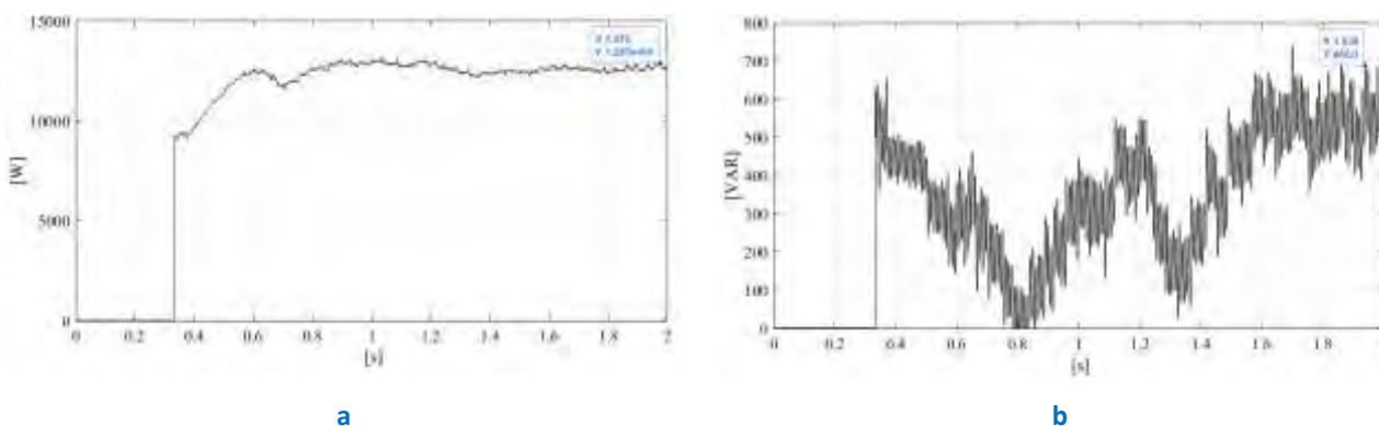
Figura 7. Misura della potenza attiva e reattiva nel corso della prova
