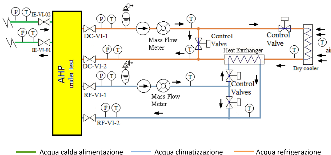
Figura 9 – Schema semplificato implementazione AHP
