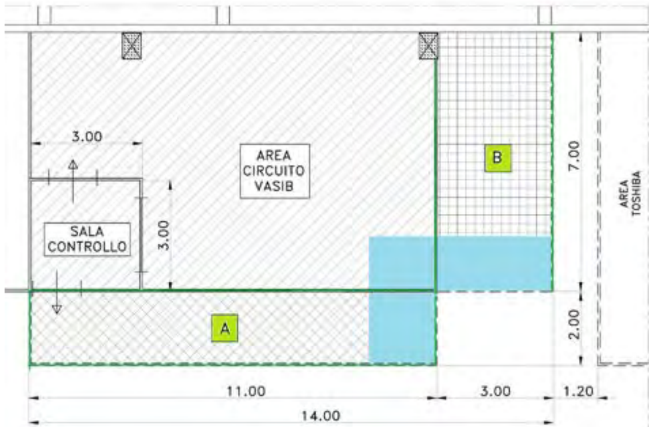
Figura 13b – Impianto VASIB attuale e aree disponibili per l'ampliamento a impianto CERCO
