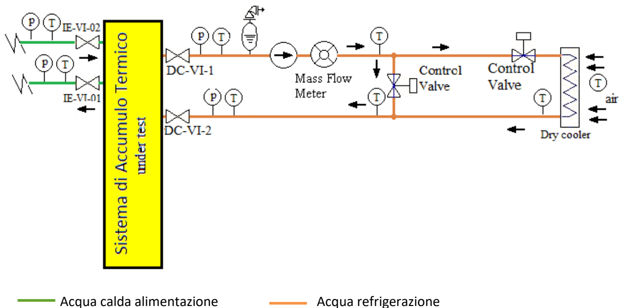
Figura 11 – Schema semplificato implementazione SAT
