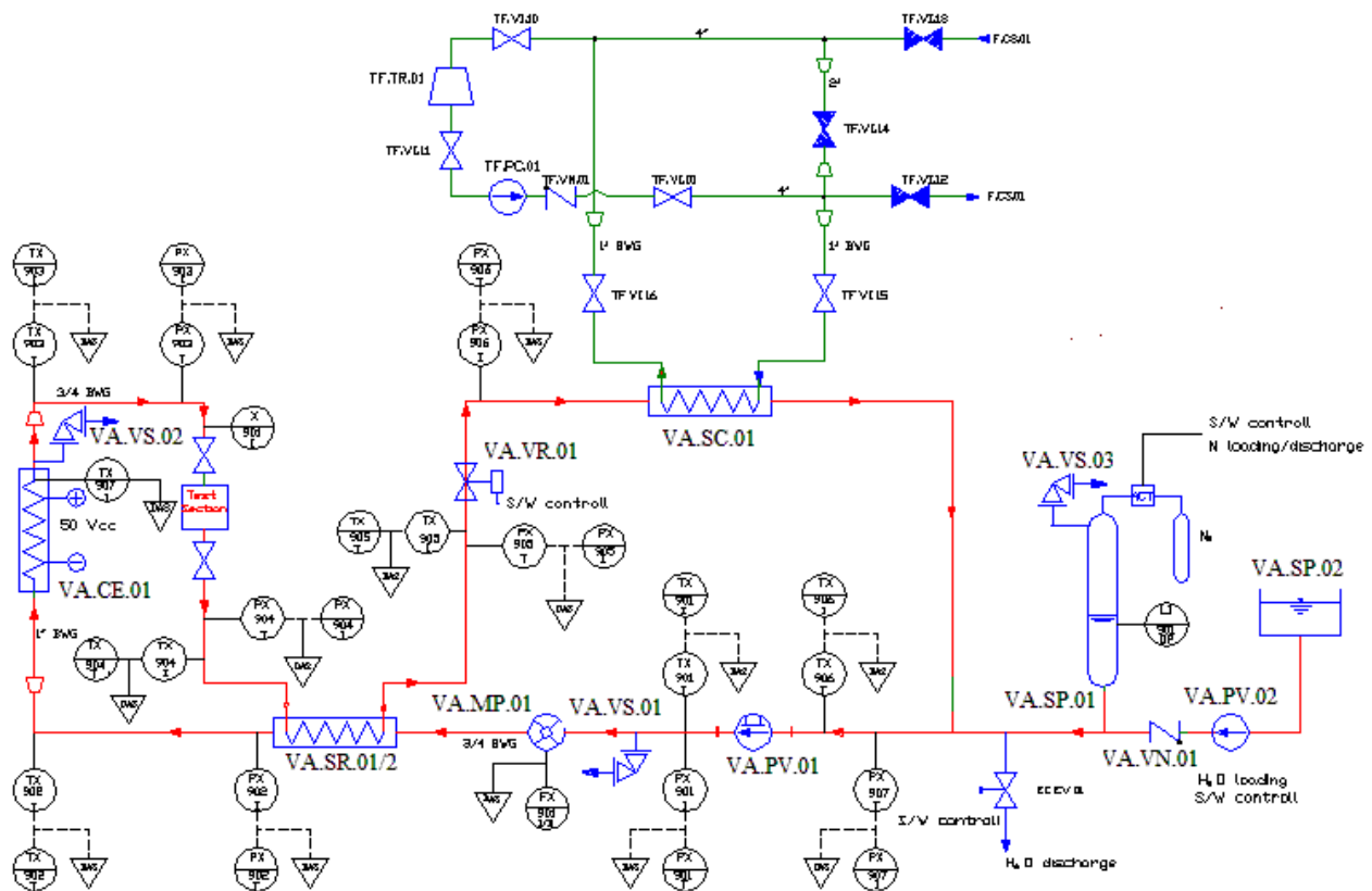
Figura 2 - Schema impianto VASIB
