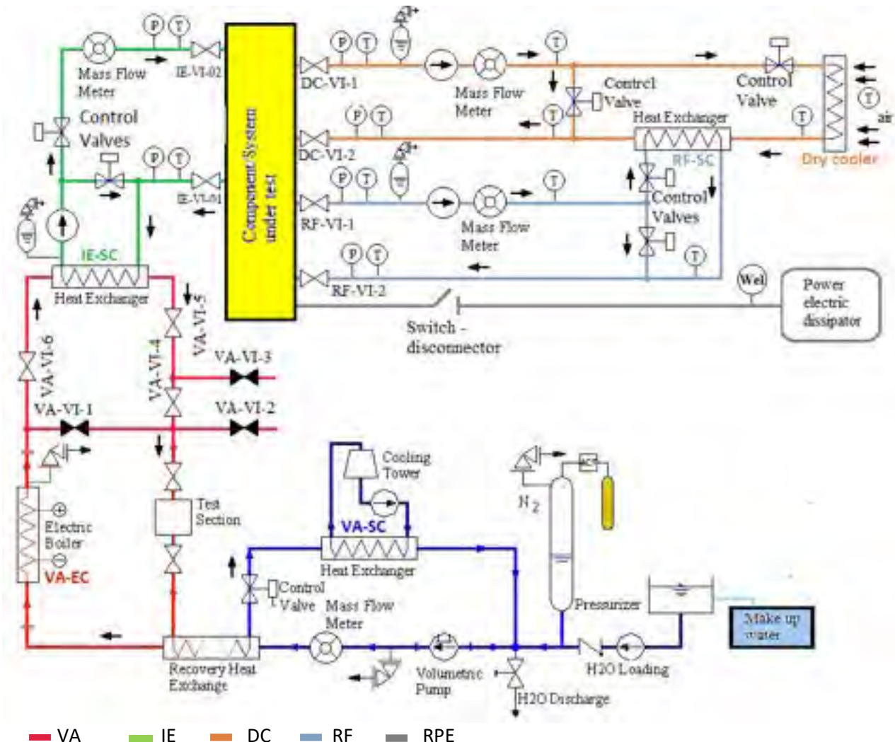
Figura 12 – Schema semplificato impianto CERCO
