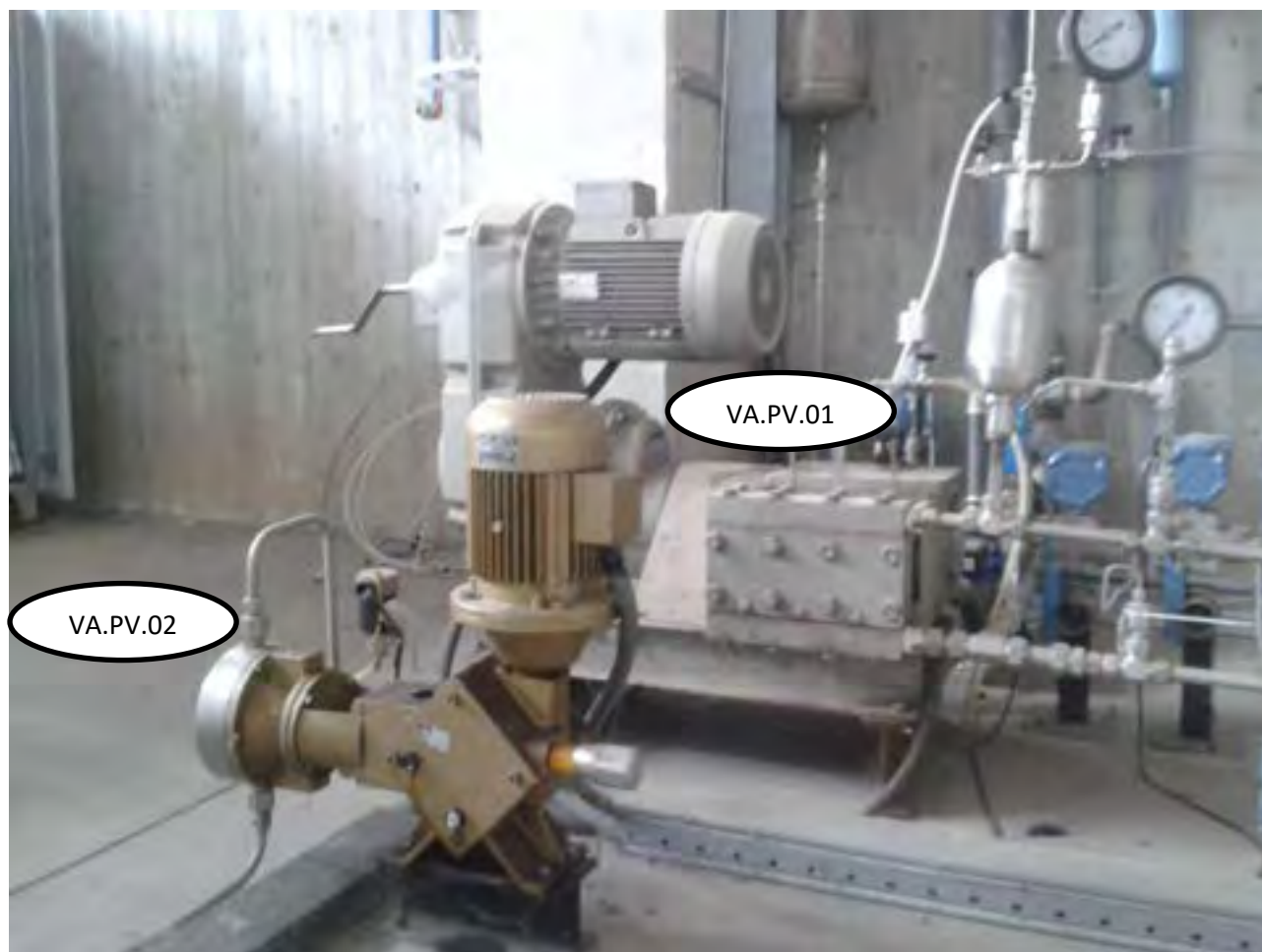
Figura 4 –pompa di carico acqua e pompa di circolazione
