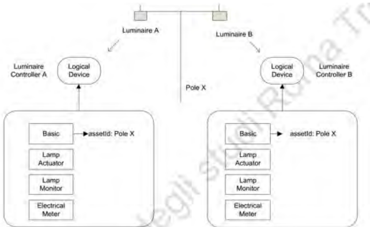
Figura 22 – Esempio pratico di due dispositivi logici assegnati allo stesso asset fisico.
