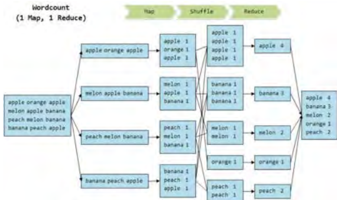
Figura 2 – Conteggio di parole in un file con MapReduce
