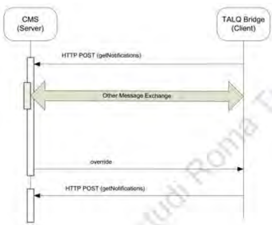
Figura 20 – Rappresentazione schematica di una tipica comunicazione HTTP long polling.
