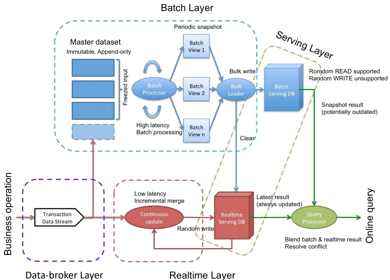
Figura 7 – l'architettura lambda per l'analisi dei big data.
