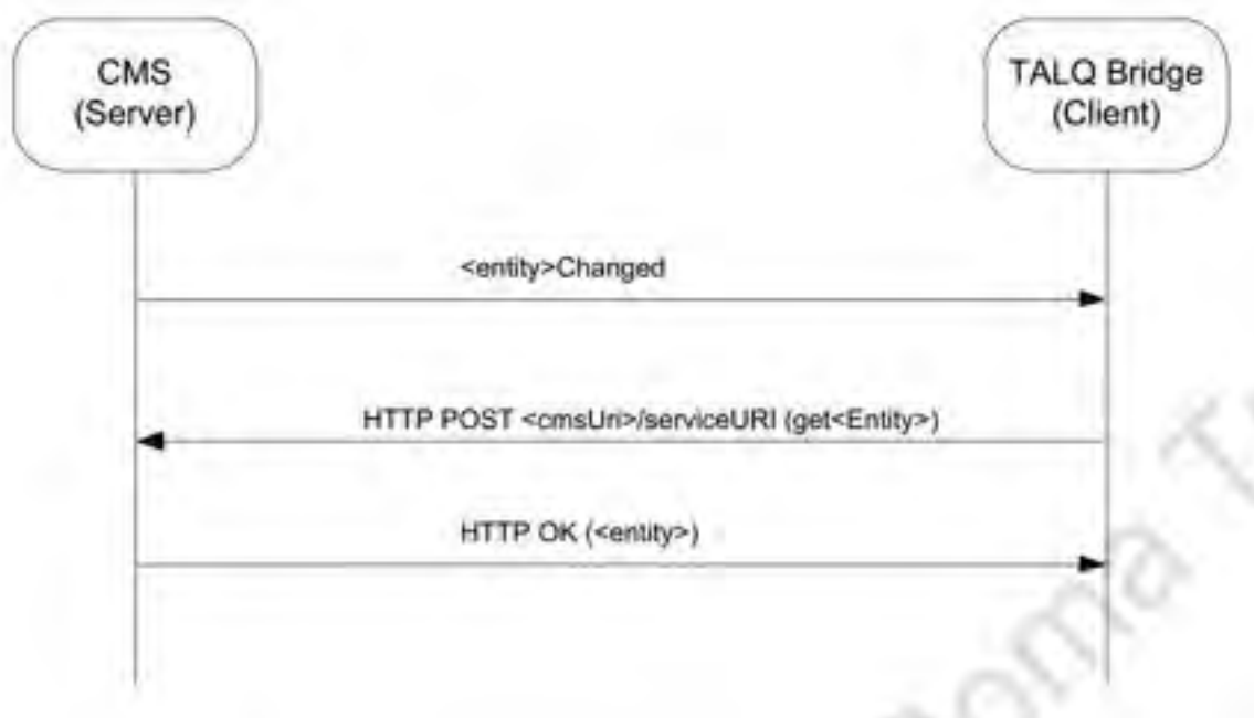
Figura 23 – Comunicazione tra TALQ Bridge e CMS per gestire una entità appartenente al CMS. Il CMS comunica l'avvenuta modifica di una entità, il TALQ Bridge risponde richiedendo la descrizione delle modifiche, il CMS conclude la comunicazione trasmettendo lo stato attuale dell'entità.
