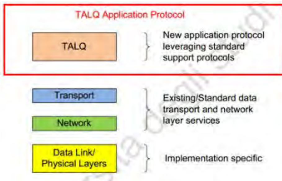
Figura 18 – Inquadramento del protocollo TALQ all’interno di uno stack ISO/OSI
