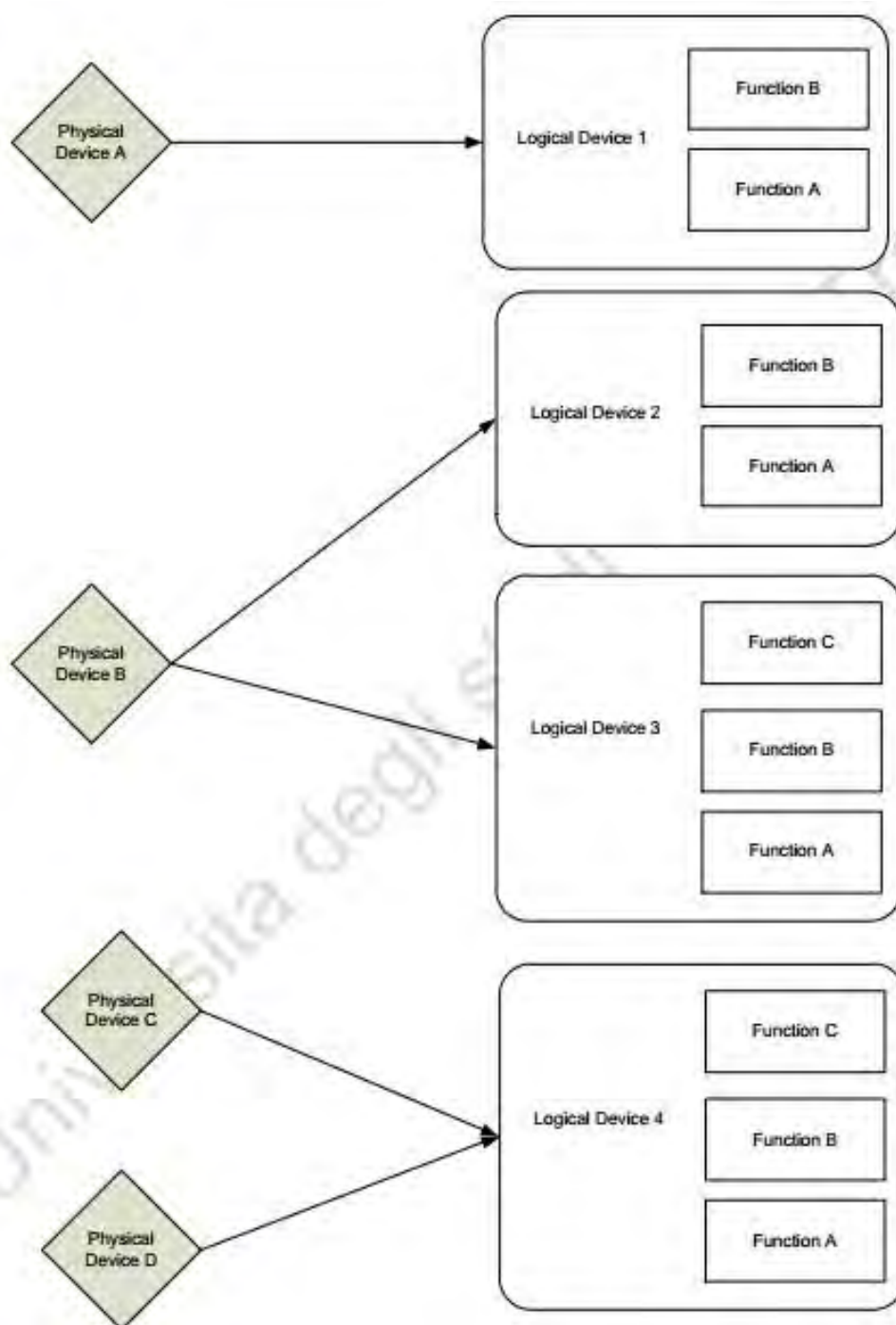
Figura 21 – Gerarchia dei dispositivi fisici, logici e delle funzioni.
