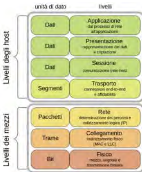
Figura 9 Modello ISO/OSI
