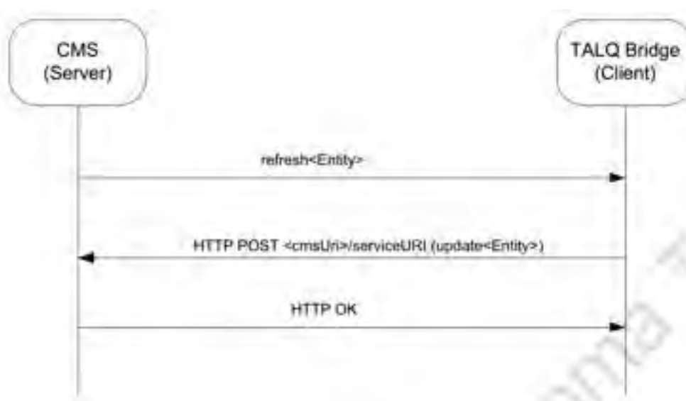
Figura 24 – Comunicazione tra TALQ Bridge e CMS per gestire una entità appartenente al TALQ Bridge. Il CMS richiede un aggiornamento dello stato della entità, il TALQ Bridge risponde con l'aggiornamento (totale o parziale), ad avvenuta ricezione il CMS conclude la comunicazione con HTTP OK.
