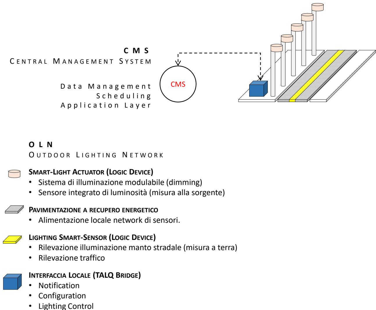
Figura 25 – Caso di studio per illuminazione smart del manto stradale.
