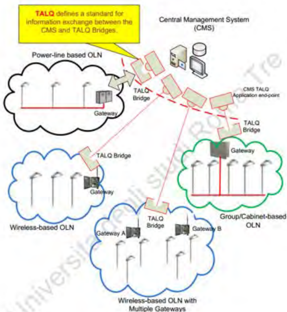
Figura 17 – Paradigma di controllo di un sistema basato su architettura TALQ.
