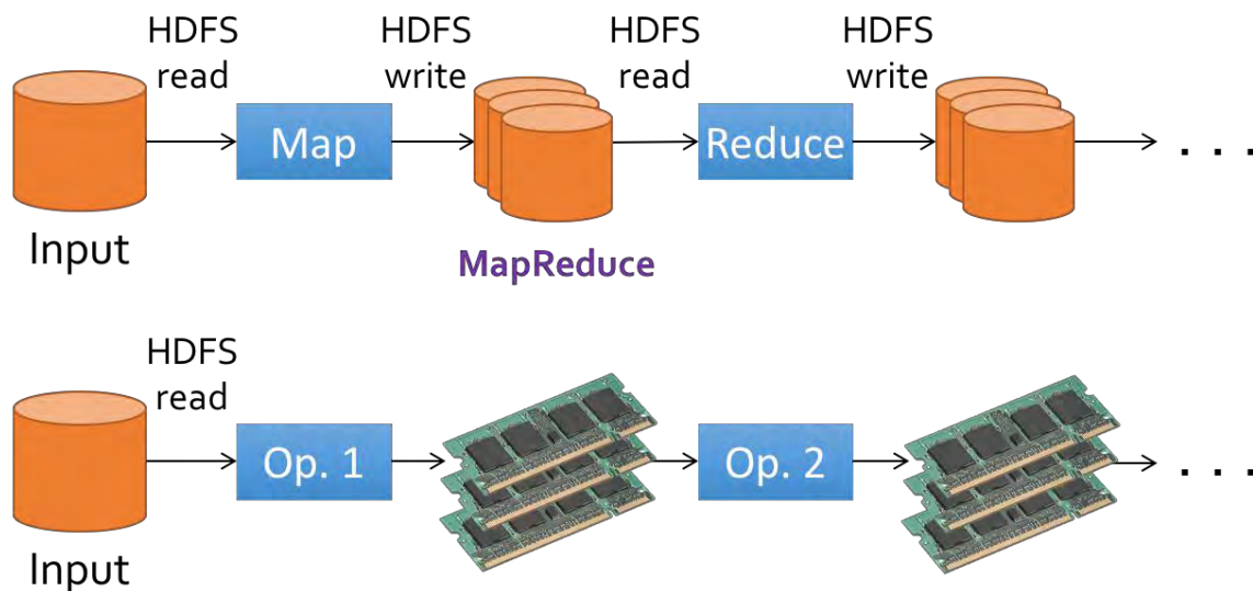
Figura 3 – Elaborazione MapReduce e Spark a confronto
