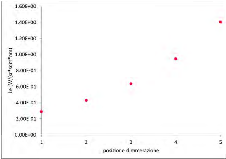
Figura 52 - Radianza in funzione della dimmerazione
