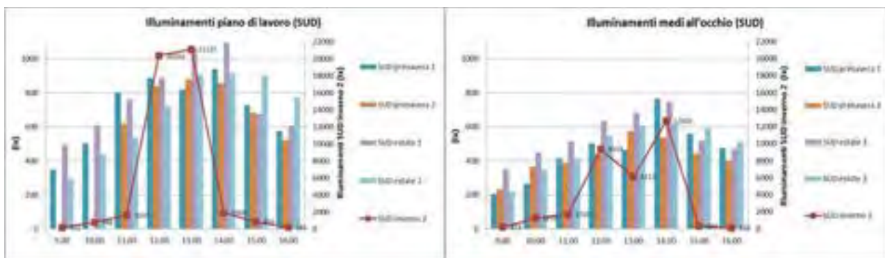
Figura 55 - Valori di illuminamento interno all'occhio e sul piano di lavoro a confronto per le due esposizioni NORD e SUD
