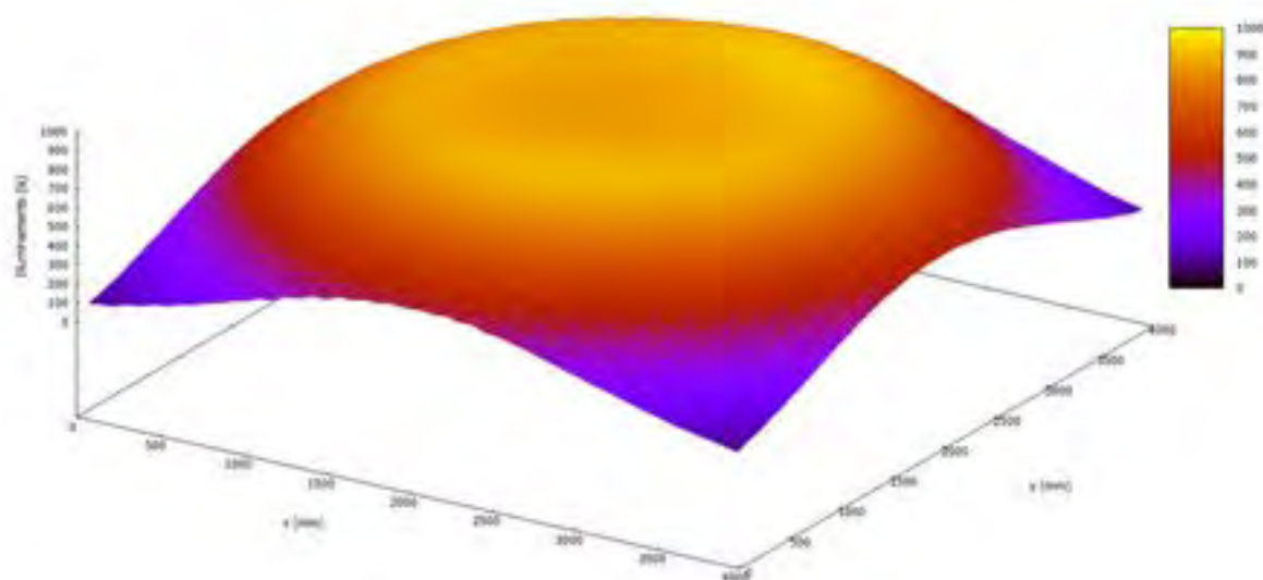
Figura 28 - Mappa illuminamento HumbleBee a 2.60 m con riflettore installato in posizione erronea
