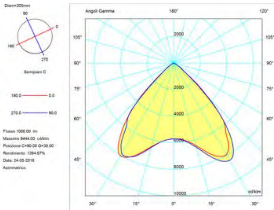
Figura 29 - Solido HumbleBee con riflettore installato in posizione errnea
