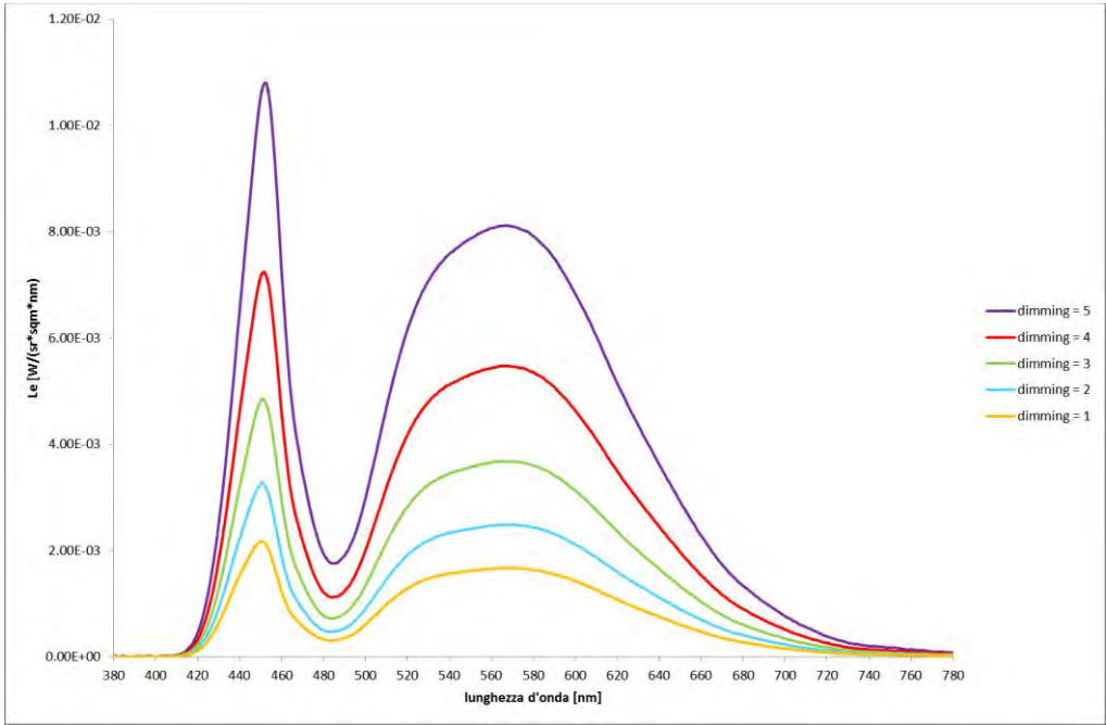
Figura 51 - Radianza spettrale
