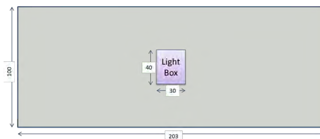
Figura 42 - Rettangolo di misura illuminanti a 50 cm (misure in cm)
