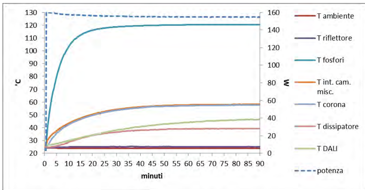
Figura 33 - Misure termiche HumbleBee a 25°C ambiente, dimmerazione 100%
