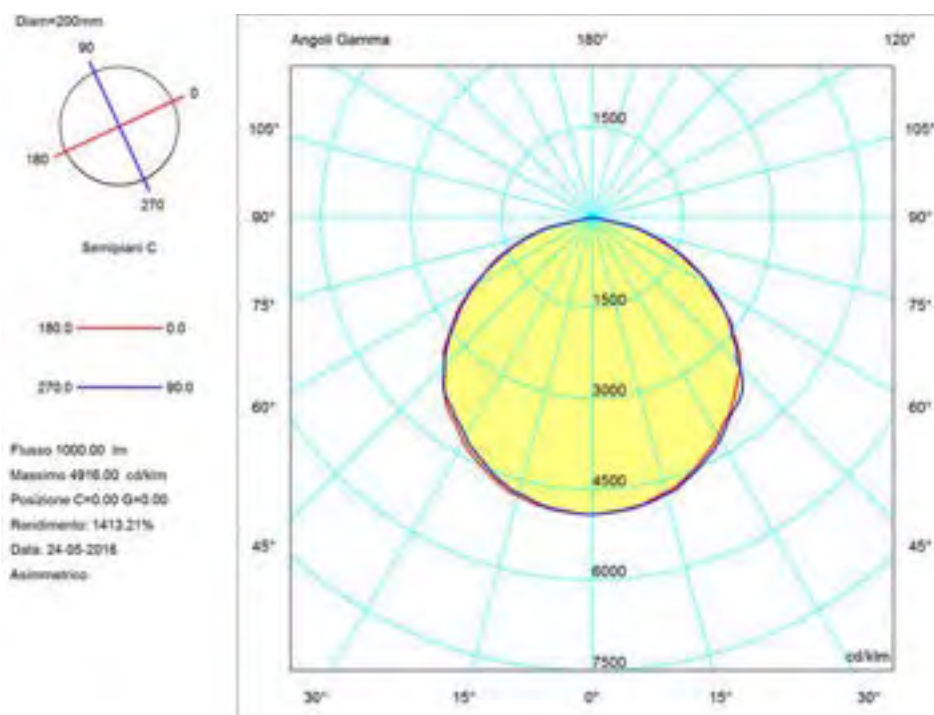
Figura 27 - Solido fotometrico HumbleBee senza riflettore
