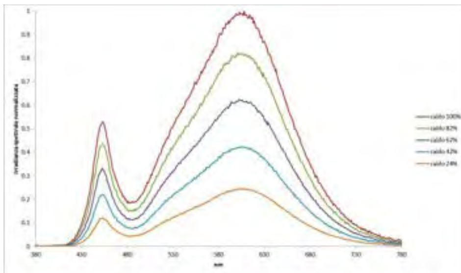
Figura 14- Irradianza spettrale normalizzata sul tavolo, in dimmerazione, tonalità calda
