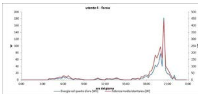
Figura 61 - utilizzo forno elettrico caso d'uso 2 - utente 4
