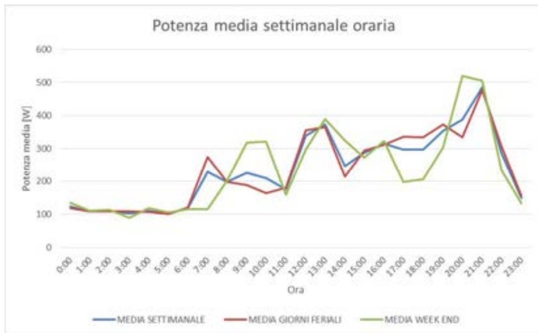
Figura 33 Profilo settimanale di utilizzo dell'energia elettrica
