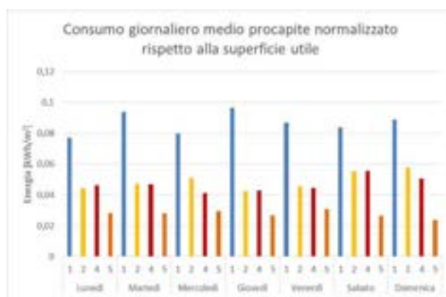
Figura 32- Consumo medio giornaliero per m² di abitazione in 4 casi pilota.
