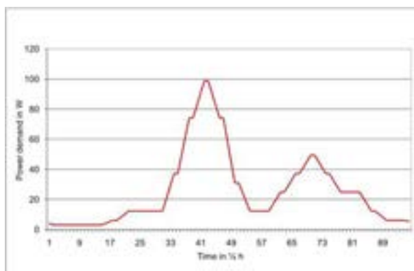
Figura 60 - Curva carico forno in Europa
