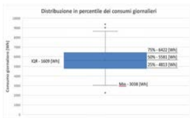
Figura 28 Distribuzione in frequenza attraverso rappresentazione box plot dei consumi dell'edificio pilota n.1
