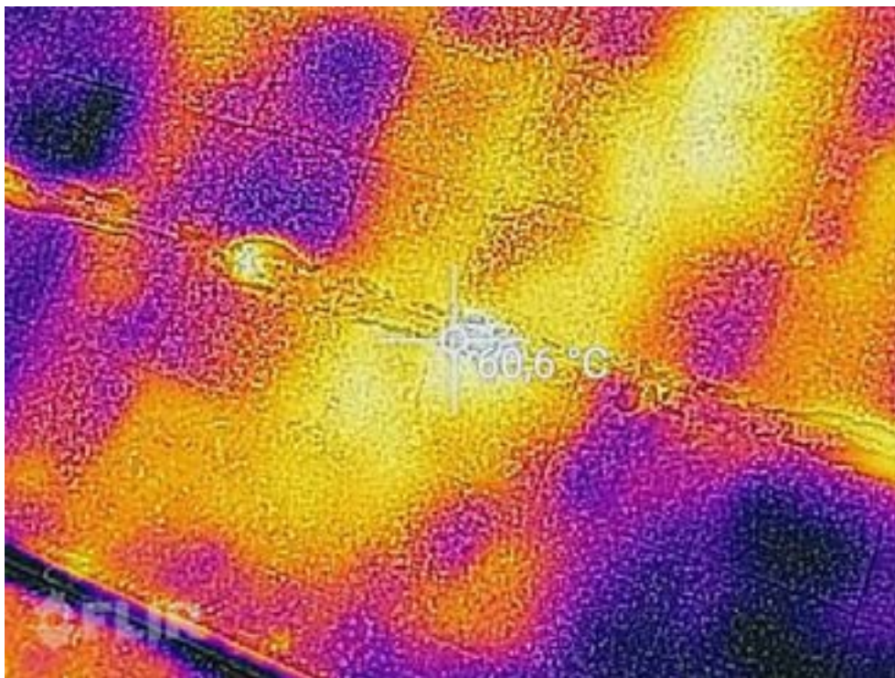
Fig.3.2.8 – Temperatura sulla parte di tetto sporco, 10° in più rispetto alla parte pulita
